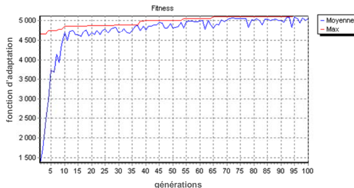
Figure 92 : Evolution de la population (moyenne et maximum de la fonction d'adaptation)
