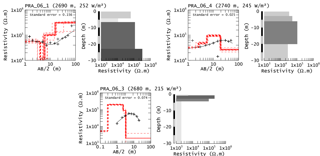
Figure VII-21 : Sondages électriques verticaux réalisés en 2006 dans le vallon de Pradiou, et leur interprétation (voir fig. VII-20 pour la localisation). Vertical electrical soundings performed in the Vallon de Pradiou in 2006, and their interpretation (see fig. VII-20 for location).
