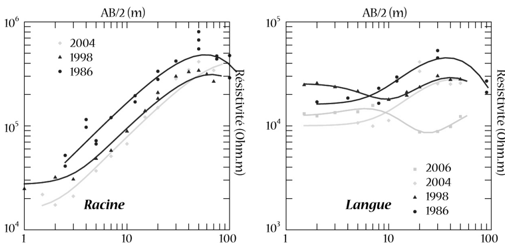
Figure VIII-15 : Comparaison des courbes des sondages électriques verticaux effectués à la racine et sur la langue de RGL1, en 1986, 1998, 2004 et 2006. Comparison between geoelectrical soundings performed on the root and on the tongue of RGL1 in 1986, 1998, 2004 and 2006.
