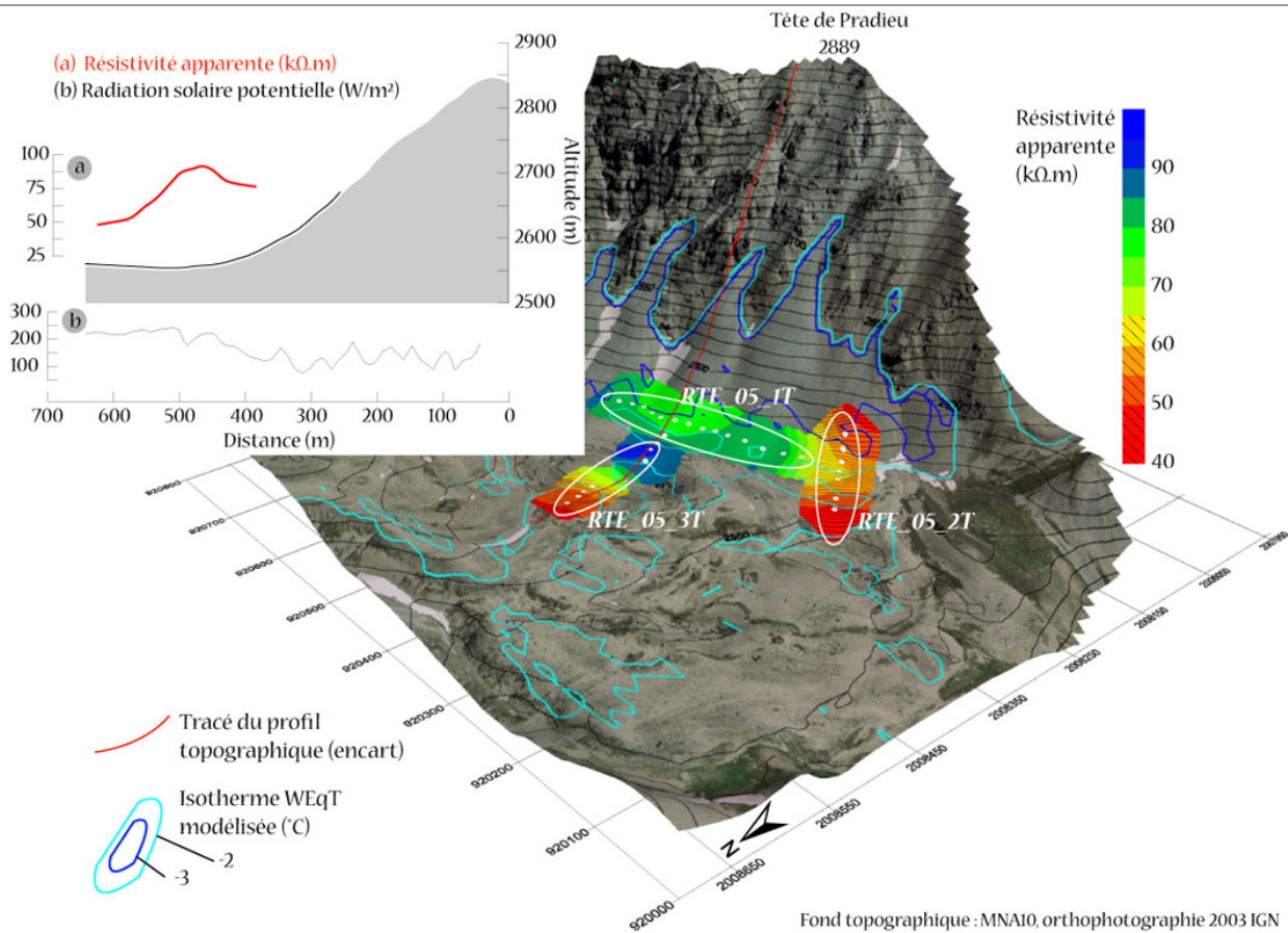
Figure VII-18 : Cartographie 3D des résistivités apparentes relevées par la méthode du traîné électrique sur trois profils du vallon de la Route (écartement inter-électrodes : 15 m, épaisseur prospectée : 8-10 m), et des WEqT (Winter Equilibrium Temperatures) modélisées (cf. chap. VI, § 3). Resistivity values measured by the "trainé" technique on the Vallon de la Route, and modelled WEqT.
