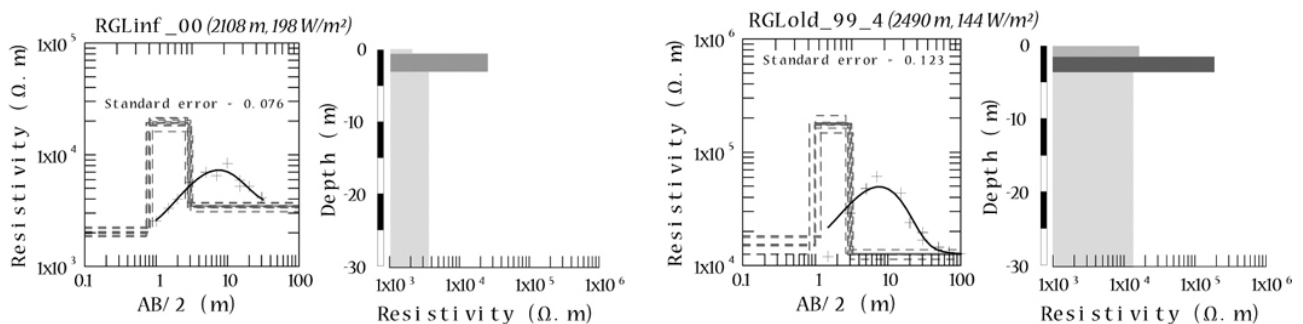
Figure VII-8 : Interprétation des sondages effectués sur des formes reliques de la combe de Laurichard (données brutes non publiées de V. Jomelli et D. Fabre) : à gauche, à 2108 m d'altitude, à proximité du col du Lautaret ; à droite, à 2490 m, au débouché du grand cône d'avalanche de l'ubac. Interpretation of the geoelectrical soundings performed on two relict landforms in the Combe de Laurichard.
