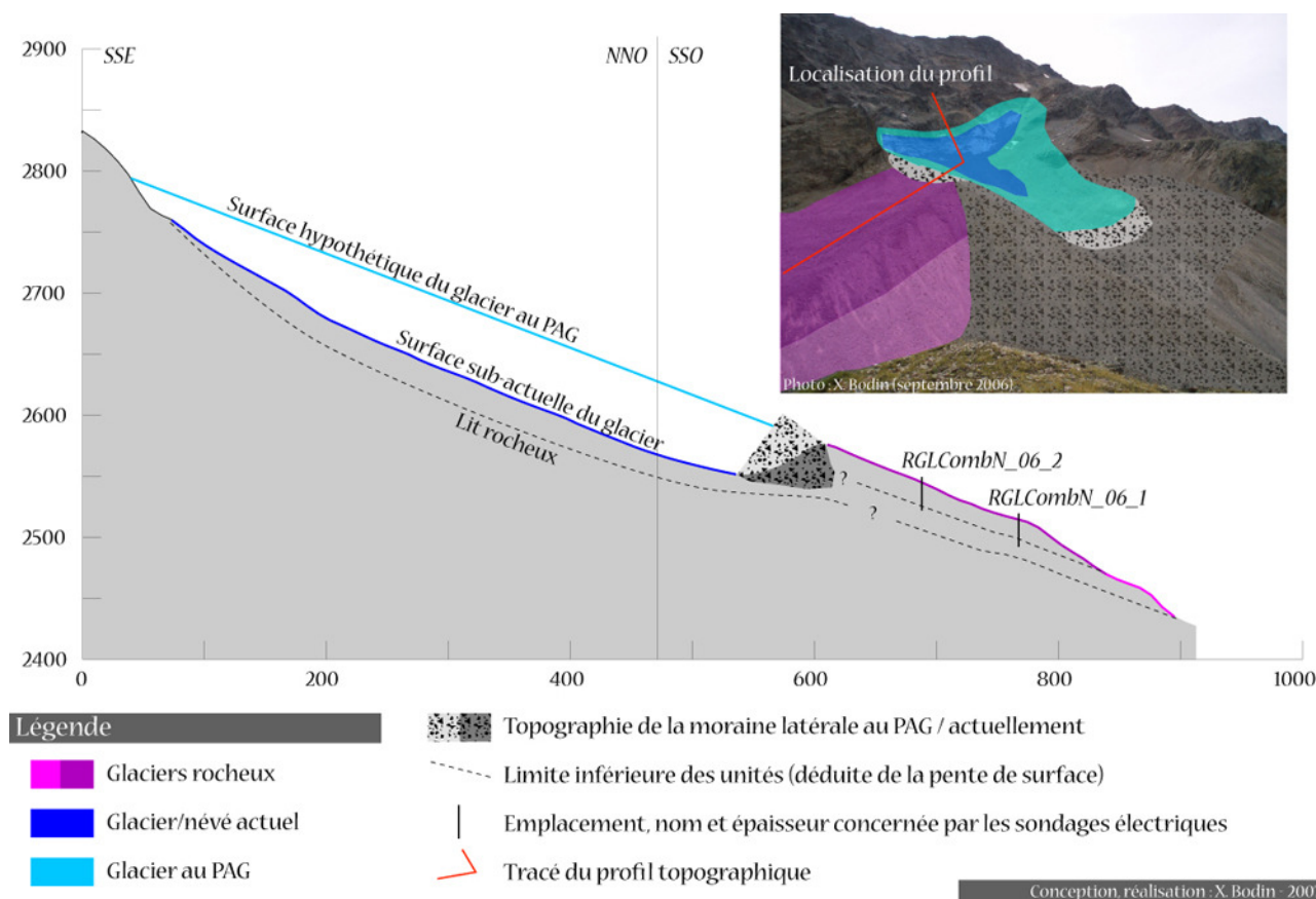
Figure VII-3 : Profil topographique du complexe glacier/moraine/glaciers rocheux du vallon du Combeynot Nord et interprétation géomorphologique déduite des sondages verticaux. Topographic cross-section (grey) and geomorphological interpretation of the glacier/moraine/rockglacier complex of the Combeynot N valley.
