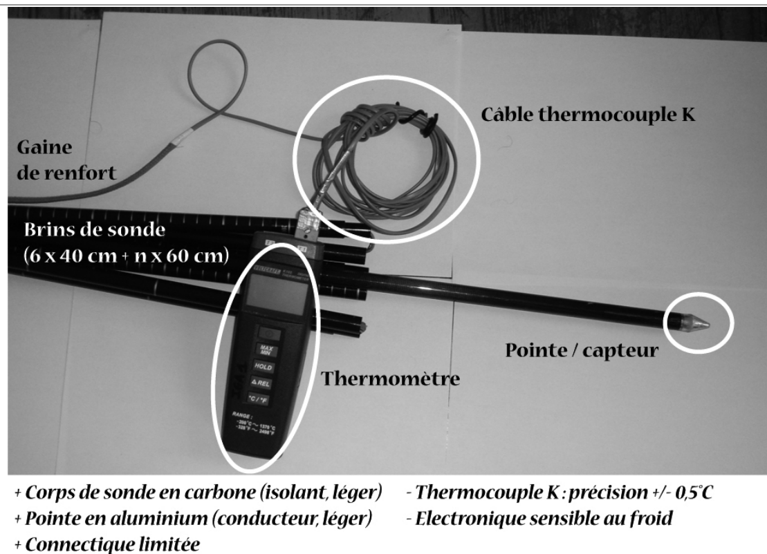
Figure III-4 : Sonde de mesure BTS à thermocouple K adaptée d'une sonde avalanche, et ses avantages (+) et inconvénient (-). Conception : IGA / GIPSA-lab. K-thermocouple BTS probe device built from an avalanche rescue probe.
