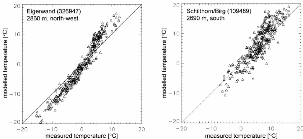
Figure I-16 : Comparaison entre les températures journalières modélisées par le modèle TEBAL et celles mesurées sur deux parois des Alpes Suisses. D'après Gruber et al. [2004b]. Daily temperatures modelled with TEBAL model as compared to the measured ones on two rockfaces in the Swiss Alps.
