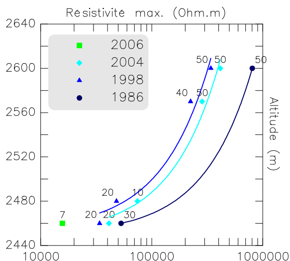
Figure VIII-16 : Valeurs de résistivité maximale mesurées sur RGL1 entre 1986 et 2006 en fonction de la position altitudinale des sondages sur le glacier rocheux (et droite de régression linéaire). Le chiffre près du symbole indique l'écartement AB/2 auquel a été mesurée la résistivité maximale. Maximal resistivity values measured on RGL1 between 1986 and 2006 according to the altitudinal position of the geoelectrical soundings.
