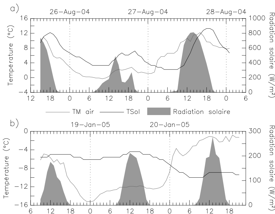
Figure IV-14 : Evolution de la température horaire de l'air (TM air), de la température du sol (TSol) et de la radiation solaire globale à la station de Laurichard (2590m) : a) en période estivale (août 2004) ; b) en période hivernale (janvier 2005). Evolution of air and ground hourly temperature and of global solar radiation at the Laurichard station in summer (a) and in winter (b).
