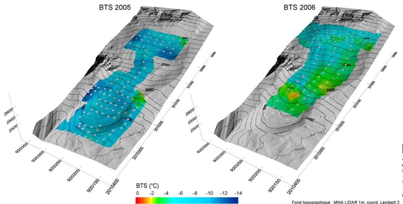
Figure IV-31 : BTS interpolées (méthode IDW) à la surface de RGL1 à partir des mesures de mars 2005 et d'avril 2006. Interpolated BTS at the RGL1 surface based on measures done on March 2005 and April 2006.
