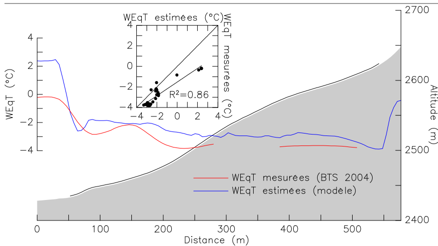
Figure VI-14 : Comparaison entre les WEqT mesurées par la méthode BTS en 2004, et les WEqT modélisées à la surface de RGL1 (profil topographique en grisé ; le glacier rocheux est délimité par la courbe noire). Comparison between measured (BTS, winter 2004) and modelled WEqT on RGL1 surface.
