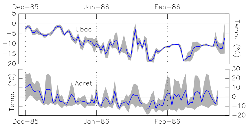
Figure IV-6: Températures mesurées à la surface du Roc Noir de Combeynot (à 3000m) : contrastes entre l'adret et l'ubac durant la saison hivernale 1985-1986. Données [Francou, 1988]. Surface temperatures at the Roc Noir de Combeynot (3000m asl.): contrasts between South and North exposed slopes during winter 1985-1986.
