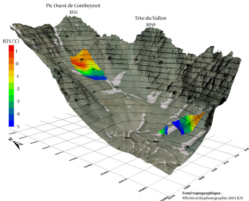
Figure VII-14 : Mesures BTS réalisées dans le vallon de la Route en mars 2005 et en avril 2006, et températures journalières de l'air (TM) et du sol enregistrées durant le mois précédant les mesures BTS dans la combe de Laurichard (LA1 : 2439 m, hors du glacier rocheux ; LA4 : 2600 m). BTS measurements performed on the Vallon de la Route in March 2005 and in April 2006, and daily air and ground temperatures at Laurichard station during the month before the measurements.
