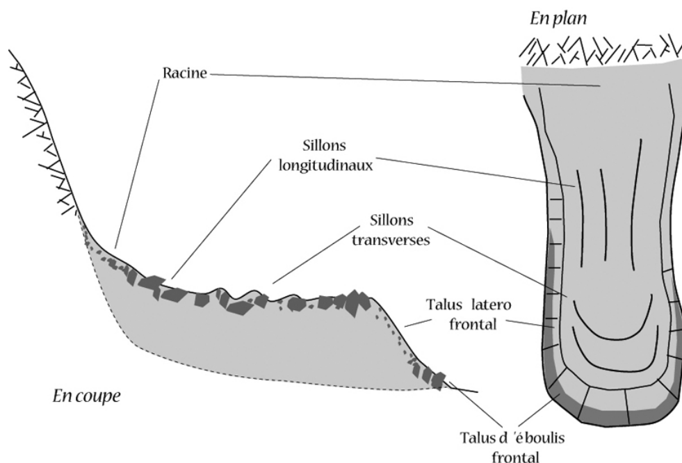
Figure VI-1 : Schéma de la morphologie typique d'une forme de fluage du pergélisol, en coupe et en plan. Typical morphology of a flowing permafrost related landform.
