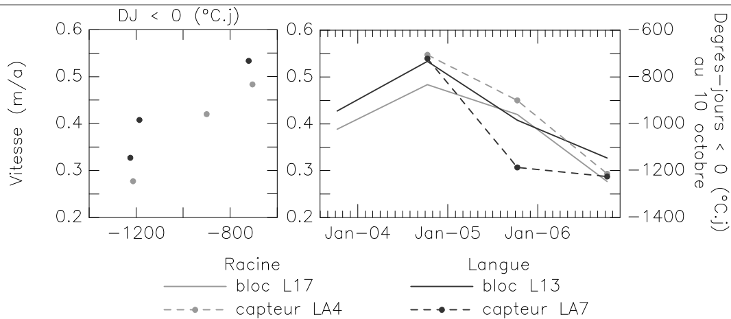
Figure VIII-1 : Comparaison annuelle entre la cinématique de RGL1 (blocs L13 et L17, vitesse annuelle) et le refroidissement de sa surface (capteurs LA7 et LA4, cumul annuel des degrés-jours négatifs sur un an, au 10 octobre) entre 2003 et 2006 : a) relation entre les deux variables, b) évolution temporelle. Données non publiées de Francou, Reynaud et Thibert. Annual comparison between RGL1 kinematics (on block L13 and L17) and the cooling of its surface (annual sum of freezing degrees-days until the 10 th Oct. on LA7 and LA4) from 2003 to 2006: a) scatter plot, b) time plot.
