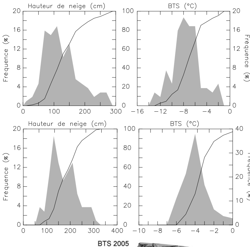
Figure IV-29 : Distribution (fréquence relative et cumulée) des hauteurs de neige et des BTS mesurées à la surface de RGL1 en mars 2005. Distribution of snow height and BTS measured on March 2004 at the RGL1 surface.
