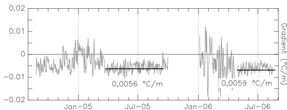
Figure IV-10 : Evolution du gradient thermique journalier entre Laurichard (2590m) et Arsine (1665m) (en trait noir, la moyenne sur les période de stabilité). Thermal gradient between Laurichard and Arsine stations (black line: average gradient during stability period).
