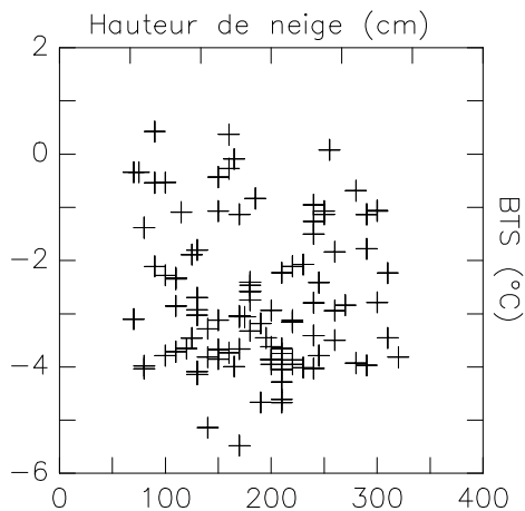
Figure IV-27 : Relation entre les hauteurs de neige et les BTS mesurées en mars 2004, à la surface de RGL1. Relationship between snow height and BTS measured on March 2004 at the RGL1 surface.
