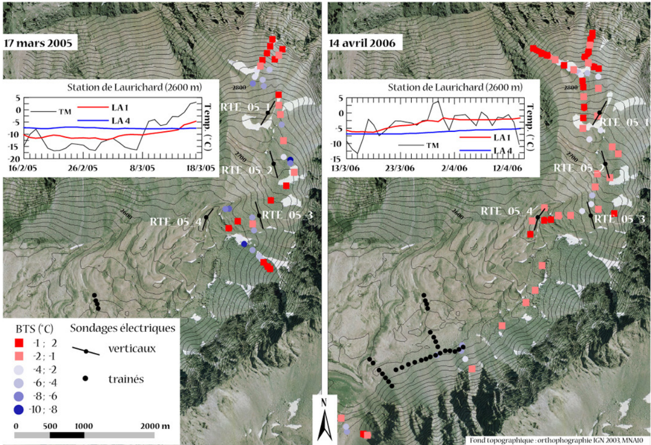
Figure VII-14 : Mesures BTS réalisées dans le vallon de la Route en mars 2005 et en avril 2006, et températures journalières de l'air (TM) et du sol enregistrées durant le mois précédant les mesures BTS dans la combe de Laurichard (LA1 : 2439 m, hors du glacier rocheux ; LA4 : 2600 m). BTS measurements performed on the Vallon de la Route in March 2005 and in April 2006, and daily air and ground temperatures at Laurichard station during the month before the measurements.
