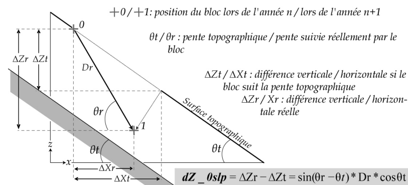
Figure VIII-7: Explication schématique du calcul de la quantité cinématique dZ_{0slp} (variation verticale compensée par la pente locale). Schematic explanation for the computation of the kinematics quantity dZ_{0slp} .
