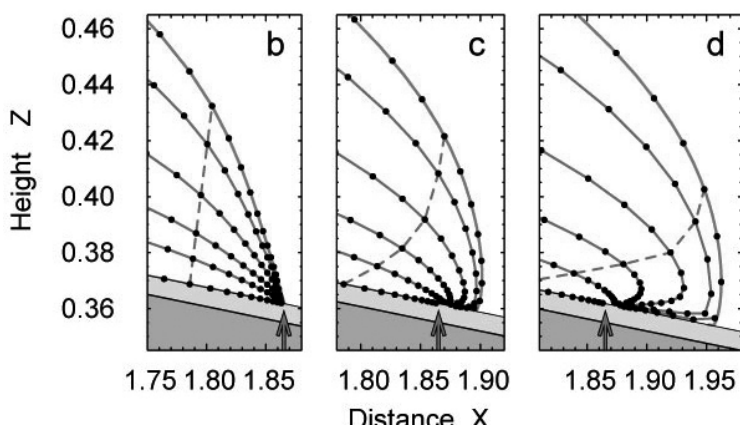
Figure I-13 : modélisation de la progression du front d'un glacier par écoulement « over-riding ». (sans glissement basal) D'après Leysinger Vieli [2004]. Modelling of the rock glacier front advance by "over-riding" flow.
