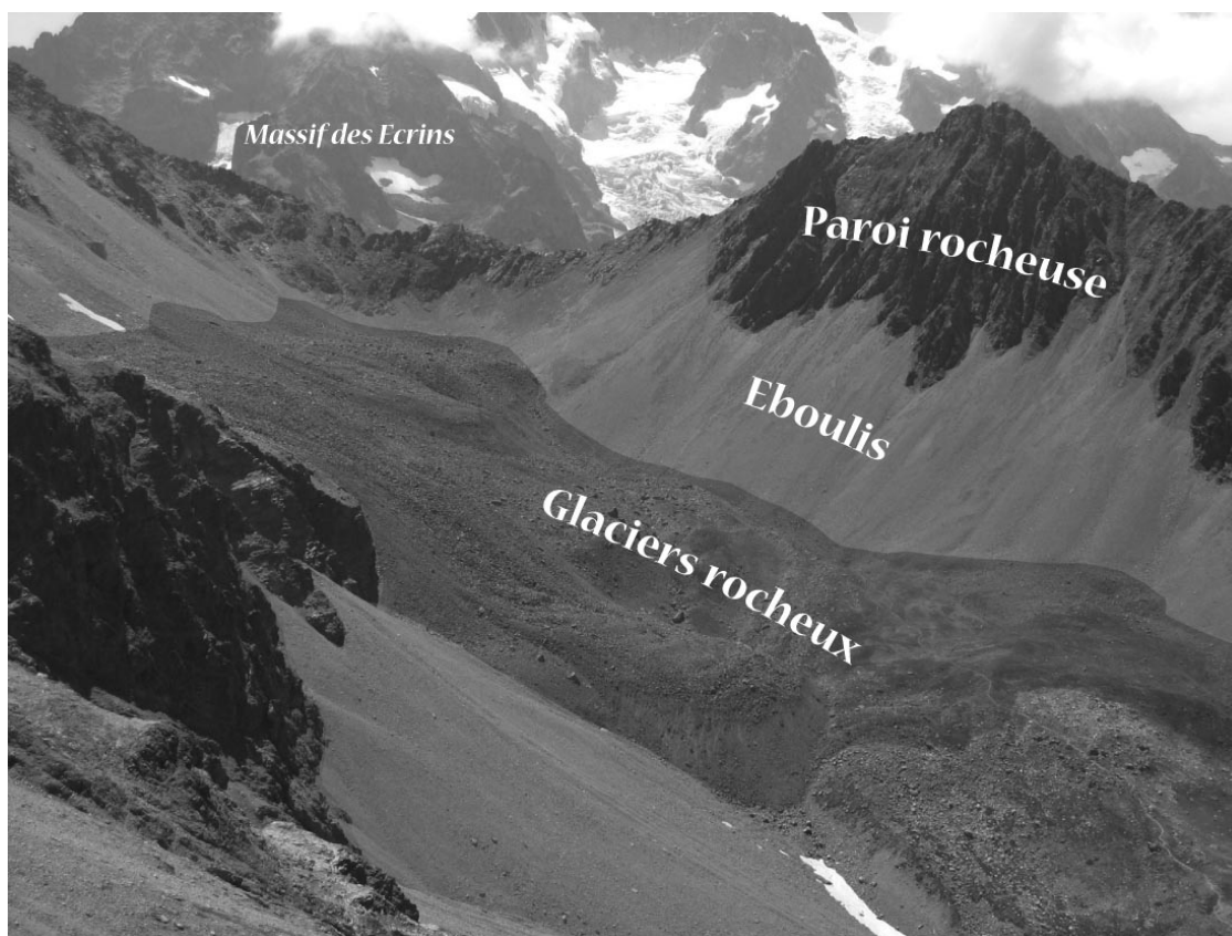
Figure II-9 : Aperçu d'une morphoséquence corniche/éboulis/forme fluante sur le massif du Combeynot (combe de Laurichard). Overview of a morphosequence rockface/scree slope/creeping landform on the Combeynot Massif.
