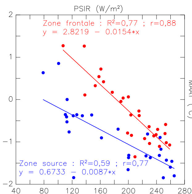
Figure VI-6 : Relation (régression linéaire) entre la radiation solaire potentielle reçue au sol (PSIR) et la température annuelle moyenne de l'air (MAAT) au niveau de la zone source (points bleus) et de la zone terminale (points rouges) des glaciers rocheux du massif du Combeynot. Linear relationship between MAAT and PSIR at the rooting zone (blue points) and frontal zone (red points) of the rockglaciers of the massif.
