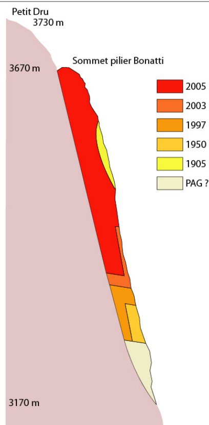
Figure I-21 : Evolution, au cours du XX ème siècle, des volumes affectés par des écoulements sur la paroi NW du Petit Dru, massif du Mont Blanc. D'après Ravanel et al. [2007]. Evolution of the volumes affected by rockfall during the 20th century on the NW face of the Petit Dru.
