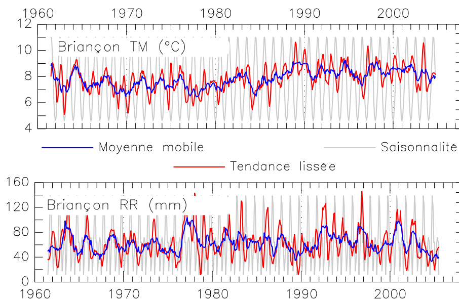
Figure II-26 : Résultats de la décomposition saisonnière des températures et des précipitations mensuelles de 1961 à 2005 enregistrées à la station de Briançon. Données Météo France. Results of the seasonal decomposition of the monthly temperatures and precipitations at Briançon.
