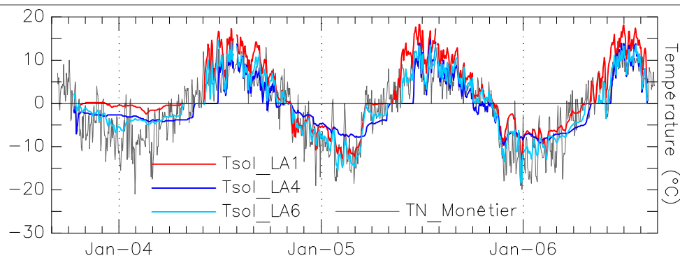
Figure IV-18 : Evolution de la température du sol mesurée aux sites LA1, LA4 et LA6 (localisation : voir fig. III-2) du glacier rocheux 1 (RGL1) de la combe de Laurichard et de la température minimale de l'air (TN) à la station de Monétier, entre octobre 2003 et août 2006. Evolution of the ground temperature recorded at sites LA1, LA4 and LA6 on RGL1 and of the air temperature at Monétier station, between October 2003 and August 2006.
