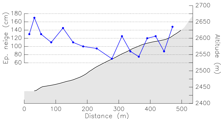
Figure IV-24 : Hauteurs de neige relevées sur un profil longitudinal de RGL1 (profil topographique en grisé; le glacier rocheux est délimité par la courbe noire) le 5/11/2003. Snow heights measured on a longitudinal profile of RGL1 on Nov. 5 th 2003.
