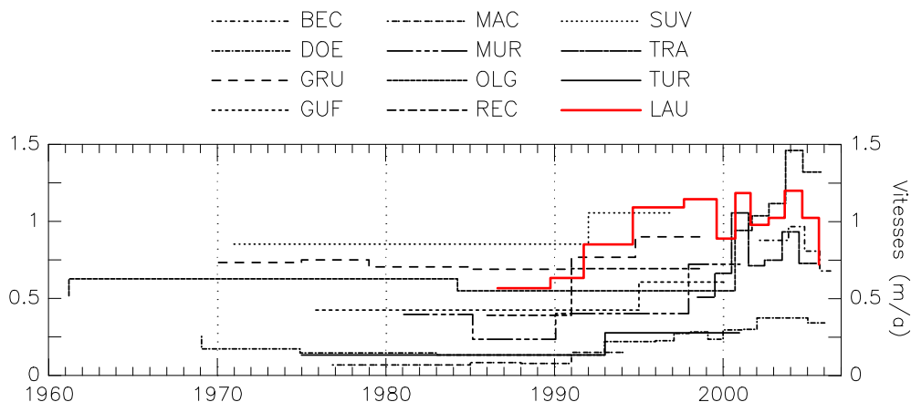
Figure VIII-11 : Evolution des vitesses moyennes d'écoulement de divers glaciers rocheux alpins au cours des quatre dernières décennies. BEC : Becs-de-Bosson (Suisse), d'après Perruchoud & Delaloye, [2006] ; DOE : Doesen (Autriche), d'après Kaufman et al. , [2006] ; GRU : Gruben, GUF : Gufer, MAC : Macun, MUR : Muragl, REC : Rechy, SUV : Suvretta, TUR : Turtmann (Suisse), d'après Käab et al. , [2006b] ; OLG : Olgrube (Autriche), d'après Hausmann et al. , [2006] ; LAU : Laurichard (France), d'après Francou & Reynaud, [1992], et données non publiées de Francou, Reynaud et Thibert. Evolution of the flow velocities of various rockglaciers in the European Alps during the last four decades.
