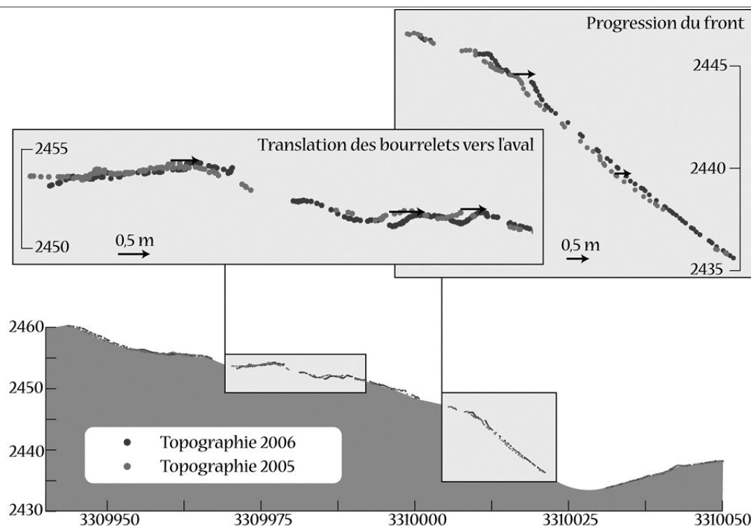
Figure V-17 : Comparaison interannuelle des surfaces topographiques (profil L3, voir fig. V-14 pour la localisation) à partir des MNT hautes résolution de 2005 et 2006. Comparison between topographic surfaces (profile L3, see fig. V-12) from the 2005 and the 2006 high resolution DEM.
