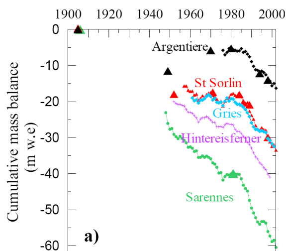
Figure II-23 : Evolution des bilans de masse cumulés de différents glaciers alpins au cours du XX ème siècle. D'après [Vincent et al. , 2005]. Evolution of the cumulative mass balances of some Alpine glaciers during the 20 th century.
