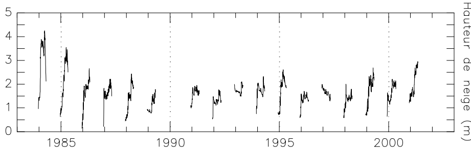
Figure II-30 : Hauteurs de neige au site de la Toura (Isère, station des Deux Alpes) entre 1984 et 2001 (entre décembre et avril). Snow height at the site of La Toura (Isère) between 1984 and 2001 (from December to April).
