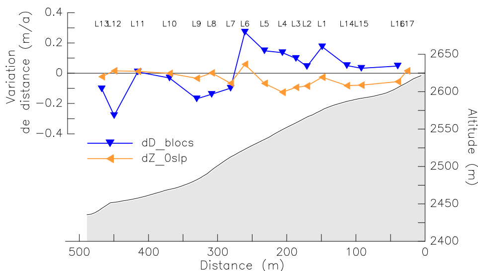
Figure V-6 : Moyenne (1986-2006) de deux quantités cinématiques calculées à partir des mesures géodésiques sur la ligne du suivi géodésique de RGL1 : dD\_blocs , variation de distance entre deux blocs successifs (dénommés L1 à L17), et dZ\_0slp , variation d'altitude de chaque bloc, indépendamment de la pente locale (profil topographique en grisé ; le glacier rocheux est délimité par la courbe noire). D'après des données non publiées de Francou, Reynaud et Thibert. Mean values of two kinematic quantities: dD\_blocs , interannual variation of distance between two successive blocks; dZ\_0slp , interannual variation of elevation of each block independently of the local slope.
