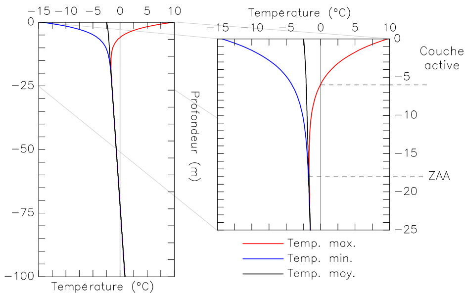
Figure IV-5: Simulation du profil thermique du sol d'après les mesures de température à l'interface air/roche obtenues par Francou [1988] à 3000m sur l'ubac du Roc Noir de Combeynot. Code du modèle de diffusion thermique: S. Gruber, Université de Zurich. Simulated ground thermal profile using the measured temperatures at air/rock interface obtained by Francou [1988] on the Roc Noir de Combeynot (3000m asl.).
