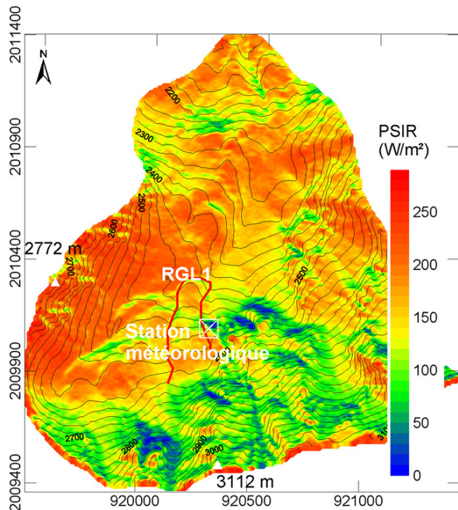
Figure IV-12: Radiation solaire potentielle (PSIR) moyenne estivale (juin-juillet-août) dans la Combe de Laurichard, calculée par le modèle TEBAL (S. Gruber, université de Zurich). Potential Incoming Solar Radiation during summer in the Combe de Laurichard catchment.
