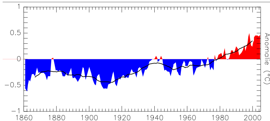
Figure II-20 : Anomalie thermique annuelle globale calculée à partir des données HadCRUT3, et moyenne lissée. Données tirées de [Brohan et al. , 2006]. HadCRUT3 global temperature anomaly time-series at annual resolution and smoothed mean.
