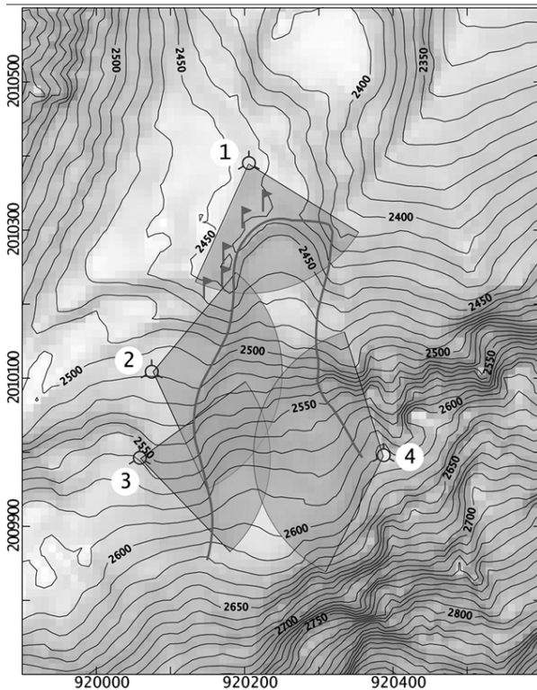
Figure III-12 : Localisation des stations et des fenêtres utilisées pour les mesures au LIDAR terrestre en septembre 2005 et septembre 2006 sur le glacier rocheux 1 de Laurichard (RGL1). Les fanions marquent l'emplacement des points fixes mesurés au DGPS pour le géoréférencement des nuages de points. Coord. Lambert 2, nord en haut de la carte. Location of the standing stations and scanning windows of the terrestrial LIDAR used in Sept. 2005 and Sept. 2006 on RGL1. Triangular markers are control points surveyed with DGPS for georeferencing the cloud points.
