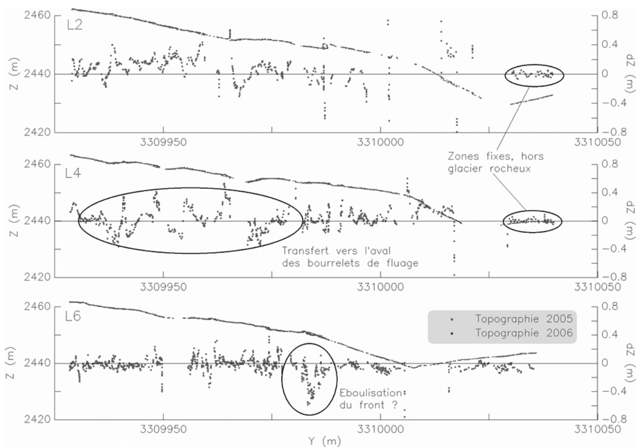
Figure V-15 : Ecarts verticaux entre les MNA haute résolution de 2005 et 2006 le long de trois profils longitudinaux. Vertical differences between 2005 and 2006 high resolution DEM along three longitudinal profiles.
