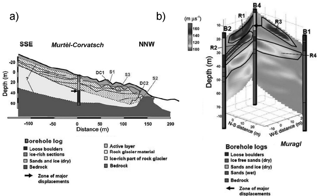
Figure I-10 : Comparaison entre les résultats de sondages géophysiques 2D (tomographie électrique, tomographie sismique, géoradar) et les informations des forages : a) pour le glacier rocheux de Murtèl-Corvatsch ; b) pour le glacier rocheux de Muragl. D'après Maurer & Hauck [2007]. Comparison between geophysical soundings results and boreholes information for: a) the Murtèl-Corvatsch rock glacier; b) the Muragl rock glacier.
