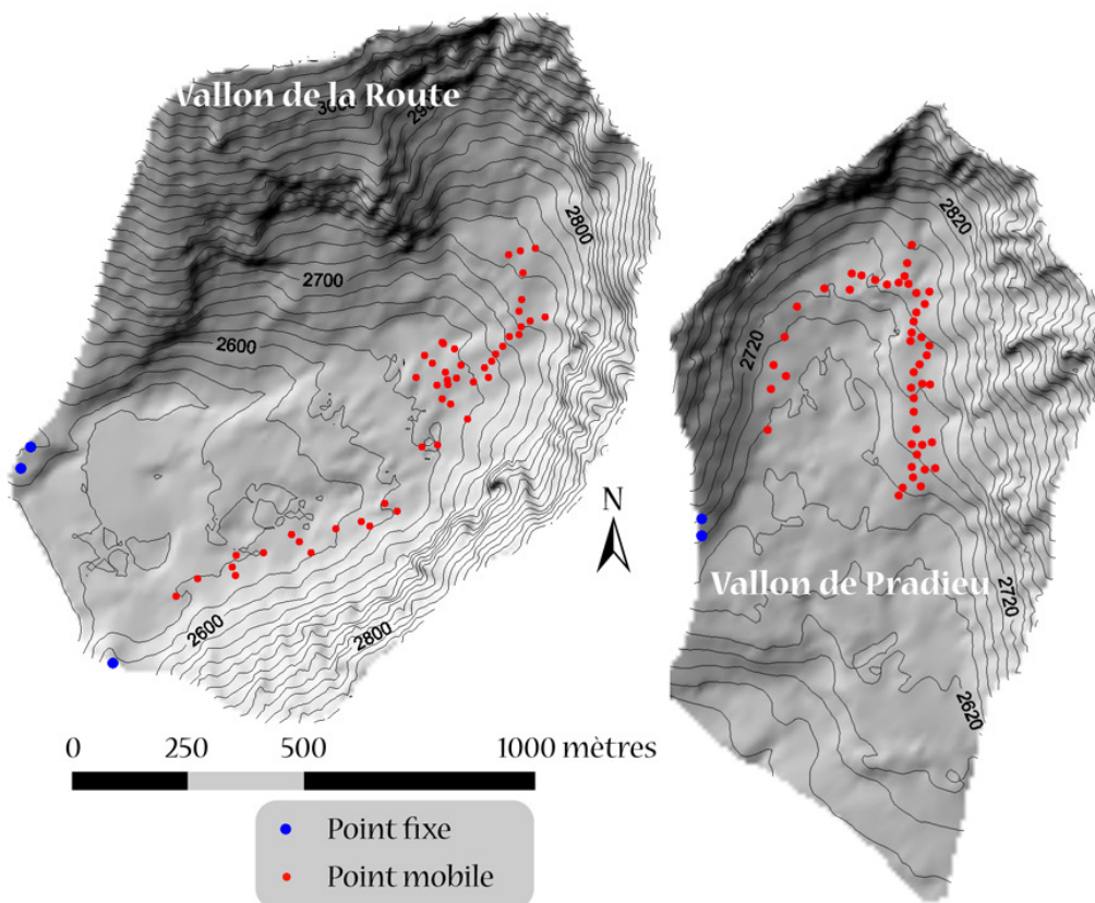
Figure V-19 : Emplacement des points fixes et mobiles des réseaux DGPS mis en place dans les vallons de la Route et de Pradieu (cf. fig. II-12 pour la localisation des vallons au sein du massif du Combeynot). Location of the fixed and mobile points of the DGPS networks, on Vallon de la Route and Vallon de Pradieu.
