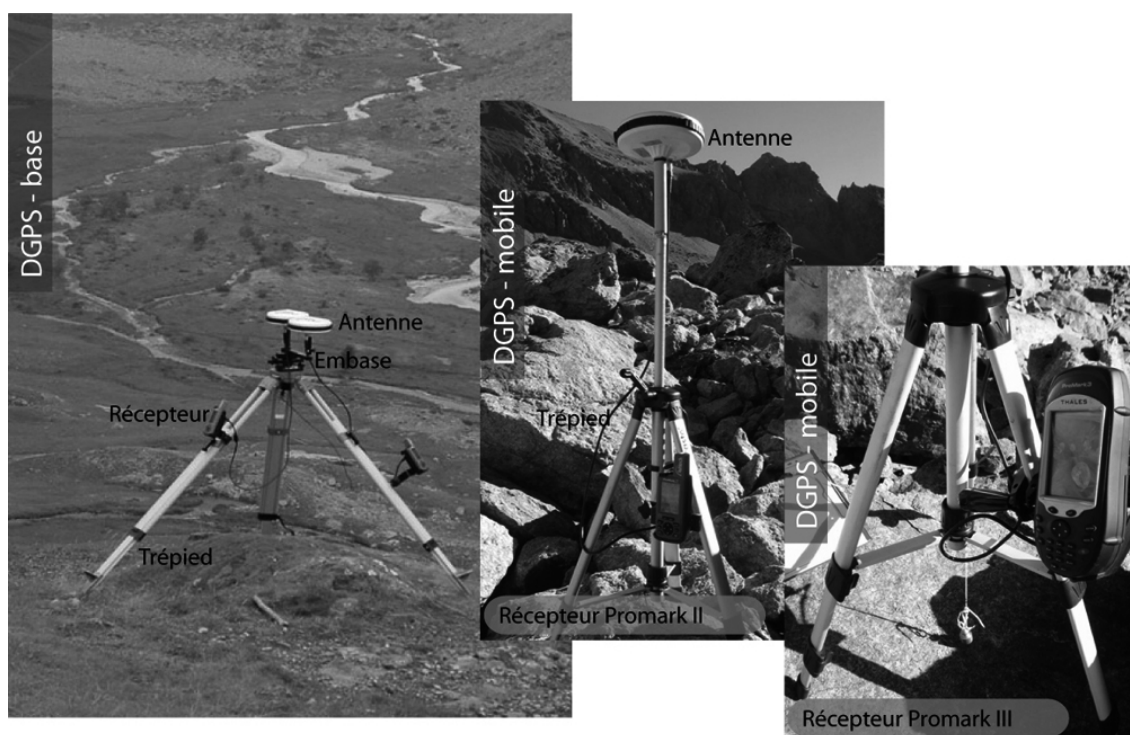
Figure III-8 : Aperçu du matériel GPS : à gauche, récepteur de base utilisé pour l'initialisation du mode Stop-&-Go ; au centre, antenne, récepteur et trépied avec le Promark II ; à droite, idem, avec le Promark III. Overview of the DGPS devices used for the field works.
