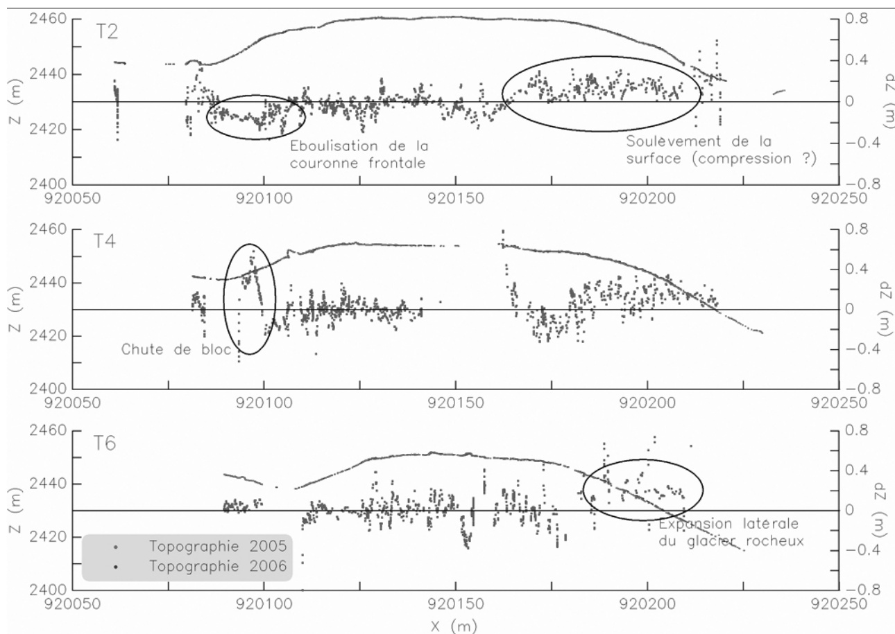
Figure V-16 : Ecarts verticaux entre les MNA haute résolution de 2005 et 2006 le long de trois profils transversaux. Vertical differences between 2005 and 2006 high resolution DEM along three transversal profiles.
