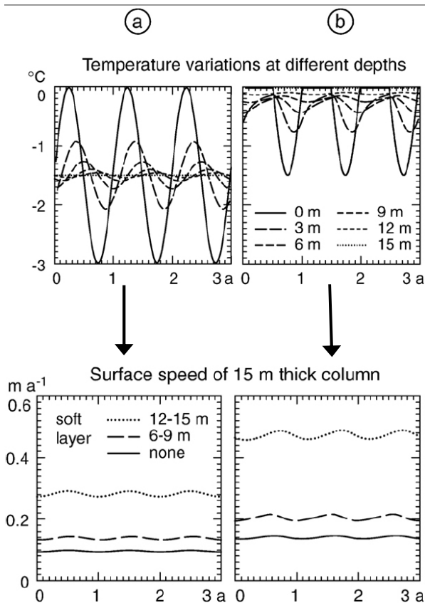
Figure VIII-5 : Simulation de la température à différentes profondeurs sur trois cycles annuels, sous une évolution sinusoïdale de la température de surface, et de la réponse de la cinématique de surface selon différentes profondeurs du niveau cisailant et (a) pour un pergélisol froid, (b) pour un pergélisol tempéré. Tiré de Käab et al. , [2006b].
