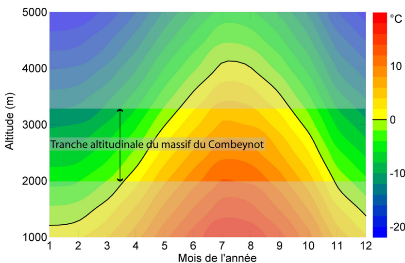
Figure II-16 : Evolution moyenne (1961-1990) mensuelle de la température de l'air entre 1000 et 5000 m d'altitude dans le secteur Oisans-Briançonnais et emprise altitudinale du massif du Combeynot. Données Météo France (cf. tabl. 3). Mean monthly evolution of air temperature at elevations between 1000 and 5000 m in the Oisans-Briançonnais area, and altitudinal range of the Combeynot Massif.
