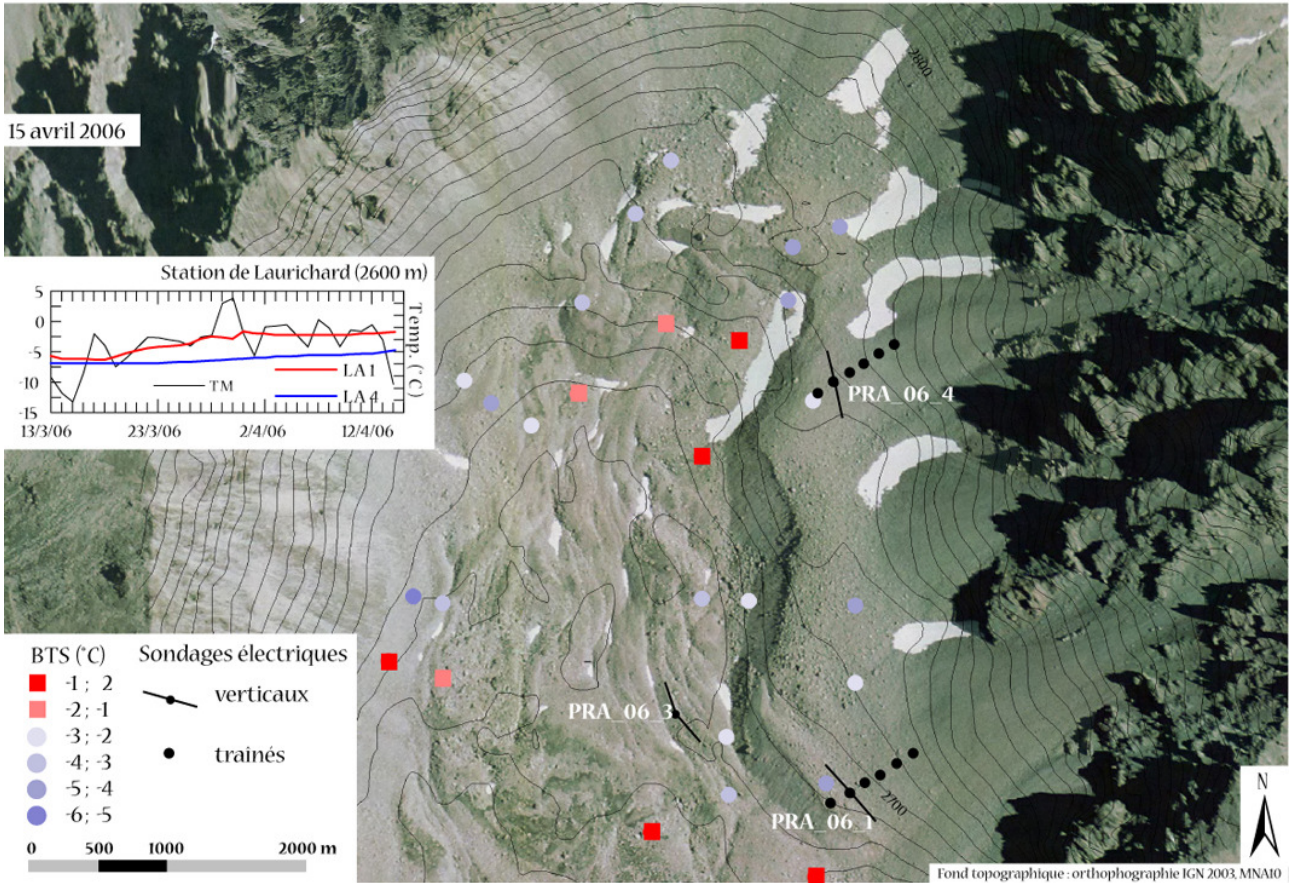
Figure VII-20 : Mesures BTS réalisées dans le vallon de Pradiou en avril 2006, et températures journalières de l'air (TM) et du sol enregistrées durant le mois précédent les mesures BTS dans la combe de Laurichard (LA1: 2439 m, hors du glacier rocheux; LA4: 2600 m). Les emplacements des sondages géoélectriques sont également indiqués. BTS measurements performed on the Vallon de Pradiou in April 2006, and daily air and ground temperatures at Laurichard station during the month before the measurements. The location of the geoelectrical soundings is also indicated.
