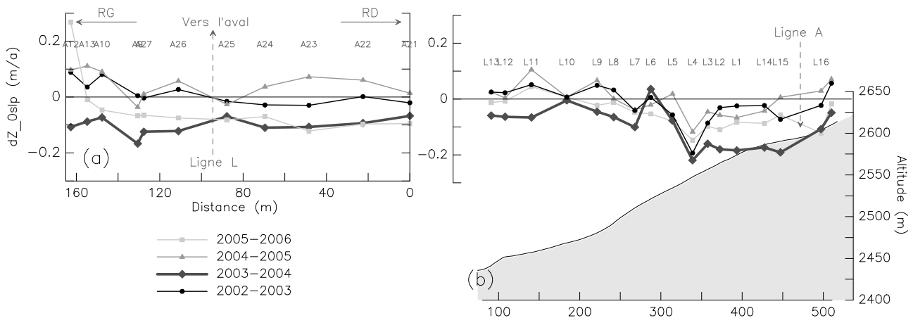
Figure VIII-8 : Profils annuels de variation verticale compensée par la pente ( dZ_{0slp} ) de la surface de RGL1, entre 2002 et 2006 : (a) ligne A, transverse à la racine de RGL1 (indications de position des bords gauche et droit du glacier rocheux, et de la ligne L ; profil topographique en gris ; le glacier rocheux est délimité par la courbe noire) ; (b) ligne L, longitudinale (position de la ligne A indiquée). Annual profiles of vertical variation with slope compensation ( dZ_{0slp} ) at the RGL1 surface, between 2002 and 2006: (a) line A, transverse to RGL1 root; (b) line L, along the main flowing axis of RGL1.
