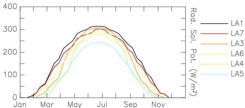
Figure IV-17: Radiation solaire potentielle reçue au sol à l'emplacement des MTD (Miniature Temperature Datalogger) du glacier rocheux de Laurichard. D'après les données du modèle TEBAL (S. Gruber). Potential solar incoming radiation at MTD sites on Laurichard rockglacier (calculations from TEBAL model, S. Gruber).
