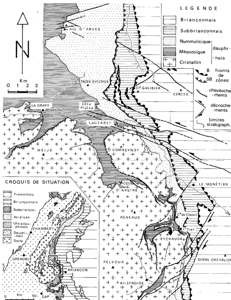
Figure II-5 : Structure géologique schématique du massif du Combeynot et de la bordure E du massif Ecrins-Pelvoux (tiré de [Bravard & Gidon, 1979]). Schematic overview of the structural settings of the Combeynot massif, and its neighbouring Ecrins-Pelvoux massif.
