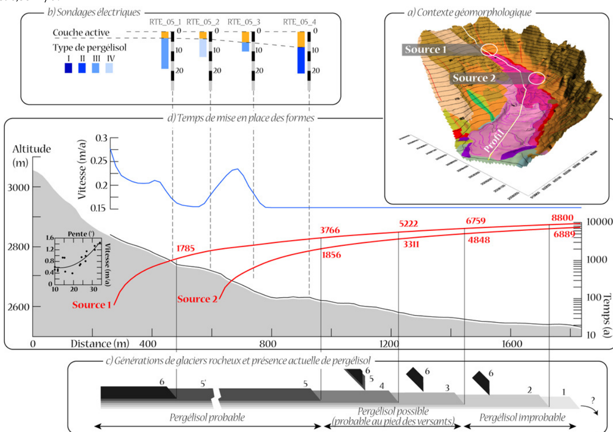
Figure VII-19 : Le pergélisol à l'échelle du vallon de la Route : a) contexte géomorphologique (avec la localisation des zones source principales et du profil topographique) ; b) résultats des sondages électriques (pour la typologie du pergélisol, cf. chap. III, § 3.1) ; c) principales générations observables de glaciers rocheux (ainsi que les formes provenant des versants ubac) et présence de pergélisol ; d) hypothèse de mise en place des formes fluantes (en rouge le temps de progression ; en noir la vitesse de progression) d'après la relation « pente / vitesse » établie pour RGL1 (cf. chap. V, § 1.2). Permafrost at the catchment scale in the Vallon de la Route: a) geomorphological context (with location of the main source zones and of the profile); b) results of the electrical soundings (for the types of permafrost, cf. chap. III, § 3.1); c) main visible generations of rockglaciers and present permafrost presence; d) time needed to acquire the present morphology (in red the duration of advance; in black the advance speed) as suggested by the relation "slope angle/surface velocity" on RGL1.
