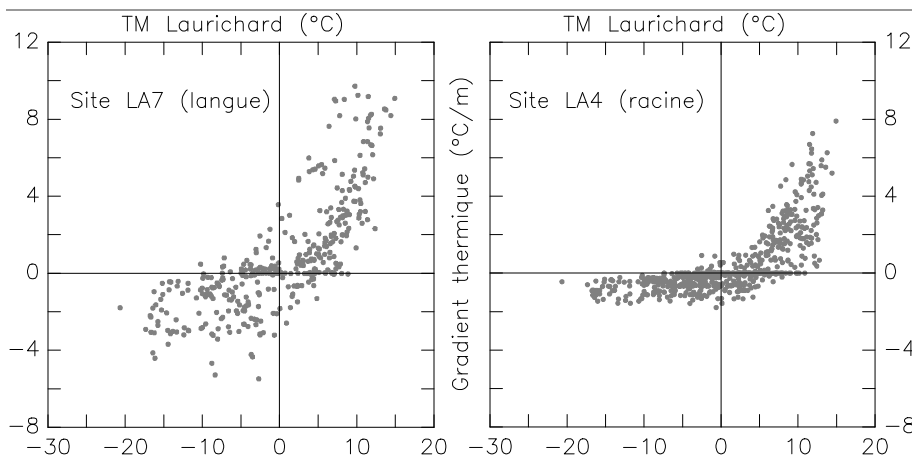
Figure IV-23 : Relation entre le gradient thermique journalier dans le premier mètre de la couche active de RGL1, aux sites LA4 (2600m) et LA7 (2451m), et la température de l'air moyenne journalière (TM) à la station de Laurichard. Relationship between the thermal gradient within the first meter of the RGL1 active layer at sites LA4 and LA7 and the air temperature at Laurichard station.
