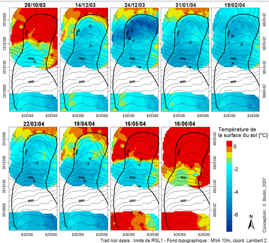
Figure IV-35 : Evolution des températures de la surface de RGL1, extrapolées d'après les mesures BTS de mars 2004 et le suivi thermique sur 5 sites du glacier rocheux (explications dans le texte). Evolution of the ground surface temperatures extrapolated after the BTS measurements and the thermal monitoring on 5 sites of the rock glacier (see text for explanation).
