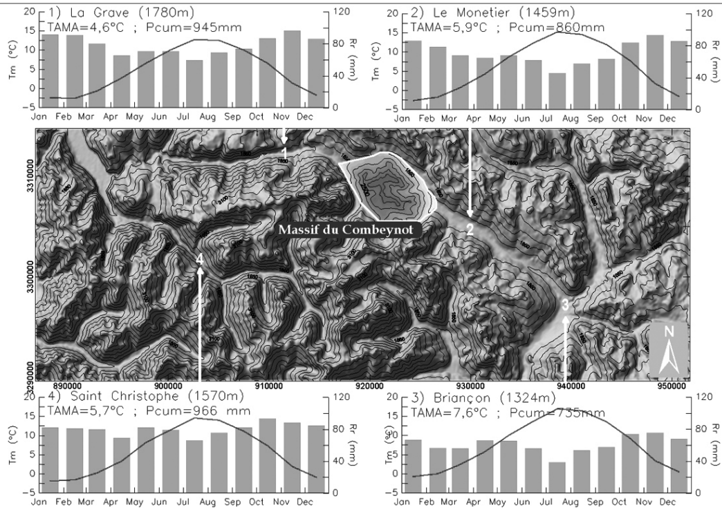
Figure II-12 : Normales climatiques des températures (courbes) et des précipitations (barres) mensuelles de quatre stations du réseau Météo France dans le secteur Oisans-Briançonnais (période 1961-1990, sauf La Grave et Saint Christophe, cf. tableau 2), et leur localisation par rapport au massif du Combeynot (MNA SRTM, 100m, coord. Lambert 3 en m). Normal climatic values of 4 Météo France stations in the Oisans-Briançonnais area (1961-1990 period) and their location in the vicinity of the Combeynot massif.
