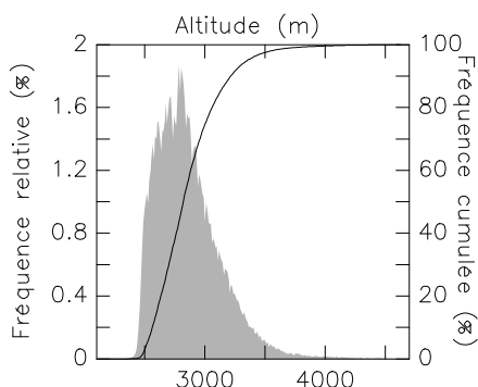
Figure IX-13 : Distribution de l'altitude des surfaces de type « formation superficielle » (pentes comprises entre 25 et 40°) potentiellement concernées par pergélisol dans les Alpes françaises, d'après le modèle « Alpes du sud ». Distribution of the altitude of the surfaces "slope deposits" that are potentially concerned with the permafrost in the French Alps, after the "Southern Alps" model.
