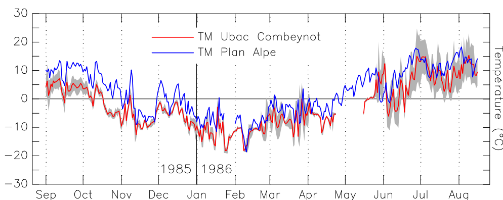
Figure IV-4 : Température moyenne (TM) de l'interface air/roche (courbe rouge ; en grisé, l'enveloppe TN/TX) sur l'ubac du Roc Noir de Combeynot, à 3000m d'altitude (données [Francou, 1988]), et température moyenne journalière à la station du Plan de l'Alpe (2065m ; courbe bleue) durant l'année 1985-1986. Mean temperature (in greyish, the Tn/Tx range) of air/rock interface at the Roc Noir de Combeynot, 3000m asl. and mean daily air temperature at Plan de l'Alpe station during 1985-1986.
