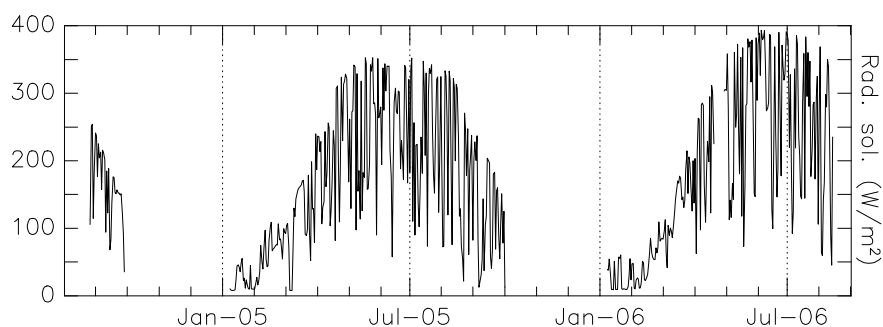
Figure IV-11 : Evolution de la radiation solaire globale à la station de Laurichard (2590m) entre août 2004 et août 2006. Measured global solar radiation at Laurichard station between august 2004 and august 2006.
