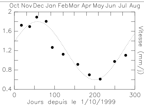
Figure VIII-3 : Vitesse calculée de la surface du glacier rocheux de Muragl lors de l'année 1999, et courbe sinusoïdale ajustée aux vitesses. Données et équation de Arenson [2002]. Computed surface velocity on the Muragl rockglacier during 1999 and adjusted sinusoidal curve.
