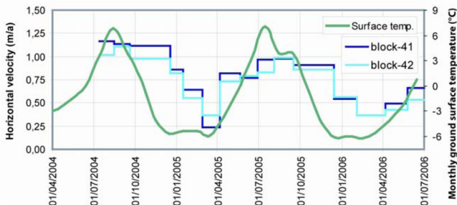
Figure VIII-4 : Variations saisonnières des vitesses horizontales de deux blocs à la surface du glacier rocheux des Becs-de-Bossons (Suisse) et évolution de la température à la surface du sol. Tiré de Perruchoud et Delaloye, [2006]. Seasonal variations of horizontal velocities of two blocks at the surface of Becs-de-Bosson rockglacier, and evolution of the ground surface temperature.
