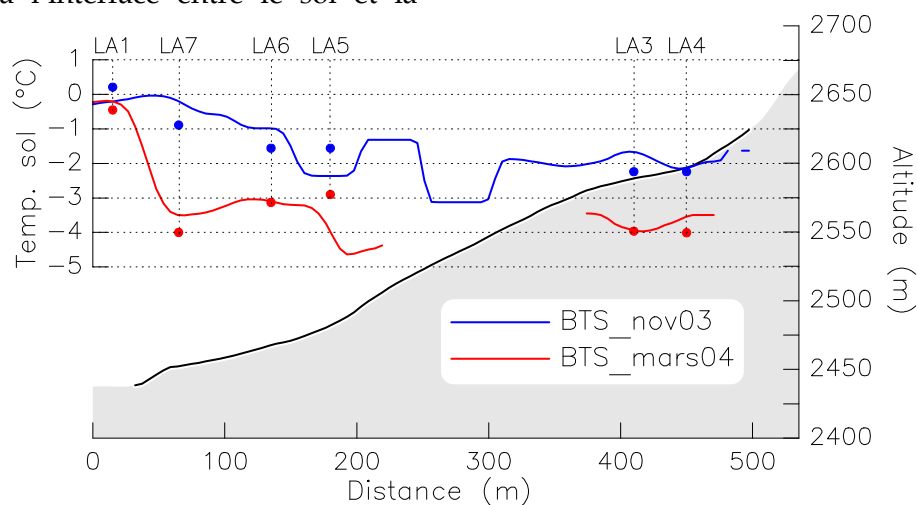
Figure IV-32 : Profils thermiques relevés lors de campagnes BTS en novembre 2003 et en mars 2004 à la surface de RGL1, et comparaison avec les valeurs moyennes (des 15 jours précédents la mesure BTS) du suivi thermique sur 5 sites du glacier rocheux (profil topographique en grisé ; le glacier rocheux est délimité par la courbe noire). Thermal profiles from BTS campaigns on Nov. 2003 and Mar. 2004 on RGL1, and comparison with mean values (15 days before the BTS measurements) recorded by thermal monitoring on 5 sites.
