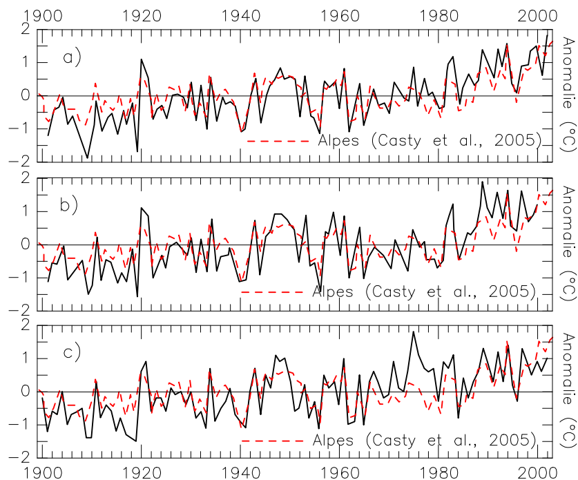
Figure II-22 : Anomalie thermique annuelle (écart à la moyenne 1900-2000) aux stations : a) de Sonnblick (3206m, Autriche, [Klein Tank et al. , 2002]) ; b) de Saentis (2500m, Suisse, [Klein Tank et al. , 2002]) ; c) du Grand St Bernard (2472m, Suisse, [Harris et al. , 2003]). Données Alpes tirées de [Casty et al. , 2005]. Annual mean temperature anomaly at a) the Sonnblick station (3206m, Austria); b) the Saentis station (2500m, Switzerland); c) the Grand St Bernard station (2472m, Switzerland).
