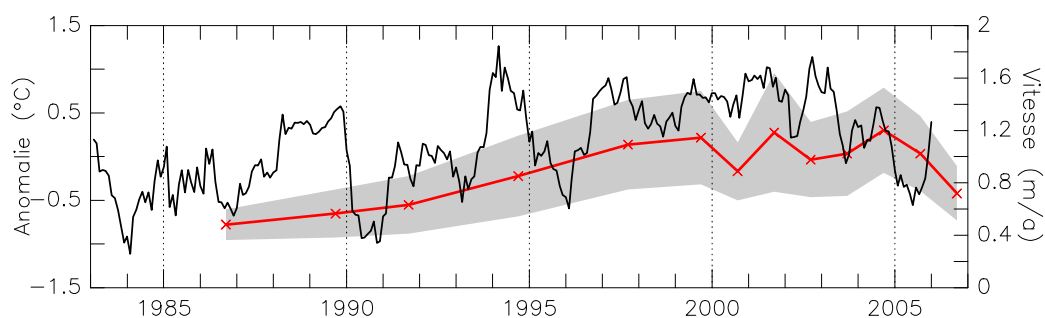
Figure VIII-12 : Evolution de la vitesse d'écoulement de RGL1 (courbe rouge : moyenne des blocs 1 à 3, 5 à 8 et 10 à 12 du profil longitudinal ; en grisé, l'intervalle \pm 1\sigma ), et de la température de l'air à la station du Monétier (courbe noire, anomalie thermique par rapport à la moyenne 1961-1990, données mensuelles lissées sur 12 mois) entre 1984 et 2006. Données non publiées de Francou, Reynaud et Thibert, et données Météo France. Evolution of the mean velocity of the blocks of the line L from 1986 to 2006 (red curve; in greyish, the \pm 1\sigma interval) and of the monthly air temperature (12 months smoothed mean).
