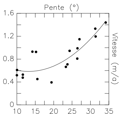
Figure V-5 : Relation entre la vitesse de RGL1 (ligne L, moyenne sur la période 1986-2006) et la pente. Relationship between the surface velocity of RGL1 and the slope angle.
