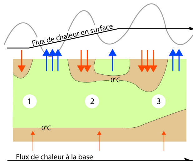
Figure I-18 : Evolution thermique simplifiée du pergélisol sous l'effet d'un réchauffement de la surface (flèche : flux de chaleur, rouge = conduisant à un réchauffement du sol, bleu = conduisant à un refroidissement ; le temps s'écoule de gauche à droite ; voir le texte pour les explications). Simplified thermal evolution of permafrost under a warming of the surface (time is flowing from left to right; see text for explanation).
