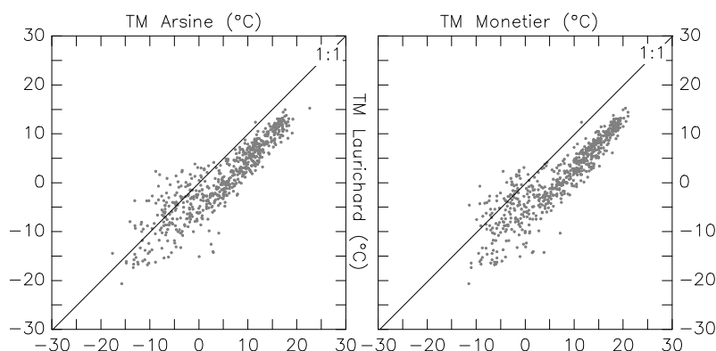
Figure IV-9 : Comparaison des températures journalières moyennes (TM) mesurées à Laurichard (ordonnée) et des températures à Arsine et au Monétier (abscisses) entre août 2004 et août 2006. Scatter plots of daily temperatures measured at Laurichard and Arsine and Monétier temperatures between August 2004 and August 2006.
