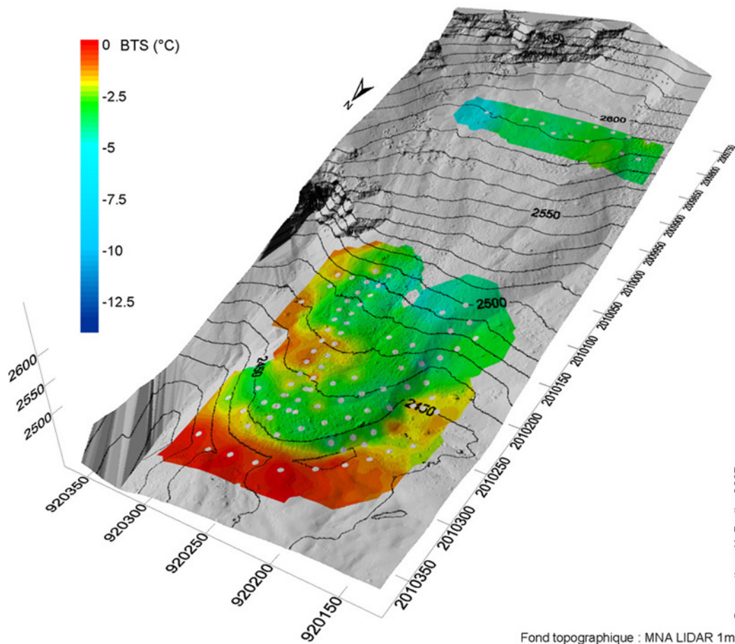
Figure IV-28 : BTS interpolées (méthode IDW : Inverse Distance Weighting) à la surface de RGL1 à partir des mesures de mars 2004. Coordonnées Lamb. 2. Interpolated BTS at the RGL1 surface based on measures done on March 2004.
