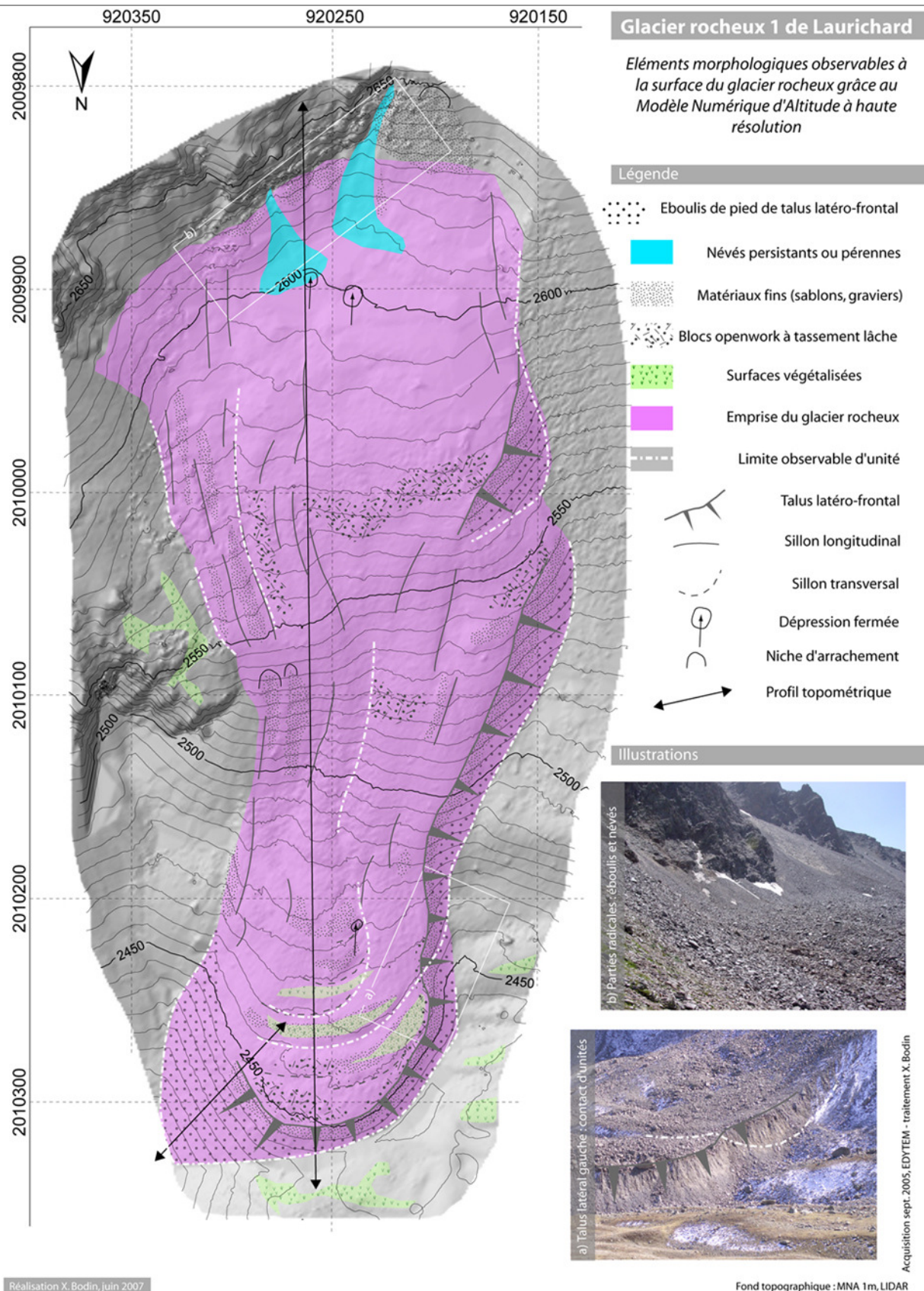
Figure V-9 : Eléments morphologiques du glacier rocheux 1 de Laurichard d'après le MNT haute résolution (2005, résolution 1m) et localisation des deux profils topométriques. Morphological characteristics of RGL1 as interpreted from the high resolution DTM and location of the two topometric profiles.
