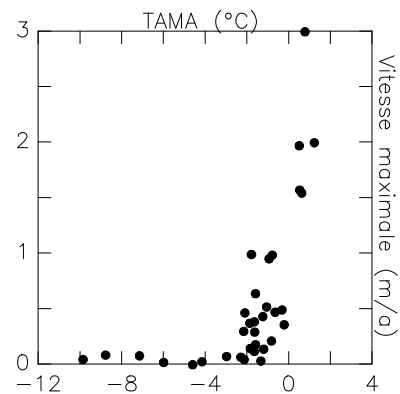
Figure VIII-2 : Relation entre la température annuelle moyenne de l’air (TAMA) au front des glaciers rocheux des Alpes suisses orientales et leur vitesse maximale en surface. Données tirées de Frauenfelder [2004]. Relationship between maximal surface velocity and mean annual air temperature (MAAT) at the Eastern Swiss Alps rockglacier front.
