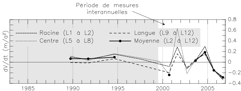
Figure V-7 : Variation interannuelle des vitesses (en blanc, les périodes durant lesquelles des mesures annuelles sont disponibles) des blocs de la ligne L entre 1989 (les années précédentes, qui sont discontinues car les données de certains blocs sont manquantes, n'ont pas été incluses dans le calcul) et 2006, sur le glacier rocheux 1 de Laurichard. Sont indiquées les moyennes de l'ensemble de la ligne (moyenne L2 à L12), de la portion haute (L1 à L2), de la portion centrale (L5 à L8) et de la langue (L9 à L12). Données non publiées de Francou, Reynaud et Thibert. Rate of change of the velocity of RGL1 along the geodetic line L (on the root, L1-L2; on the central part, L5-L8; on the tongue, L9-12; and average of line L, L2-L12) between 1984 and 2006.
