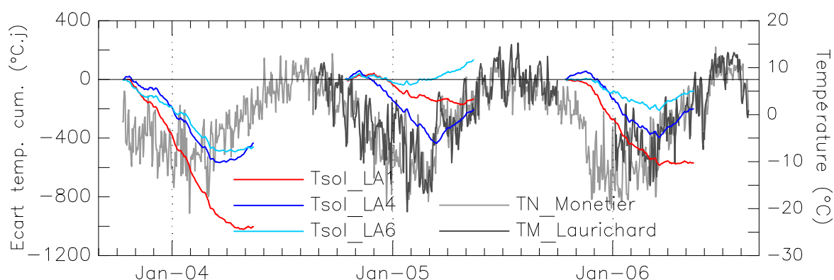
Figure IV-19 : Cumul des écarts journaliers entre les températures de l'air (TN, température minimale ; TM, température moyenne) et les températures du sol, aux sites LA1, LA4 et LA6, durant les hivers 2003 à 2006 (du 15/10 au 15/05). Cumulated differences between air temperature and ground surface temperature at sites LA1, LA4 and LA6, during winters 2003 to 2006.
