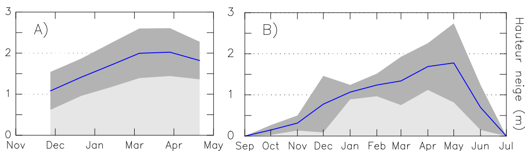
Figure II-17 : A) épaisseur moyenne (courbe bleue ; en grisé sombre, l'enveloppe +/- 1σ) du manteau neigeux sur le site de La Toura (2590m d'altitude, 20km à l'ouest du col du Lautaret) sur la période 1983-2001 ; B) épaisseur moyenne (courbe bleue ; en grisé sombre, l'enveloppe +/- 1σ) du manteau neigeux dans la Combe de Laurichard (2450m d'altitude, massif du Combeynot sur la période 1979-1986. Données Météo France et [Francou, 1988]. A) mean thickness (in greyish, the +/- 1σ envelope) of the snow cover at La Toura site for the 1983-2001 period; B) mean thickness (in greyish, the +/- 1σ envelope) of the snow cover at Combe de Laurichard site for the 1979-1986 period.
