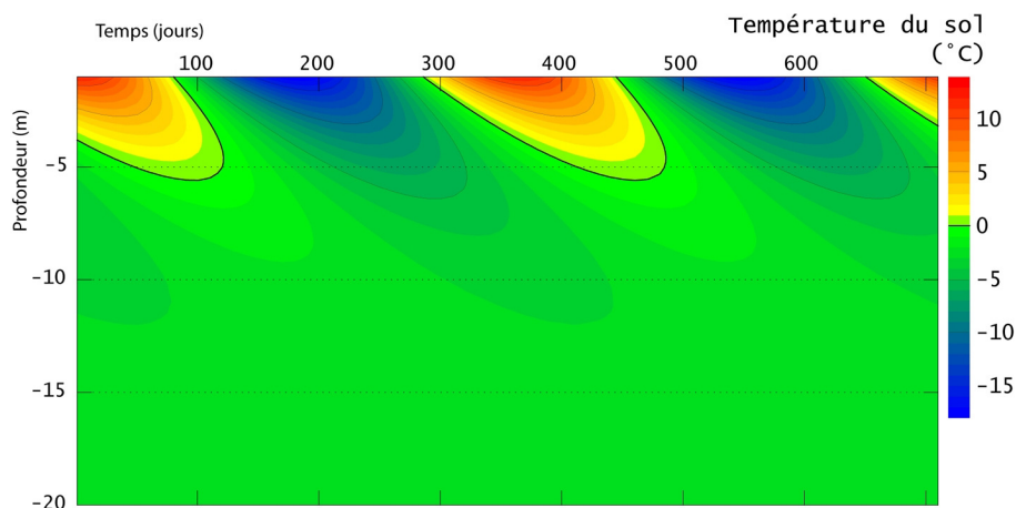
Figure I-3 : Température modélisée selon la profondeur (ordonnée) et le temps (abscisse) sous l'effet d'une variation sinusoïdale de la température de surface (code du modèle : S. Gruber, Université de Zurich, d'après Carslaw & Jaeger [1959]). Modelled ground temperature with time and depth under the control of a sinusoid variation of ground surface temperature (model code: S. Gruber, University of Zürich).
