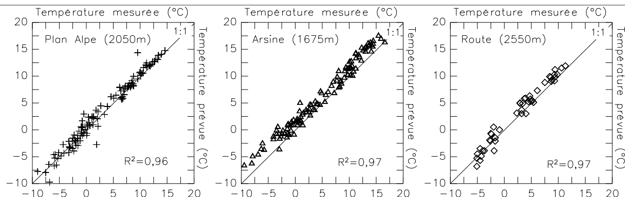
Figure II-19 : Relation entre les températures moyennes mensuelles mesurées aux stations du Plan de l'Alpe (2050m), d'Arsine (1675m) et de la Route (2550m) et les températures mensuelles moyennes extrapolées à partir des longues séries (1961-1990) de Météo France (cf. fig. III-13). Données Météo France et IGA. Relationship between mean monthly air temperatures measured at Plan de l'Alpe, Arsine and Route stations and extrapolated values from the long Météo France series.
