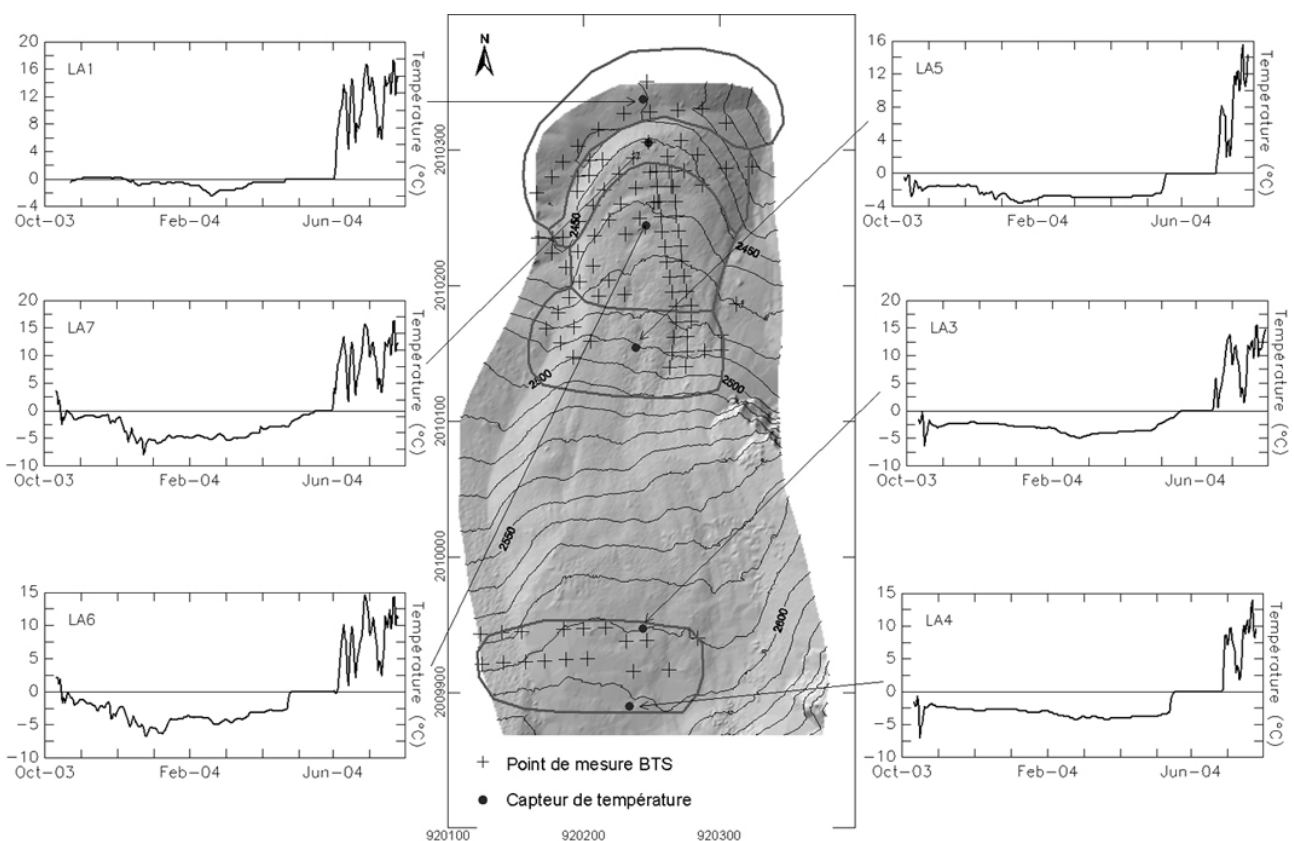
Figure IV-33 : Délimitation des secteurs homogènes (trait rouge) pour l'extrapolation des températures à la surface de RGL1 durant l'hiver 2003-2004. La localisation des points BTS (croix), celle des capteurs de température (point bleu), ainsi que l'évolution de cette dernière sont également représentées Delimitation of the homogeneous areas (red curve) for the ground surface temperature extrapolation at RGL1 during winter 2003-2004. BTS points, loggers' location and temperature records are also plotted.
