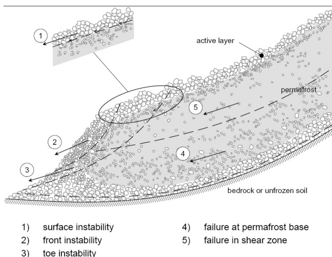
Figure IX-14 : Différents types d'instabilités probables au sein d'un glacier rocheux actif. Tiré de Arenson [2002]. Different types of probable instabilities within an active rockglacier.
