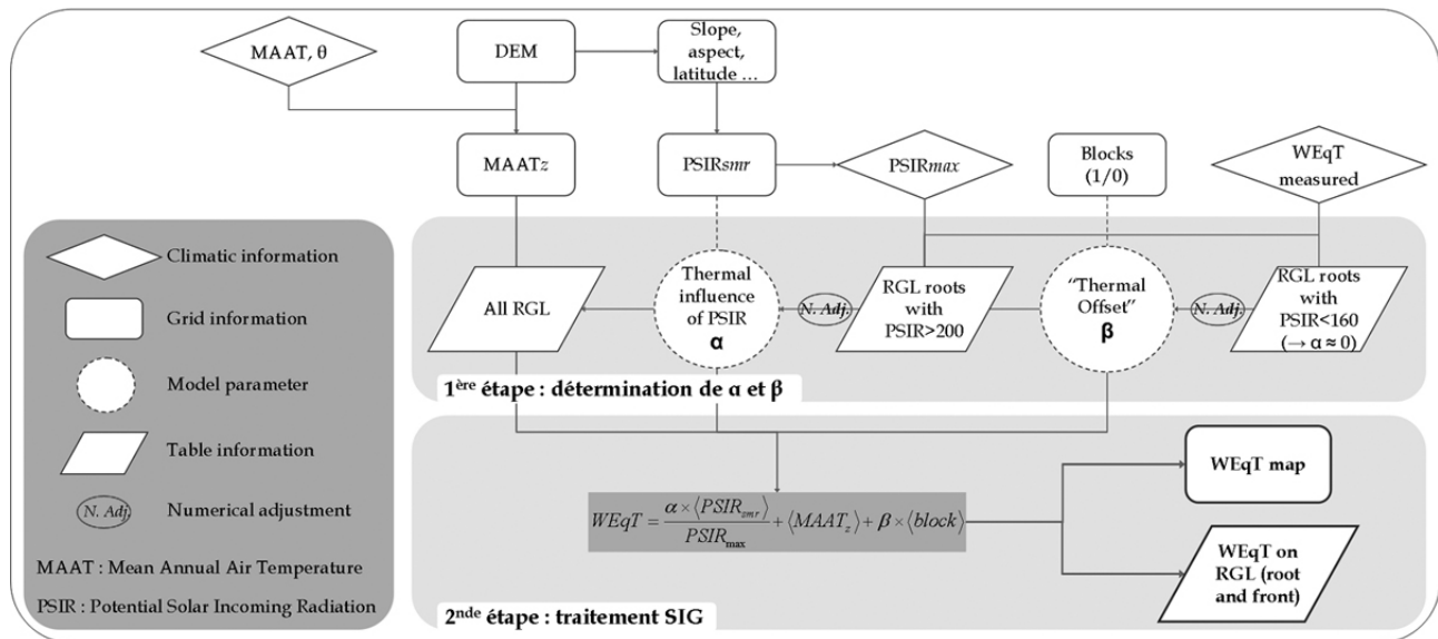
Figure VI-10 : Structure conceptuelle du modèle de spatialisation de la WEqT et description des étapes de calculs de la WEqT et de la cartographie associée (voir le texte pour la signification des termes). Source : Bodin et al. [2006], modifié. Conceptual framework of the model of WEqT spatialisation and description of the procedure to compute WEqT.
