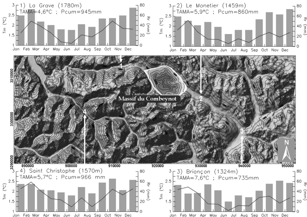
Figure II-13 : Ecart-type des températures et des précipitations mensuelles des quatre stations du réseau Météo France dans le secteur Oisans-Briançonnais (période 1961-1990, exceptées La Grave (1960-1988) et Saint Christophe (1964-2006), cf. tableau 2; MNA SRTM 100m, coord. Lambert 3 en m). Standard-deviation values of temperatures and precipitations of the 4 Météo France stations in the Oisans-Briançonnais area (1961-1990 period, except for La Grave, 1960-1988 and Saint Christophe, 1964-2006).
