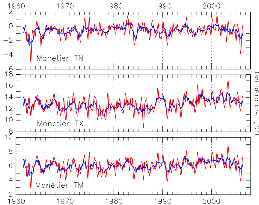
Figure II-29 : Résultats de la décomposition saisonnière des températures mensuelles minimales, maximales et moyennes de 1961 à 2006 enregistrées à la station de Monêtier. Données Météo France. Results of the seasonal decomposition of the minimal, maximal and mean monthly temperatures of Monêtier station.
