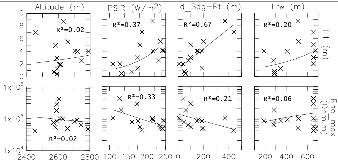
Figure IX-10 : Relation entre les paramètres géoélectriques (H1 : épaisseur de la couche active ; Rho_max : résistivité apparente maximale mesurée) déduits des sondages verticaux menés sur le massif du Combeynot et les variables morphométriques des sites prospectés (de gauche à droite : altitude ; insolation estivale potentielle ; distance entre le sondage et la racine de la forme ; ampleur de la paroi rocheuse en amont, cf. Ikeda [2004]). Modifié de Bodin et al. [2007a]. Relationship between geoelectrical parameters (H1: active layer thickness; Rho_max: maximal apparent resistivity) deduced from vertical soundings performed on the Combeynot Massif and the morphometric variables of the prospected sites (from left to right: elevation, potential solar radiation in summer, distance between the sounding and the root of the landform, length of the rockwall).
