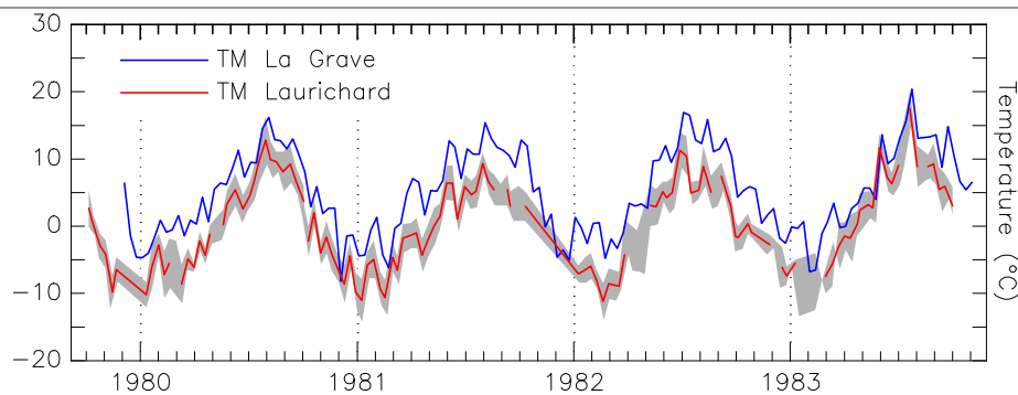
Figure IV-3 : Température moyenne (TM) décadaire de l'air à Laurichard (2450m ; courbe rouge ; en grisé, l'enveloppe TN/TX, température minimale / température maximale ; données [Francou, 1988]) et à La Grave (1780m ; courbe bleue, données Météo France). Decadal mean air temperature (TM) at Laurichard (2480m asl; red curve; in greyish the TN/TX envelope) and at La Grave (blue curve).
