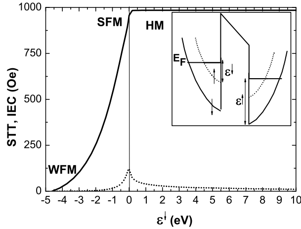
FIG. 3.19 : Couple de transfert de spin (trait plein) et partie dissipative du couplage d'échange intercouche (pointillés) en fonction du couplage J_{sd} . La ligne verticale indique la limite entre régime ferromagnétique (ferromagnétique faible -WFM- et ferromagnétique fort -SFM-) et régime demi-métallique (HM).
