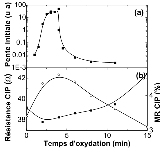
FIG. 2.41 : (a) Pente initiale du signal EHE d'une multicouche Pt/Co/AlOx( t )/Pt, pour différents temps d'oxydation. Le champ est appliqué perpendiculairement au plan des couches. (b) Résistance et magnétorésistance CIP d'une vanne de spin miroir équivalente, Co/Cu/Co/AlOx( t ), pour différents temps d'oxydation. D'après [3].
