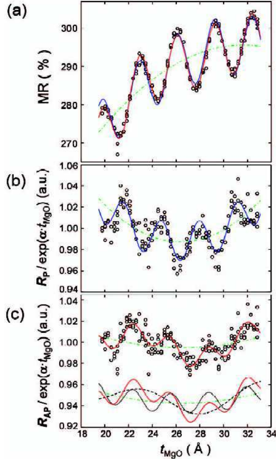
FIG. 1.30 : (a) TMR, (b) R^P / \exp(\alpha t_{\text{MgO}}) , (c) R^{AP} / \exp(\alpha t_{\text{MgO}}) . \alpha est un paramètre déduit des mesures de conductance. D'après [102].
