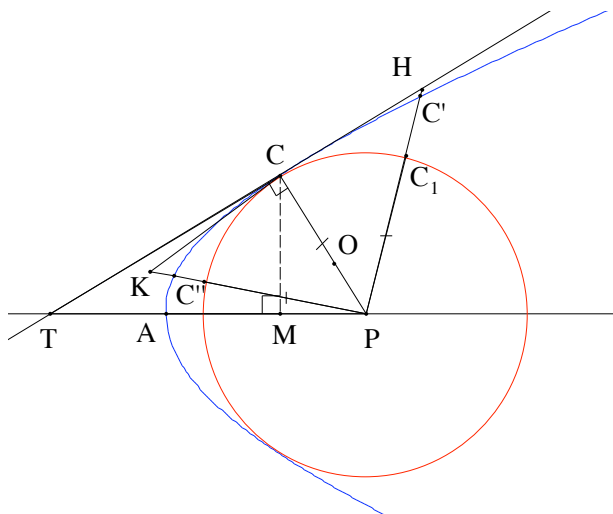
FIG. 6.2 – La droite minimum et la normale à une conique selon Apollonius et Descartes.
