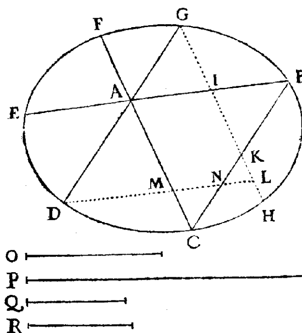
FIG. 13.1 – Geometria (1649), p. 296
