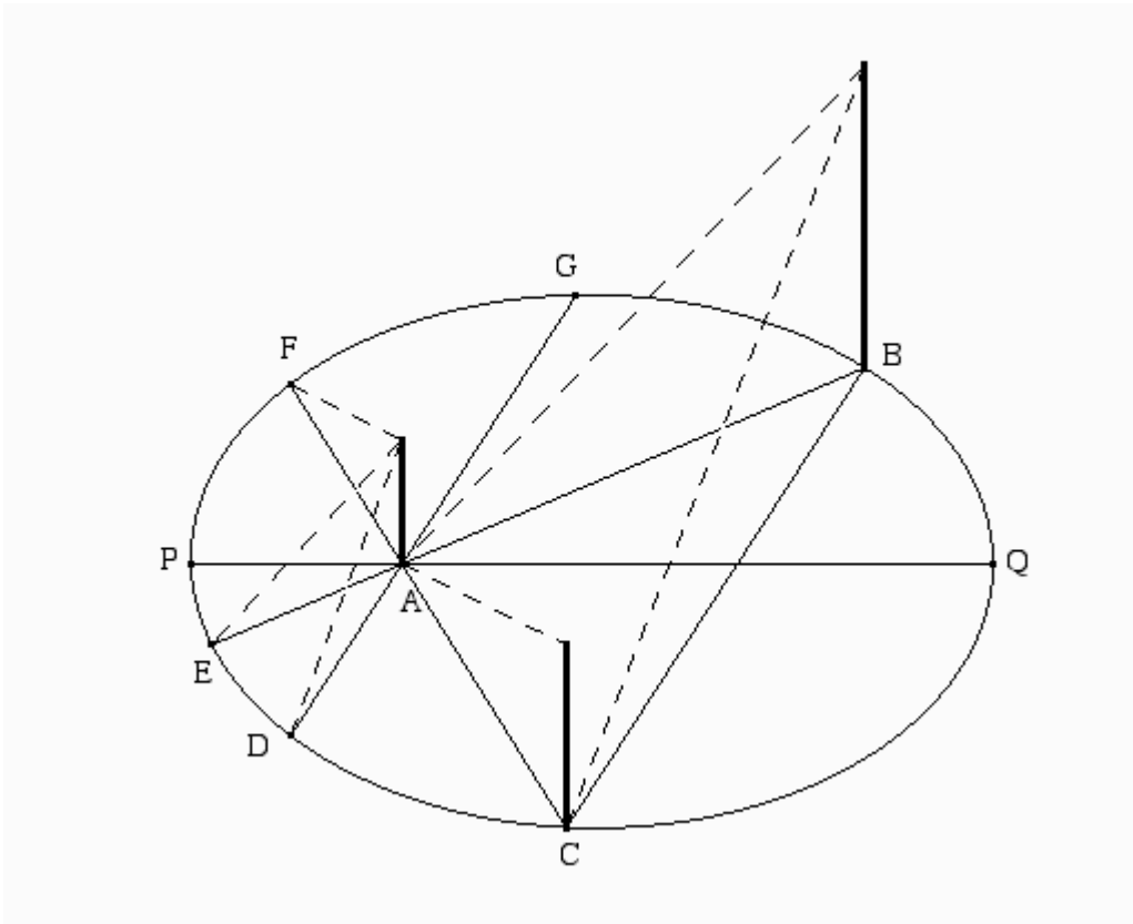
FIG. 12.5 – Le Problema astronomicum
