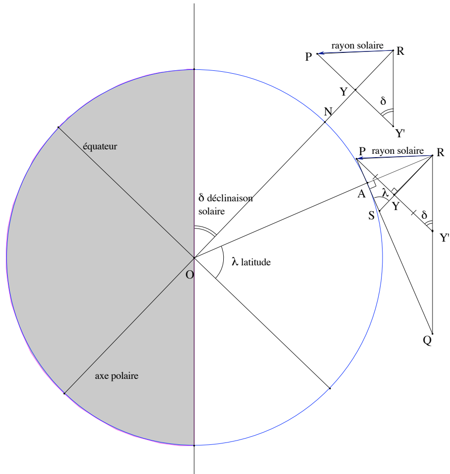
FIG. 12.1 – Le cône des rayons solaires (1)
