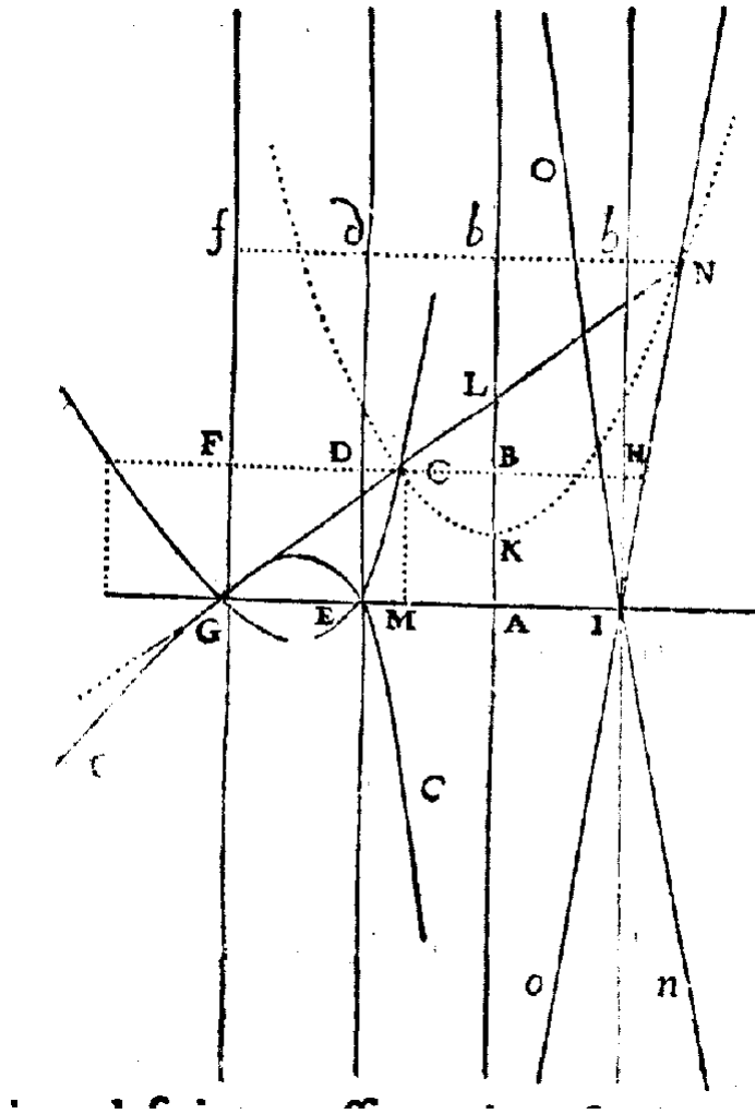
FIG. 2.10 – Géométrie (1637), p. 336.
