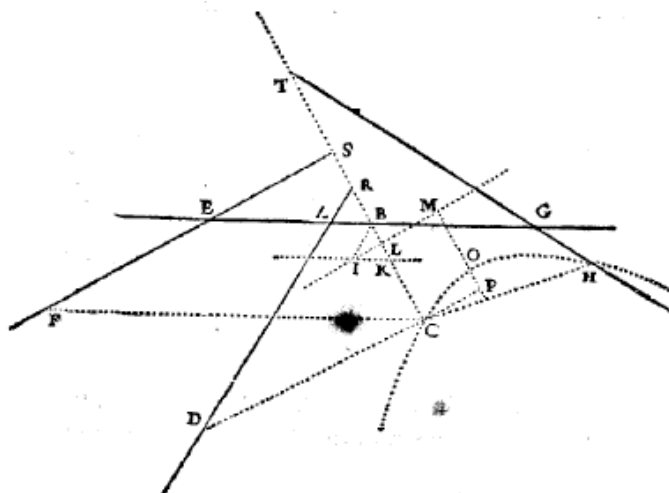
FIG. 4.2 – Géométrie (1637), p. 331
