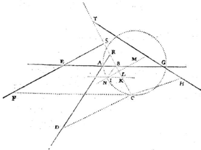
FIG. 2.7 – Géométrie (1637), p. 331
