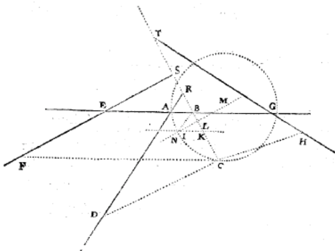
FIG. 4.3 – Géométrie (1637), p. 325
