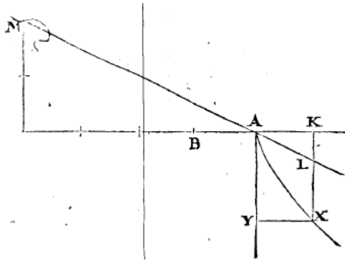
FIG. 4.1 – [Debeaune(1649), p. 132]
