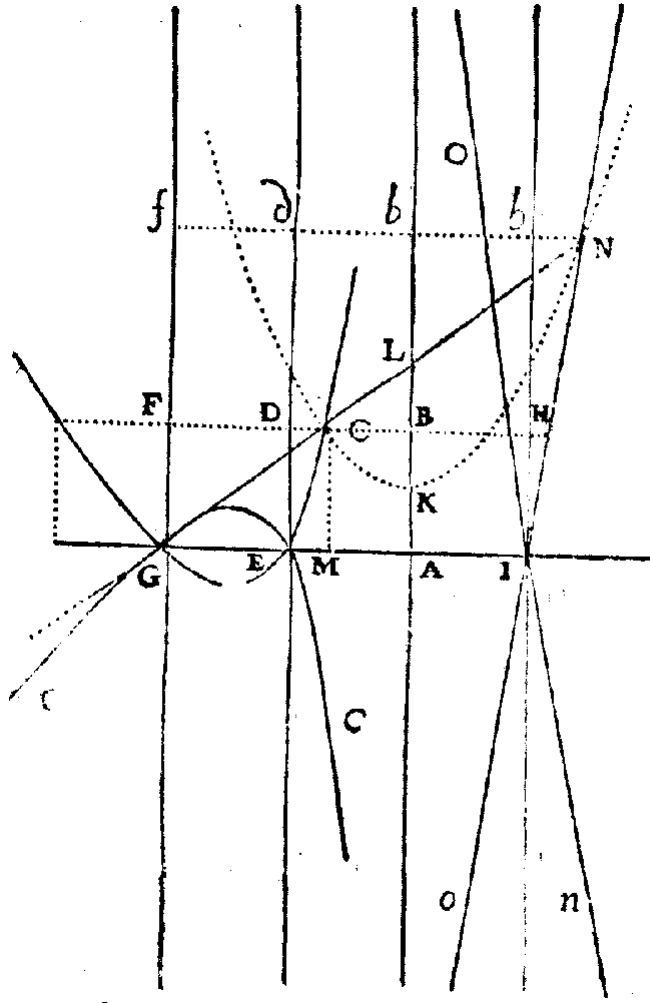
FIG. 2.10 – Géométrie (1637), p. 336.
