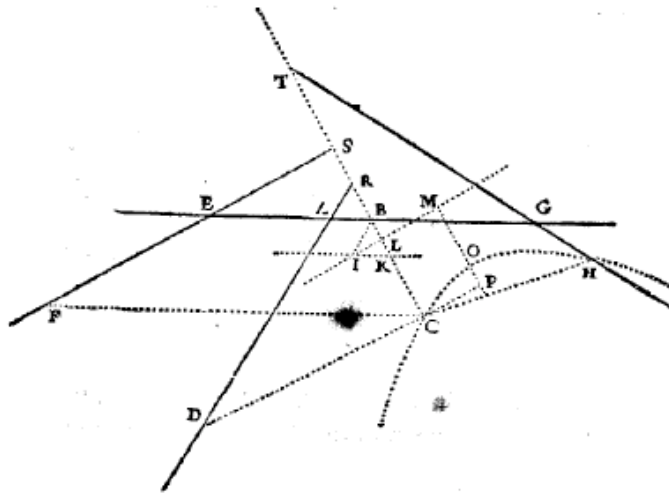
FIG. 4.2 – Géométrie (1637), p. 331
