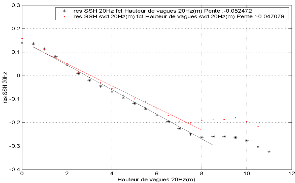
Figure 5-4 Résidu 20Hz en fonction de la hauteur de vagues 20 Hz. En astérisques noires ( \alpha \approx -5,25\% de SWH ). En points rouge avec la SVD ( \alpha_{\text{SVD}} \approx -4,71\% de \text{SWH}_{\text{SVD}} ) (99 demi orbites du cycle 61 de JASON)
