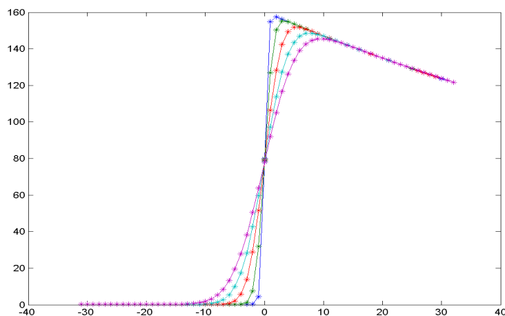
Figure 3-2 Modèle de Hayne pour 5 valeurs de SWH P_u = 160u , \tau = 0 , P_b = 1,3 et courbe bleue : SWH=0, verte : SWH = 2m, rouge : SWH = 4m, cyan : SWH = 6m, violette : SWH = 8m
