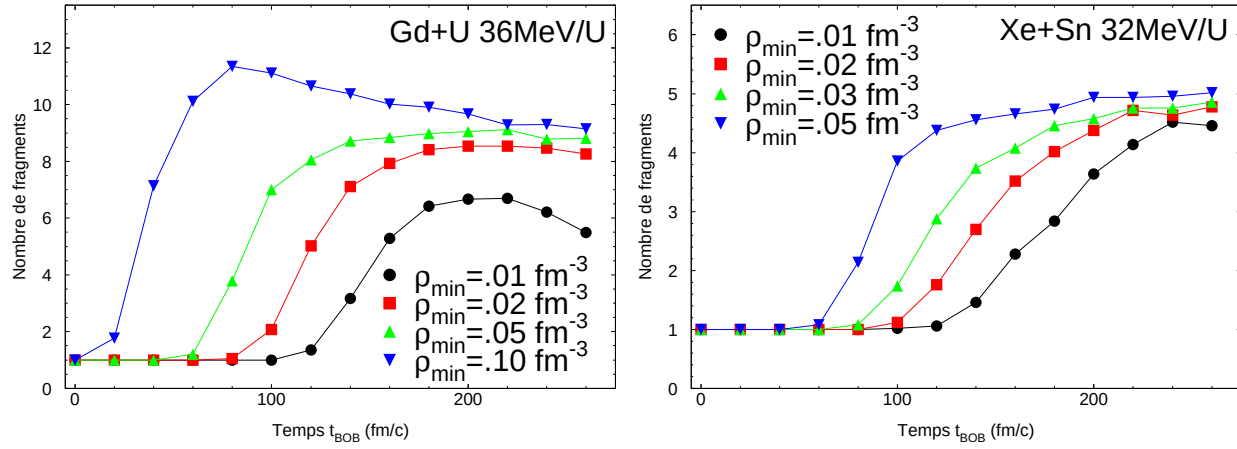
FIG. 12.8 – Multiplicité moyenne des fragments ( Z \geq 5 ) en fonction du temps depuis le début du calcul BoB pour les systèmes ^{155}Gd + ^{238}U et ^{129}Xe + ^{119}Sn . Le temps indiqué correspond au temps depuis le début du calcul BoB i.e. t_{BOB} = t_{BNV} - 40 fm/c.
