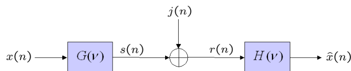
FIG. 4.5 – Chaîne de transmission monoporteuse.
