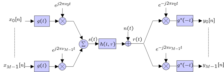
FIG. 2.1 – Chaîne de transmission multiporteuses.
