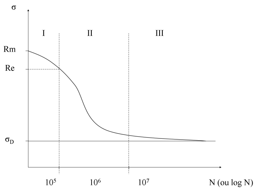
FIG. 2.2.4 – Courbe S-N.
