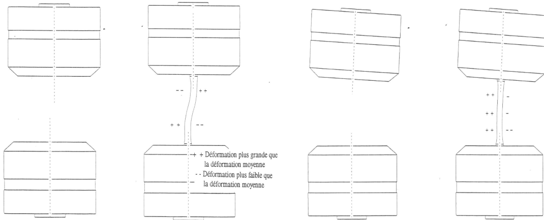
FIG. 1.3.3 – Déformation des éprouvettes dans les mors sans préreglage.
