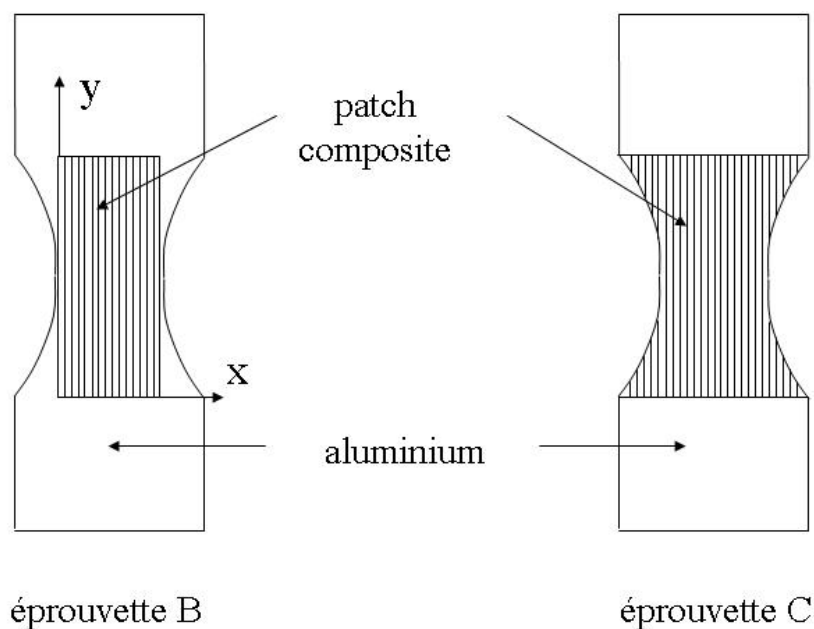
FIG. 1.4.3 – Deux types d'éprouvettes renforcées par patchs composites.
