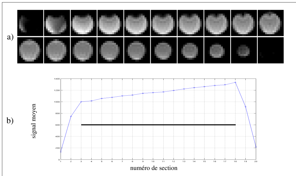
FIG. 4.10 Evaluation de la sélectivité spatiale de l'impulsion spectrospatiale : a) Volume acquis en EVI. b) Profil moyen du signal IRM selon la direction de partition, calculé dans une région d'intérêt de 25 voxels au centre de l'image. La ligne noire représente la largeur d'excitation théorique. La bande de transition représente environ 1 section pour 15 sections excitée. Le nombre de sections inutiles n'est plus que de 3 environ pour une vingtaine de coupes acquises. Paramètres d'acquisition :
