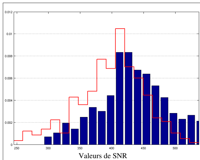
FIG. 5.4 Histogrammes décrivant les distributions spatiales du SNR dans une région d'intérêt, pour deux incréments de phase différents : 0^\circ (bleu), 45^\circ (rouge).
