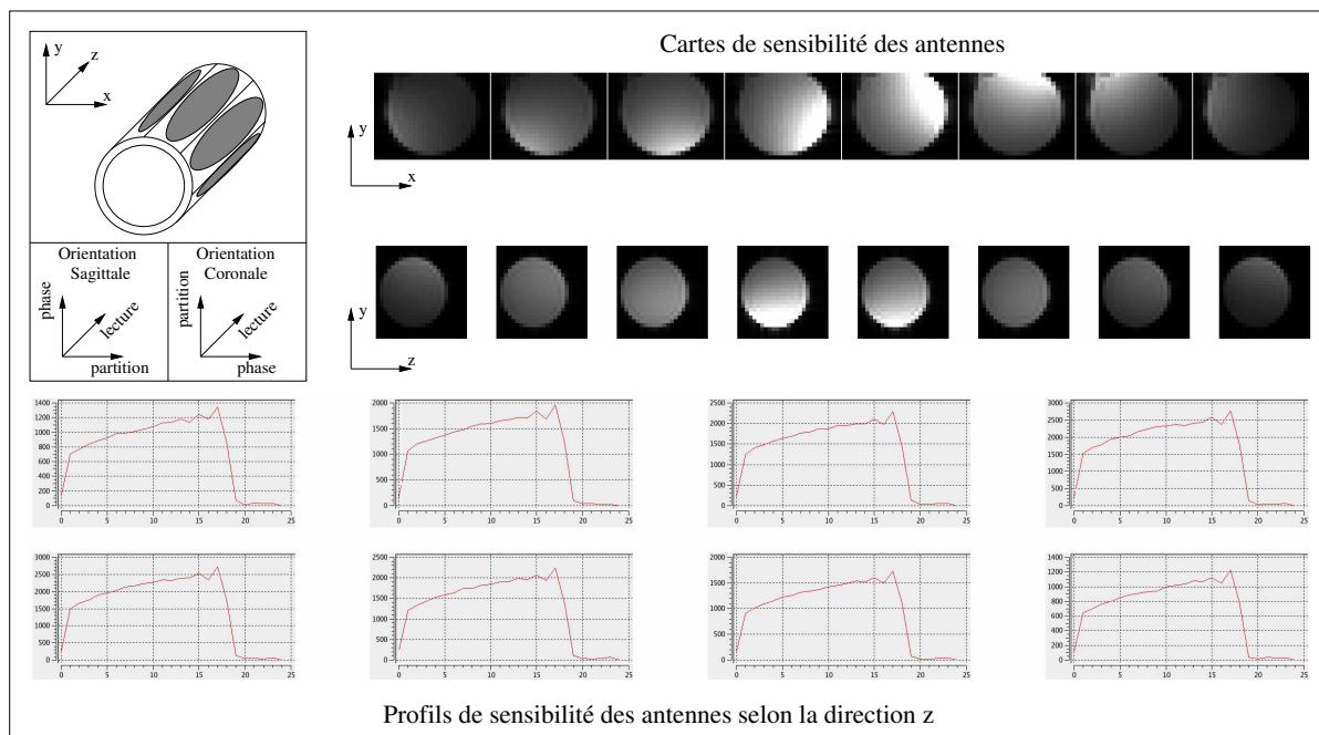
FIG. 7.7 A gauche : schéma de l'antenne tête à 8 canaux en réception, et description des deux orientations d'acquisitions utilisables en imagerie parallèle 2D. A droite : cartes de sensibilité des antennes présentées en sections (x,y) et en sections (z,y) . En bas : profils de sensibilité des 8 antennes selon la direction z , comme sur la carte de sensibilité montrant les sections (z,y) , tous les profils varient de la même manière, il est donc impossible d'appliquer la reconstruction parallèle selon cette direction.
