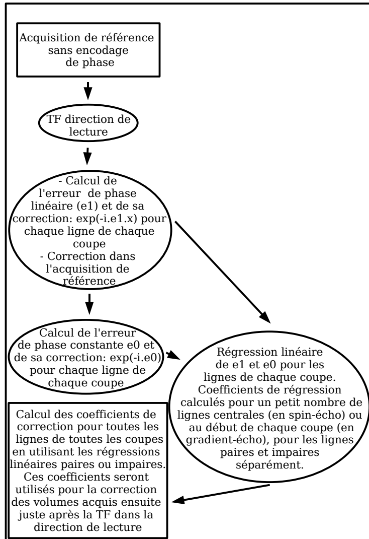
FIG. 1.21 Algorithme de correction de l'artéfact de "ghosting". Les données brutes de l'acquisition de référence subissent d'abord une transformation de Fourier 1D selon la direction de lecture. L'erreur de phase linéaire est ensuite estimée pour chaque ligne de l'acquisition de référence, ce qui correspond à une estimation du déplacement du centre de l'écho dans le plan de Fourier (théorème de décalage de la transformation de Fourier). Cette erreur est corrigée pour chaque ligne de l'acquisition de référence puis l'erreur de phase constante est estimée. Finalement, les coefficients de correction linéaires et constants sont modélisés linéairement (à partir de quelques lignes uniquement, dans la partie du plan de Fourier la moins exposée aux distorsions). Les coefficients ainsi corrigés seront utilisés pour la correction des données réelles. Une modélisation non linéaire est aussi possible.
