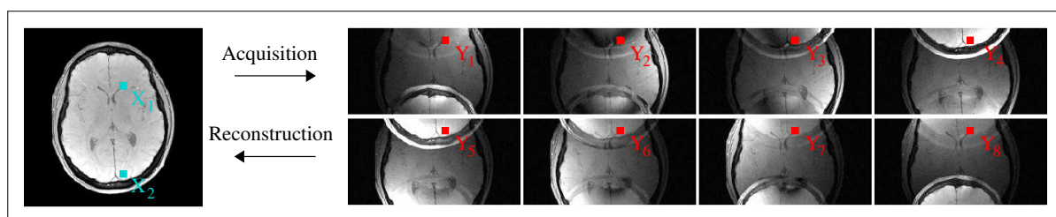
FIG. 7.1 Reconstruction parallèle SENSE dans le cas d'une acquisition 2D selon une grille cartésienne. À gauche : image reconstruite, à droite : images fournies par les différentes antennes (amplitude des images complexes reconstruites séparément par transformation de Fourier inverse 2D, à partir des données complexes).
