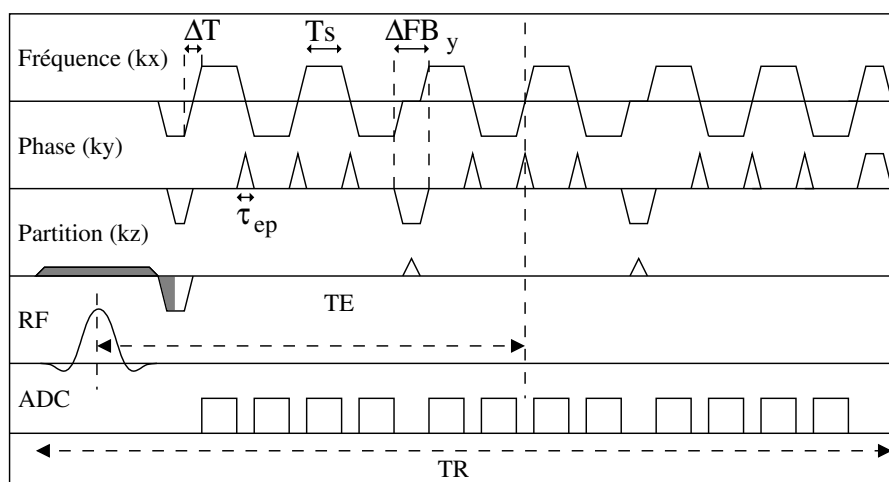
Chronogramme
