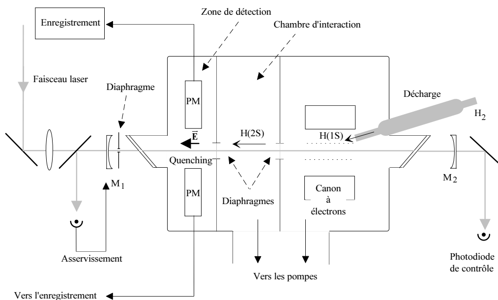
FIG. 1.2 – Schéma du jet atomique 2S.
