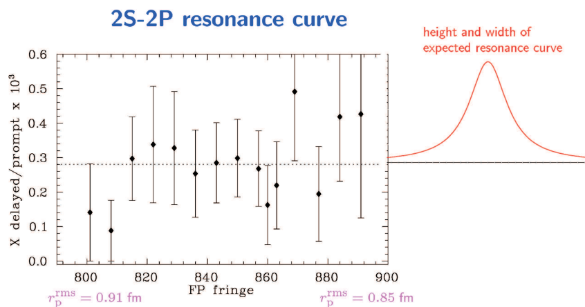
FIG. 1.10 – Evolution de la fluorescence 2P-1S en fonction de la fréquence laser. Le signal de résonance attendu est présenté à côté des points expérimentaux. Cette figure est extraite d'une présentation de F.Kottmann (Coimbra 2005).
