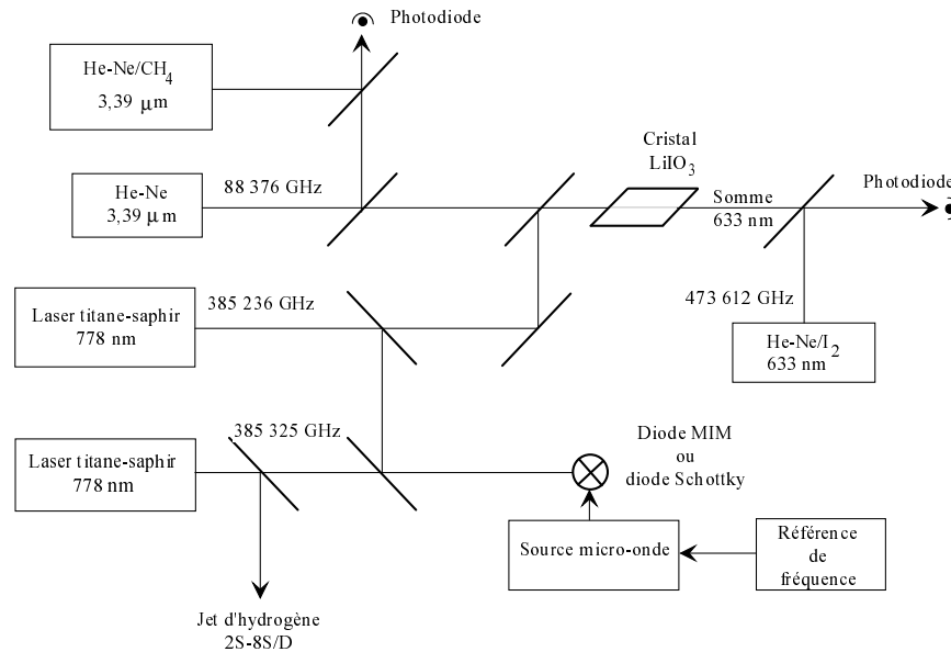
FIG. 1.3 – Schéma de la chaîne de fréquence utilisée en 1993
