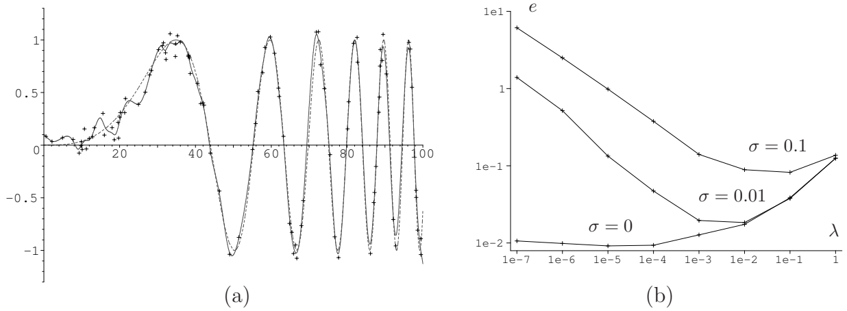
FIG. 4.6 : Reconstruction de la fonction s(t) = \sin\left(\left(\frac{t}{30}\right)^3\right) (en pointillés) à partir de 100 échantillons contaminés par un bruit blanc additif gaussien d'écart-type \sigma à des positions aléatoires localisées dans l'intervalle [0, 100] . (a) : spline uniforme cubique ayant ses nœuds aux entiers ( \varphi = \beta^3 , r = 2 , T = 1 ) reconstruite à partir des données bruitées ( \sigma = 0.1 , \lambda = 0.1 ). (b) : erreur e = \left(\frac{1}{100} \int_0^{100} |s(t) - f_T(t)|^2 dt\right)^{1/2} en fonction du niveau de bruit \sigma et du paramètre \lambda , en échelle log-log.
