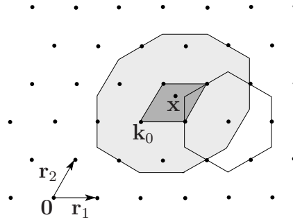
FIG. 3.15 : Pour évaluer f_T(\mathbf{x}) à un certain point \mathbf{x} , à l'aide de la formule (3.112), il faut connaître les sites \mathbf{R}\mathbf{k} tels que \varphi(\mathbf{x} - \mathbf{R}\mathbf{k}) \neq 0 . Ils appartiennent au domaine gris clair obtenu par dilatation morphologique du losange contenant \mathbf{x} (en gris foncé) avec le support de \varphi comme élément structurant. Dans cet exemple, \varphi = \eta_2 , dont le support est l'hexagone représenté. Celui-ci est ici centré en l'un des 8 sites susceptibles de contribuer à la valeur de f_T(\mathbf{x}) , si l'on sait seulement de \mathbf{x} qu'il est dans le losange.
