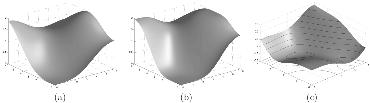
FIG. 3.12 : Noyaux d'erreur pour la reconstruction hex-spline d'ordre 2 : (a) E_{\text{int}}(\boldsymbol{\omega}) associé à l'interpolation (donc sans préfiltre car \eta_2 est interpolante); (b) E(\boldsymbol{\omega}) pour la quasi-interpolation avec le filtre RIF du tableau 3.2; (c) la différence E - E_{\text{int}} montrant clairement l'avantage de la quasi-interpolation, qui offre une meilleure qualité d'approximation dans toute la bande de Nyquist.
