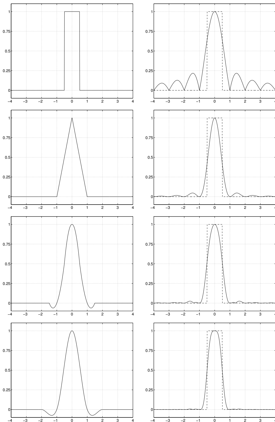
FIG. 2.4 : De haut en bas : générateurs polynomiaux par morceaux \varphi(t) de degrés 0,1,2,3 (à gauche) et leurs spectres respectifs \hat{\varphi}(\omega) (à droite, avec comme variable la fréquence \nu = \omega/2\pi ).
