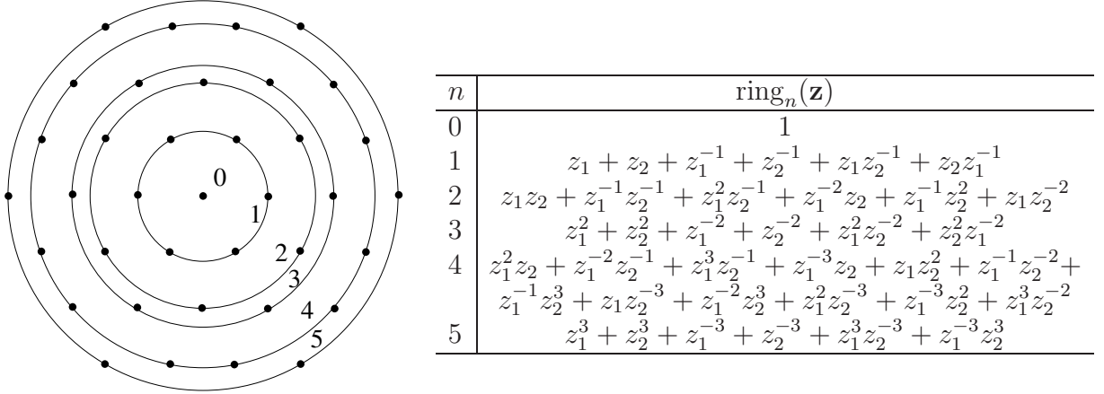
FIG. 3.4 : On définit des anneaux (à gauche) collectant les sites du treillis \Lambda_{\text{hex}} à égale distance de l'origine. On peut ainsi exprimer aisément, et sous une forme compacte, les transformées en \mathbf{z} de filtres discrets isotropes, au moyen des fonctions \text{ring}_n(\mathbf{z}) (à droite), qui sont les transformées en \mathbf{z} de filtres concentriques dont les coefficients sont 1 sur le n -ième anneau, et 0 ailleurs.
