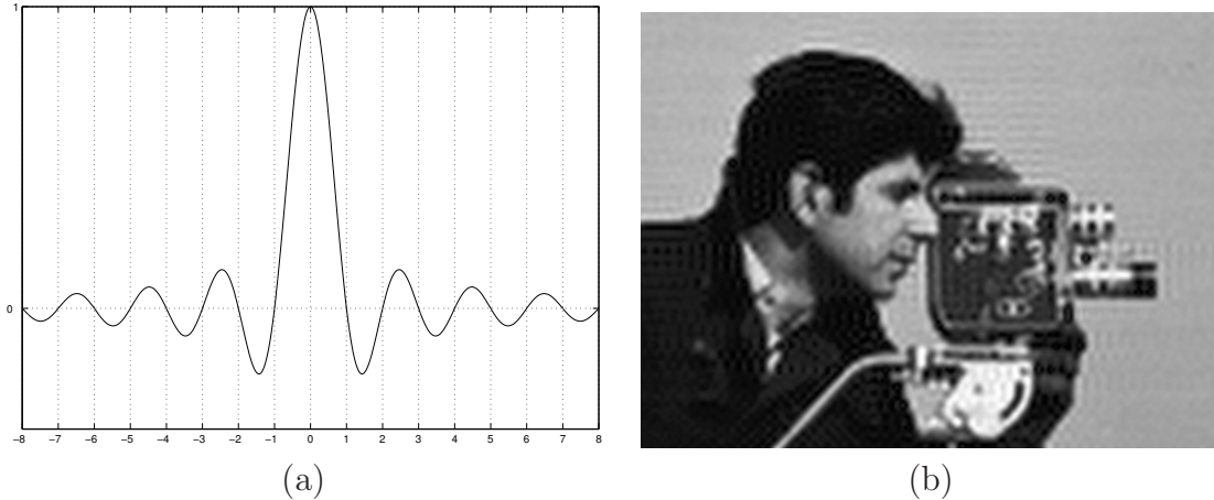
FIG. 2.2 : (a) : la fonction \text{sinc}(\pi t) et (b) : interpolation sinus cardinal f_T(\mathbf{x}) de l'image (v[\mathbf{k}]) (portion de l'image Camera ).
