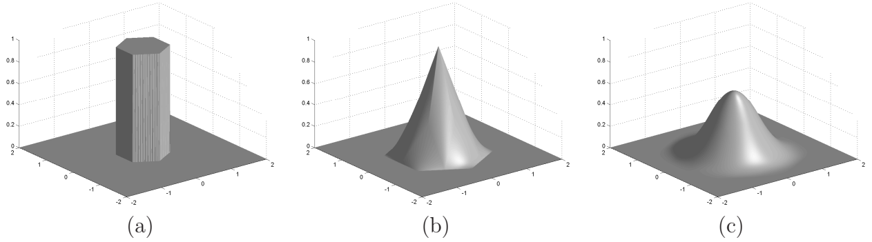
FIG. 3.3 : Hex-splines (a) \eta_1(\mathbf{x}) , (b) \eta_2(\mathbf{x}) , (c) \eta_3(\mathbf{x}) déployées sur le treillis hexagonal \Lambda_{\text{hex}} .
