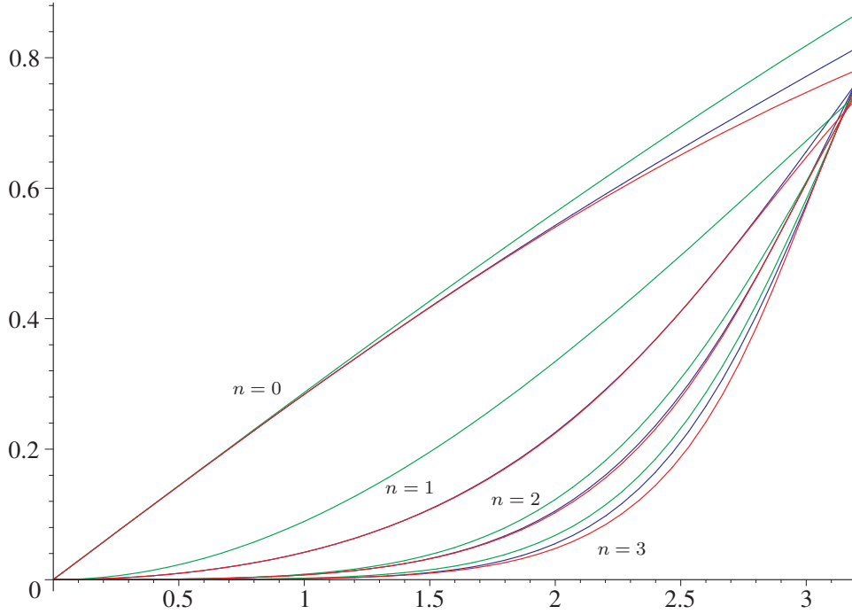
FIG. 2.12 : Noyaux d'erreur associés à la projection orthogonale (en rouge), l'interpolation (en vert), et la quasi-interpolation (en bleu) spline de degré n = 0 à 3.
