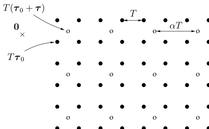
FIG. 5.1 : En redimensionnant une image définie sur le treillis noir \Lambda_{T,\tau_0} avec un facteur \alpha = 2 et un offset \boldsymbol{\tau} = (\frac{1}{2}, \frac{1}{2}) , on obtient une image localisée sur le treillis blanc \Lambda_{\alpha T, (\tau_0 + \boldsymbol{\tau})/\alpha} . Inversement, on passe d'une image localisée sur le treillis blanc à une autre localisée sur le treillis noir par redimensionnement de facteur \frac{1}{2} , d'offset (-\frac{1}{4}, -\frac{1}{4}) .
