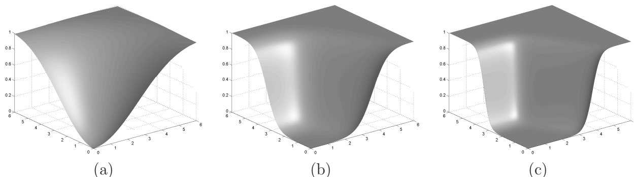
FIG. 3.11 : Noyaux d'erreur E_{\min}(\boldsymbol{\omega}) associés à la projection orthogonale spline sur le treillis hexagonal. (a) \varphi = \eta_1 , (b) \varphi = \eta_2 , (c) \varphi = \chi_4 . Lorsque l'ordre d'approximation de \varphi augmente, le noyau d'erreur s'annule de plus en plus dans la région de Nyquist, de forme hexagonale.
