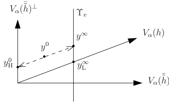
FIG. 7.3 : L'induction oblique en termes de projections.
