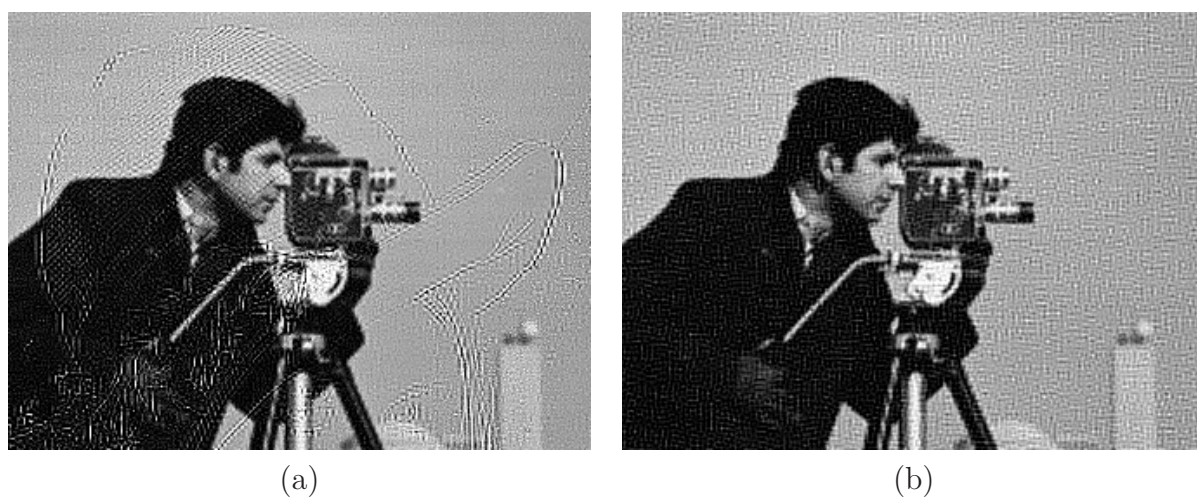
FIG. 7.2 : L'ensemble induit contient une infinité d'images, pouvant être assez éloignées de l'image idéale y^{id} . Il va nous falloir trouver une « bonne » méthode inductrice, en un sens à préciser, fournissant une image inductrice y^0 qui, après induction, soit visuellement satisfaisante. Un choix naïf d'image inductrice donne des résultats peu convaincants. Par exemple, si l'image v est Camera et que l'on considère Lena comme inductrice, l'image induite contient bien le cameraman, mais avec les contours de Lena en filigrane (a). En (b), l'image induite en prenant comme inductrice une image de bruit : le cameraman est bien présent, mais avec du bruit en surimpression.
