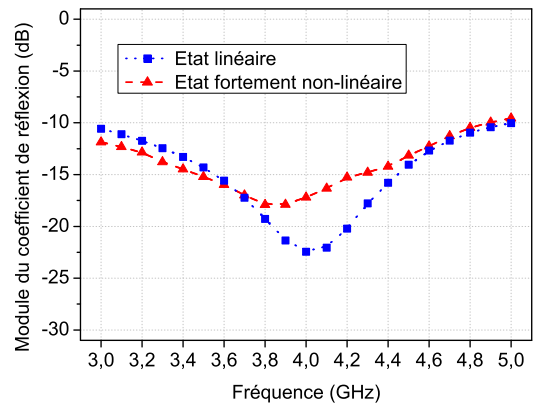
FIG. 3.44 – Paramètre S22 en régime linéaire et fortement non-linéaire pour le second LNA à base de BFY420.
