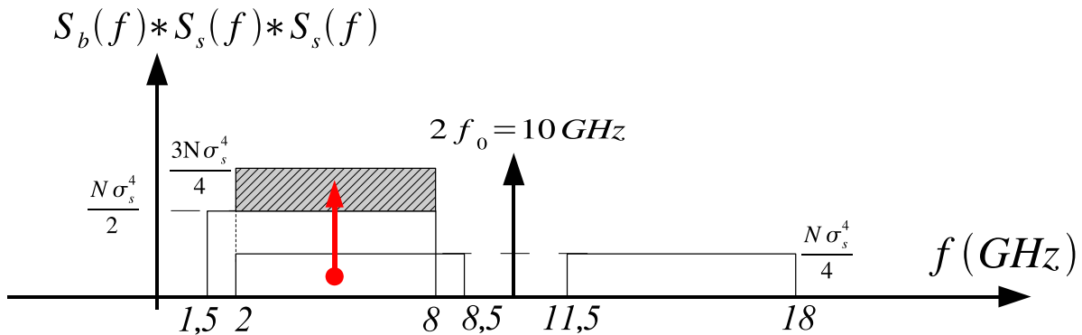
FIG. 3.46 – DSP en BLU de S_b(f) * S_s(f) * S_s(f) pour f_0=5 GHz.
