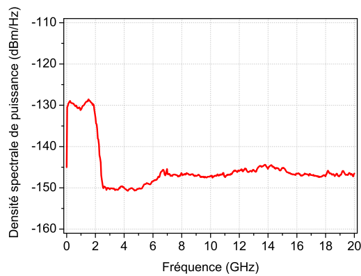
FIG. 1.14 – Bruit de type passe bas, injecté à l’entrée du DST.
