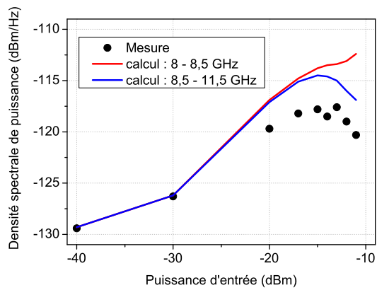
FIG. 1.47 – Comparaison calcul/mesure pour la bande 8 - 11,5 GHz.
