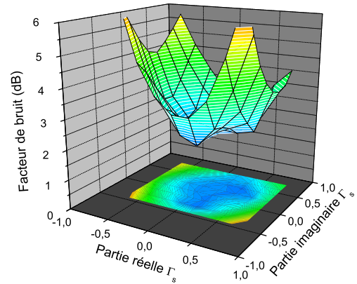
FIG. 2.34 – Facteurs de bruit du BFY420 à 4 GHz en fonction des impédances de source, régime fortement non-linéaire. Bleu : faible F, rouge : fort F.
