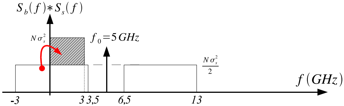
FIG. 3.45 – DSP en BLU de S_b(f) * S_s(f) pour f_0=5 GHz.
