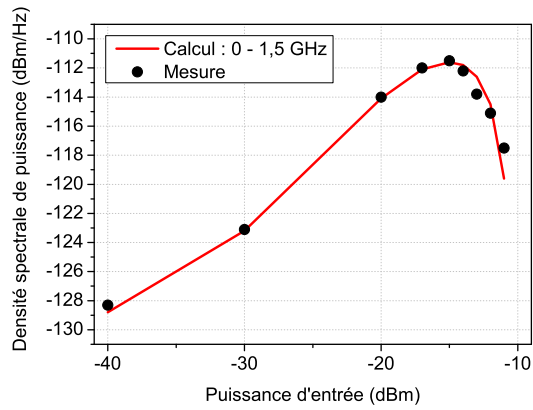
FIG. 1.45 – Comparaison calcul/mesure pour la bande 0 - 1,5 GHz.
