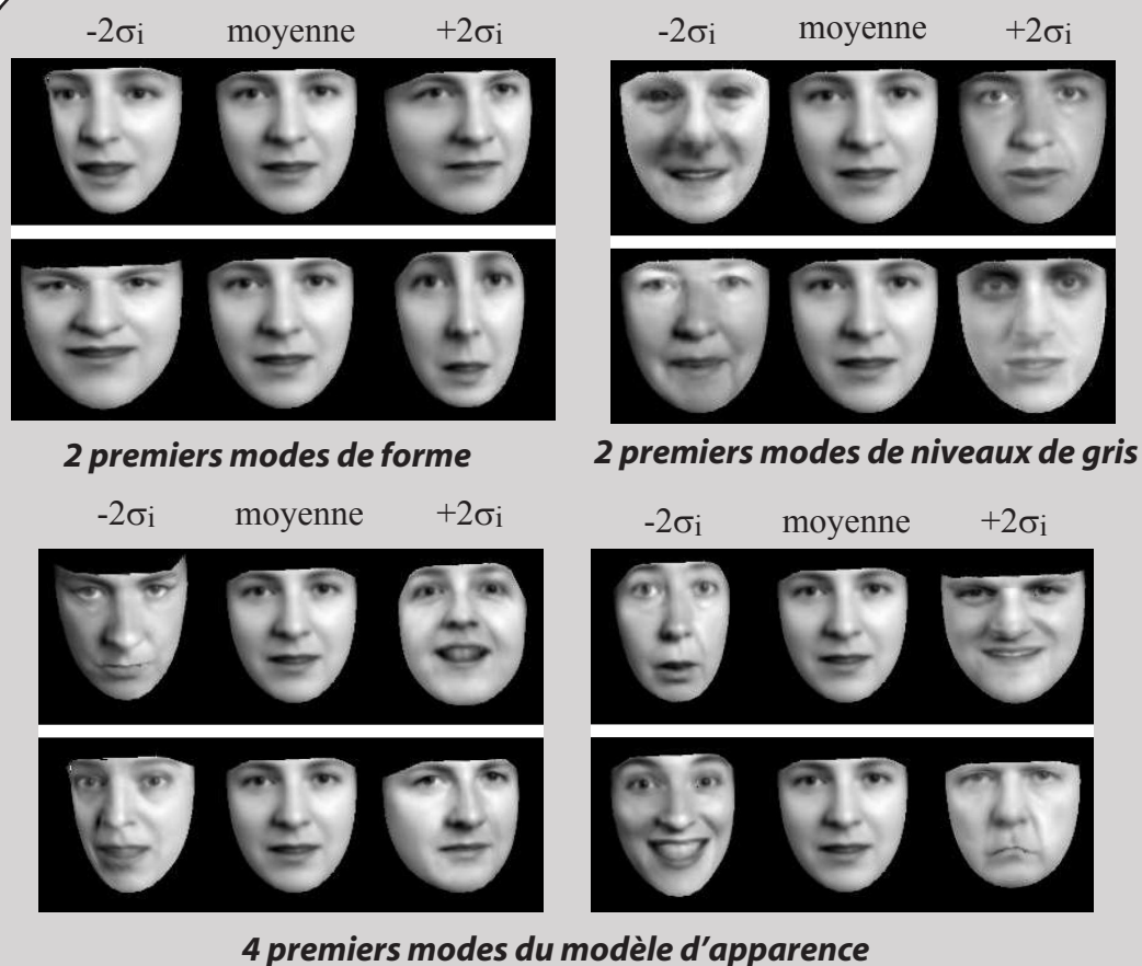
Figure 1.15 Premiers modes de variations pour les différents modèles d'un AAM, [Cootes, 1998].
