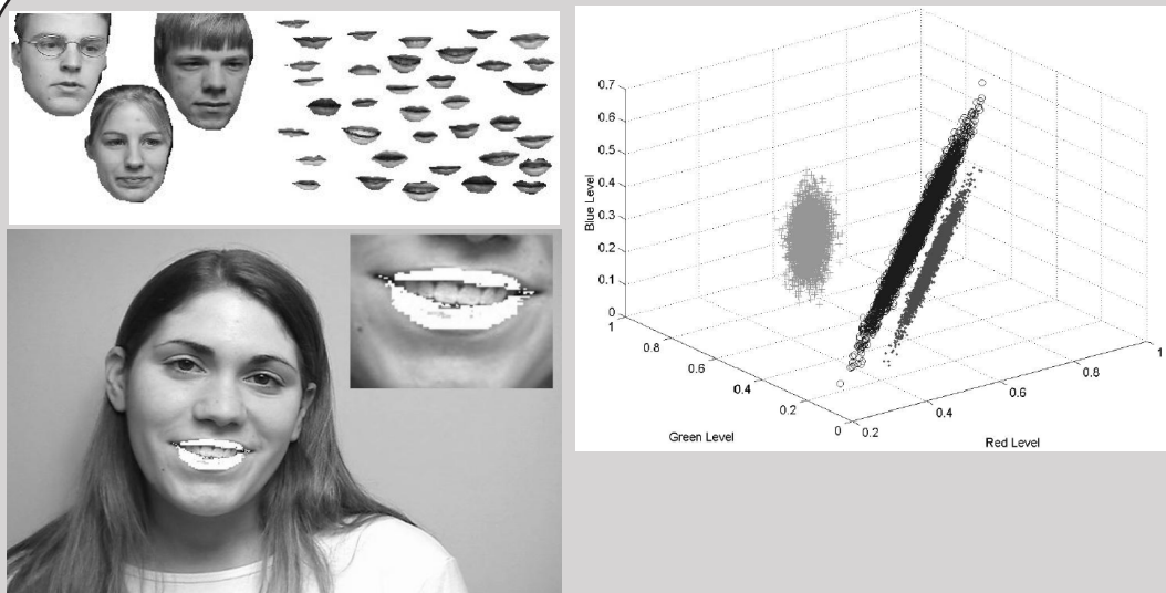
Figure 1.7 : Système de détection de lèvre par modélisation gaussienne des distributions des valeurs de peau, lèvres et fond dans l'espace RVB, d'après [Patterson, 2002].
