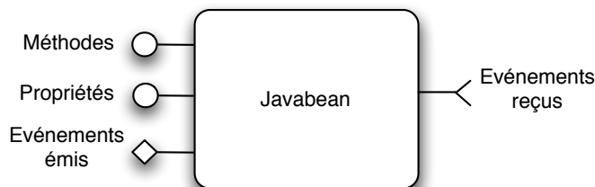
FIG. 2.9 : Structure d'un composant Javabeans
