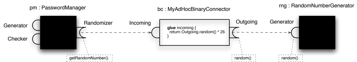
FIG. 3.12 : Utilisation d'un connecteur binaire
