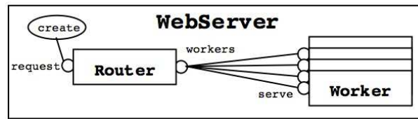
FIG. 2.19 : Architecture d'un composite WEBSERVER en ArchJava
