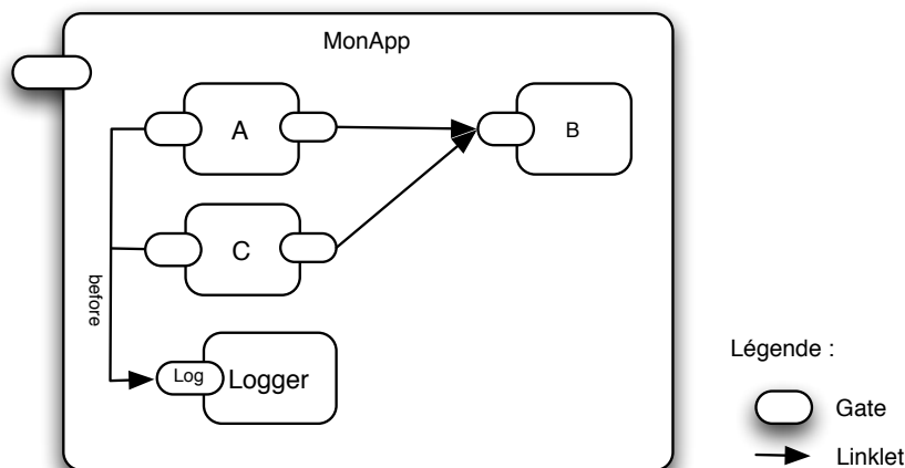
FIG. 4.4 : Schéma général du modèle FuseJ
