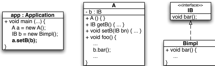
FIG. 2.2 : Couplage faible et explicite entre deux classes d'objets
