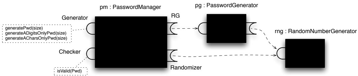
FIG. 3.16 : Exemple d'architecture équivalente sans composite
