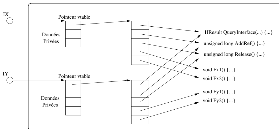
FIG. 2.6 : Organisation interne d'un objet COM ayant deux interfaces fournies IX et IY
