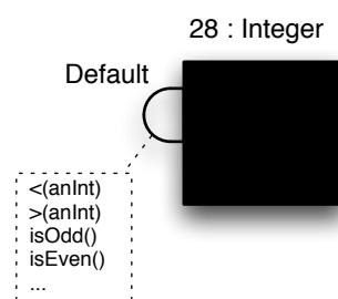
FIG. 3.4 : Un entier vu comme un composant en SCL
