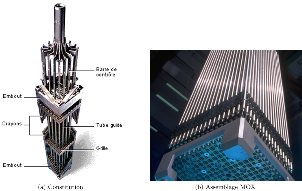
FIG. 1.4: Assemblage combustible d'un réacteur à eau sous pression.
