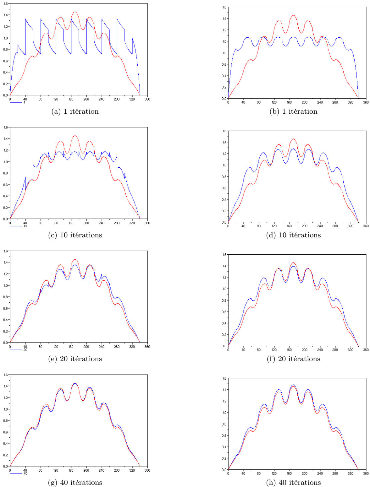
FIG. 7.3: Représentation des flux au cours des itérations. A droite la convergence du calcul direct, à gauche la convergence de la méthode IDD avec 17 sous-domaines.
