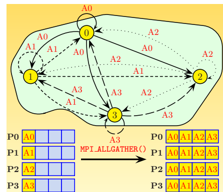
(d) MPI_Allgather
