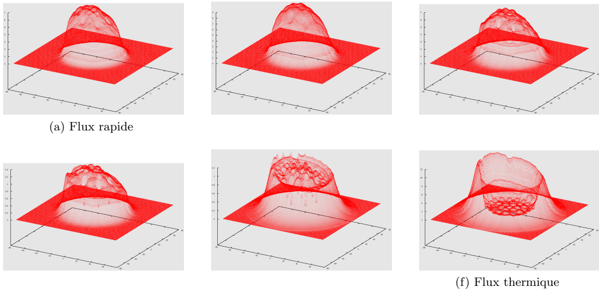
FIG. 2.9: Représentations graphiques des flux du RJH en 2D pour un calcul à six groupes d'énergie.
