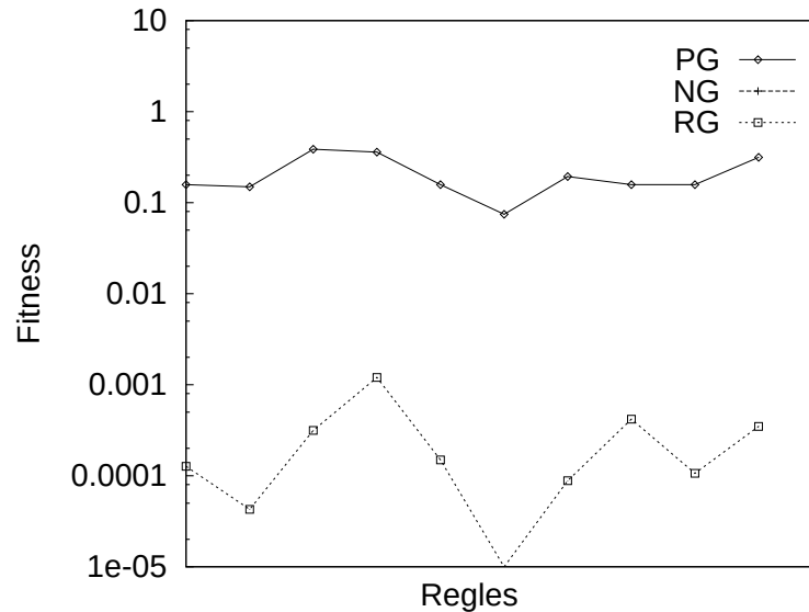
FIG. 8.1: Meilleures règles apprises sur le groupe PG et évaluées sur les groupes RG et NG
