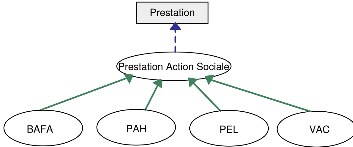
FIG. 7.2: Le sous-domaine « Prestation Action Sociale » dans une ontologie dédiée au contact allocataire
