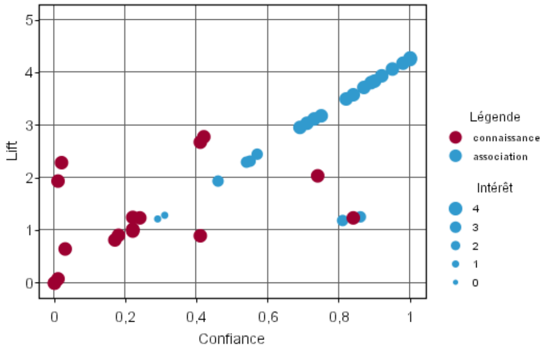
FIG. 8.10: Confiance et lift des connaissances exprimées par les experts en langage naturel (en rouge) et des règles qui leur sont associées (en bleu)
