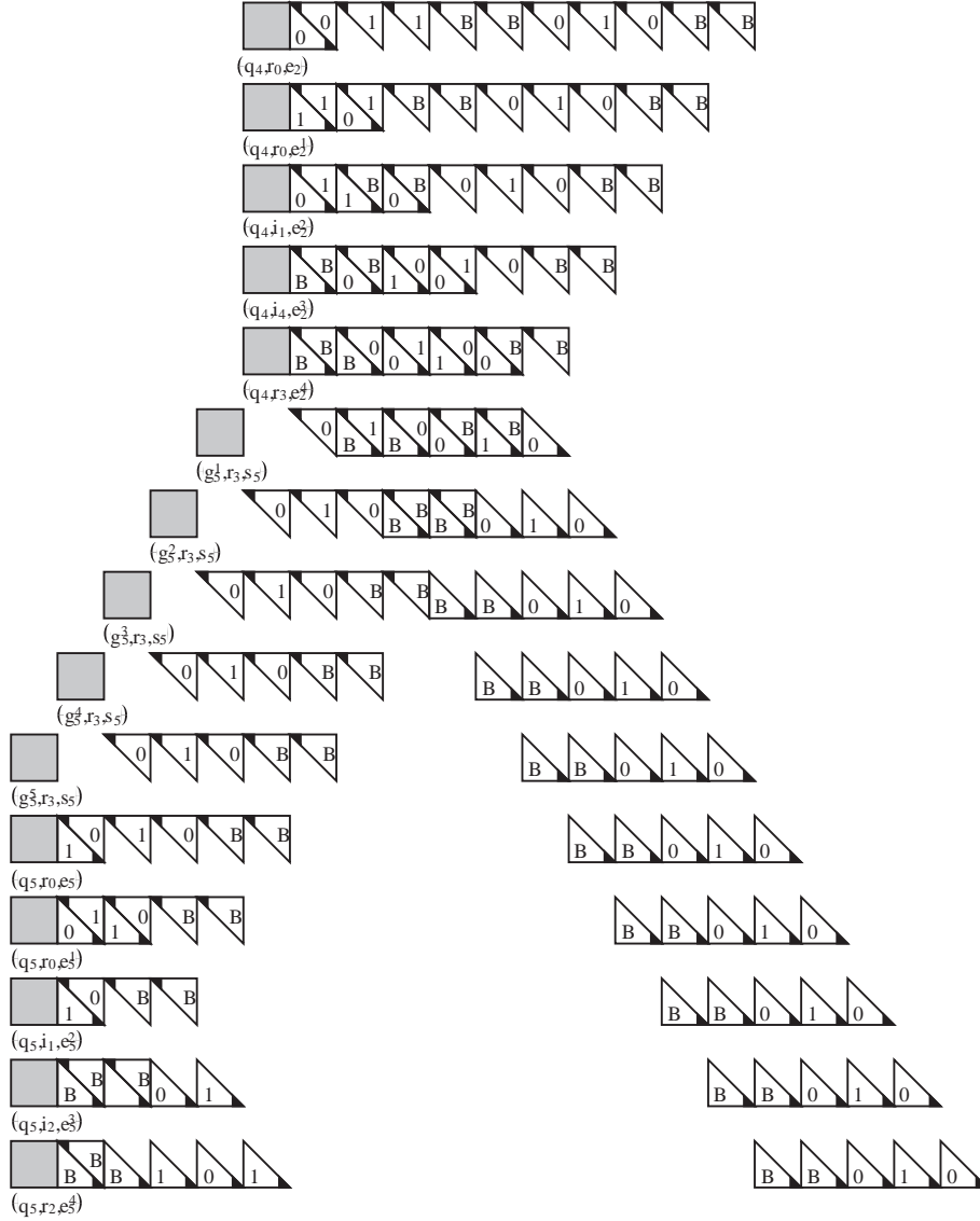
Fig. 7. Simulation du déplacement d'un processeur.
