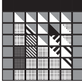
Fig. 3. Solution de Mazoyer à deux généraux.
