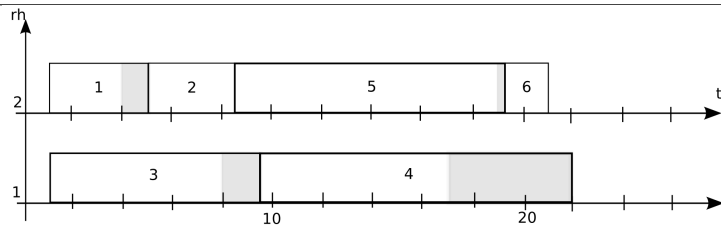
FIG. B.1 – Ordonnancement ECT-EDD en contexte de faible charge
