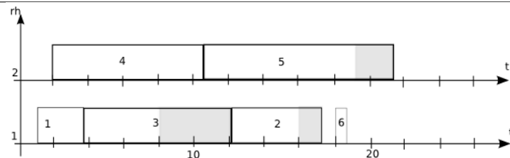
FIG. B.3 – Ordonnancement LPT-H-EDD en contexte de faible charge
