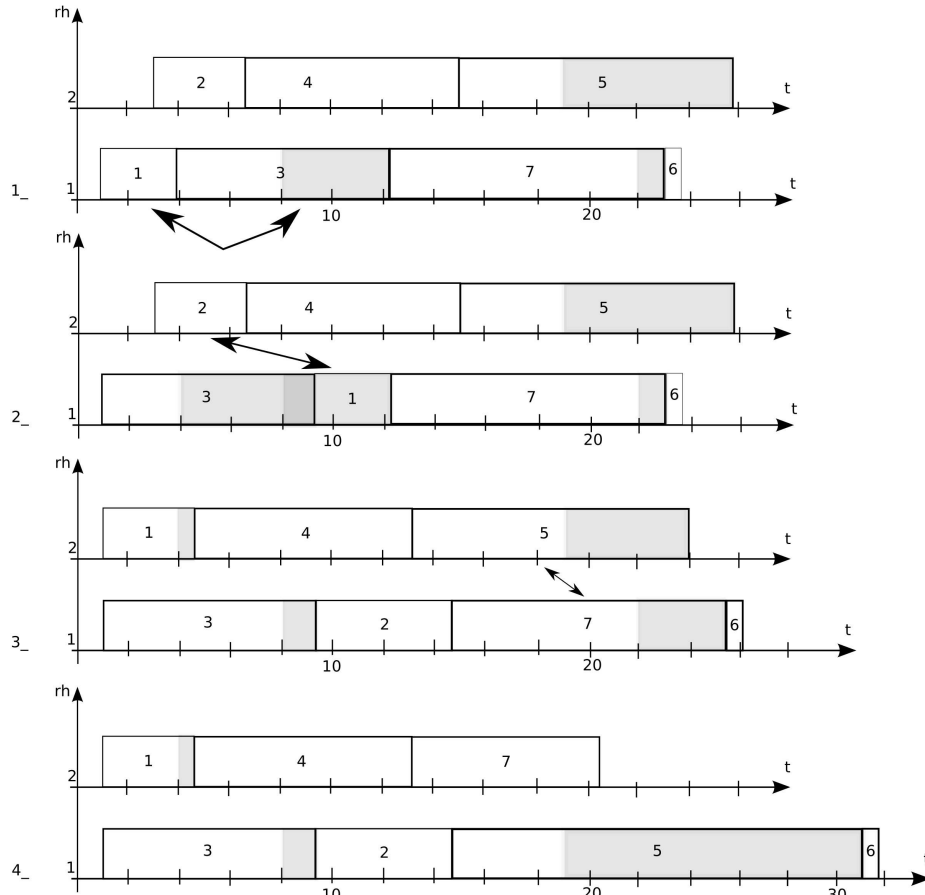
FIG. D.3 – Déroulement d'un saut
