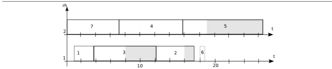
FIG. C.2 – Ordonnement courant après insertion
