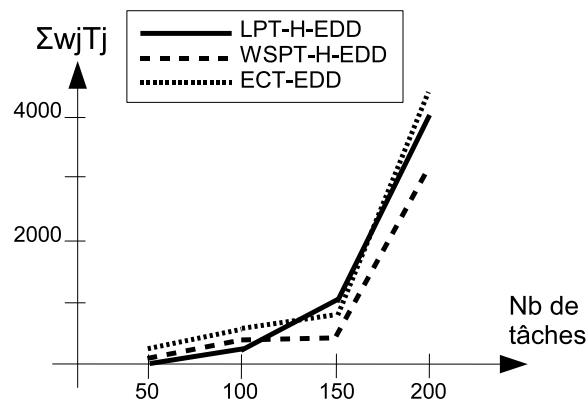
FIG. III.3 – Évolution de \sum w_j T_j
