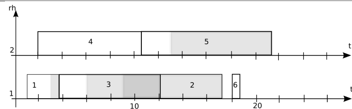
FIG. B.4 – Ordonnancement LPT-H-EDD en contexte de forte charge
