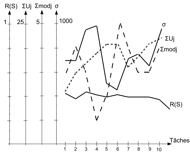
FIG. V.11 – Évolution des solutions de l'approche multi-critère
