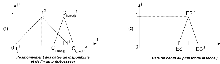
FIG. V.3 – Obtention de la date de début au plus tôt floue de la tâche j
