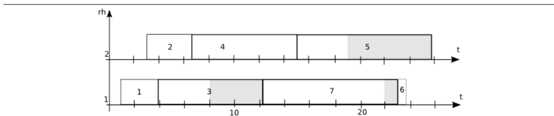
FIG. C.5 – Ordonnement réalisé avec l'heuristique LPT-H-EDD
