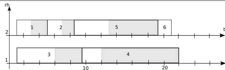
FIG. B.2 – Ordonnancement ECT-EDD en contexte de forte charge
