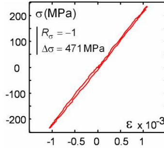
FIG. 3.33 – Exemple d'hystérésis mécanique
