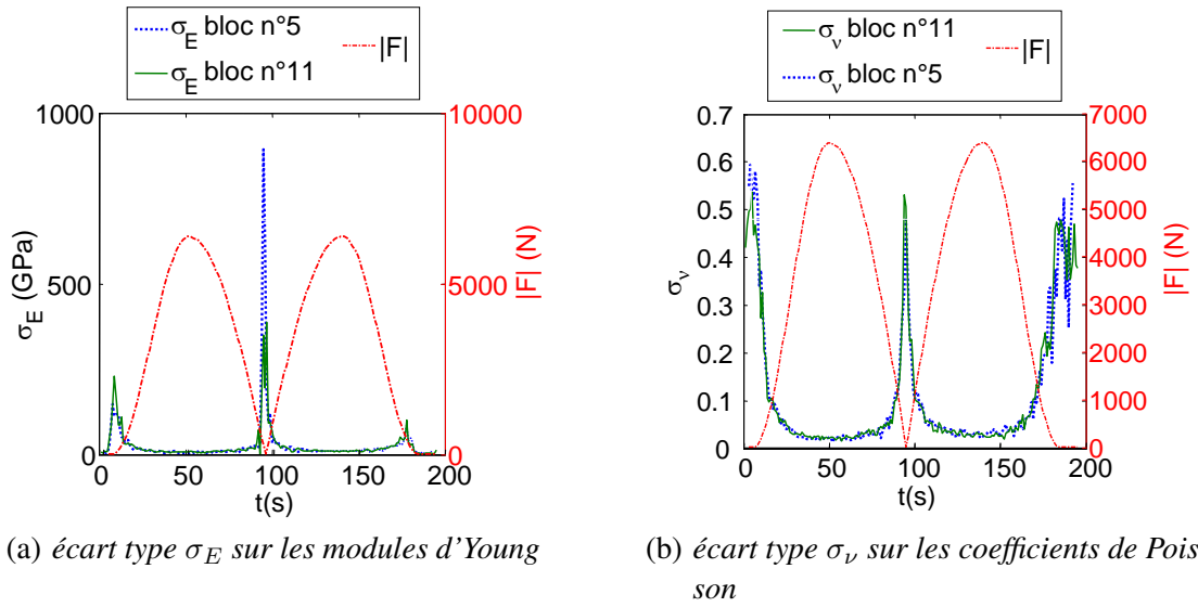
FIG. 3.37 – évolution des écarts types sur les paramètres identifiées au cours des cycles mécaniques associés aux blocs n°5 et n°11
