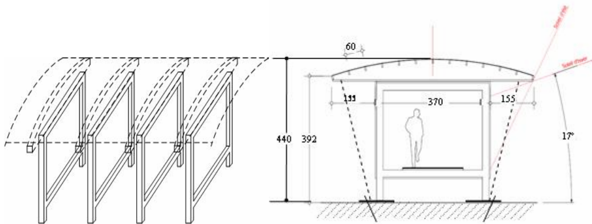
Figure 24 : Structure de type squelette de la cellule expérimentale (unité en cm)
