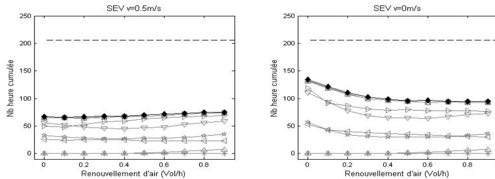
Figure 137 : Nombre d’heure de surchauffe en fonction du taux de renouvellement d’air pour les SENV et SEV sous trois régimes de convection (Nice, ép.: 1cm)
