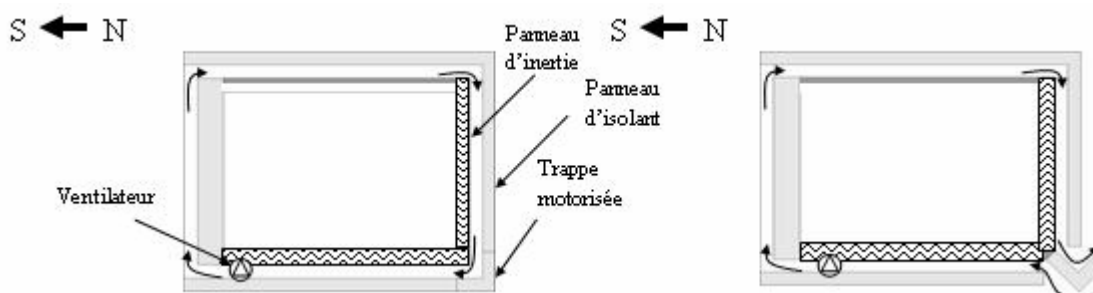
Figure 22 : Schéma de représentation en boucle fermée (à gauche) et en boucle ouverte (à droite)
