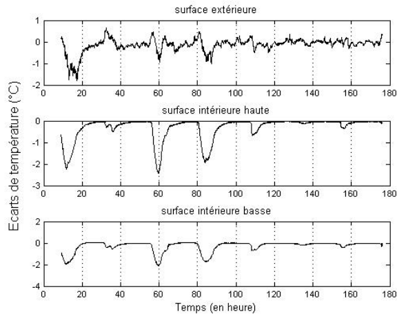
Figure 169 : Gradients longitudinaux sur le panneau de toiture en convection naturelle
