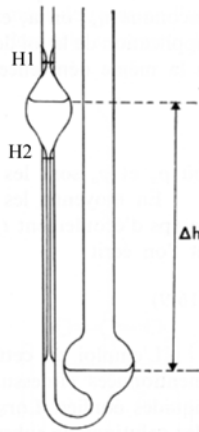
Figure 174 : Tube à capillaire
