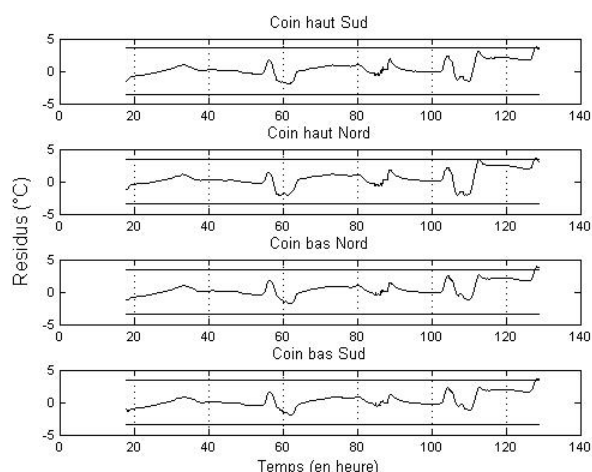
Résidus sur les températures d'air aux 4 coins du système SV1 en régime de convection forcée (du 7 au 12 mars 2007)
