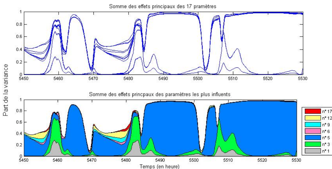
Figure 186 : Effets principaux cumulés des 17 paramètres (en haut) et des paramètres expliquant plus de 10% à un instant donné de la période (en bas) sur la température d'air en entrée de capteur solaire.
