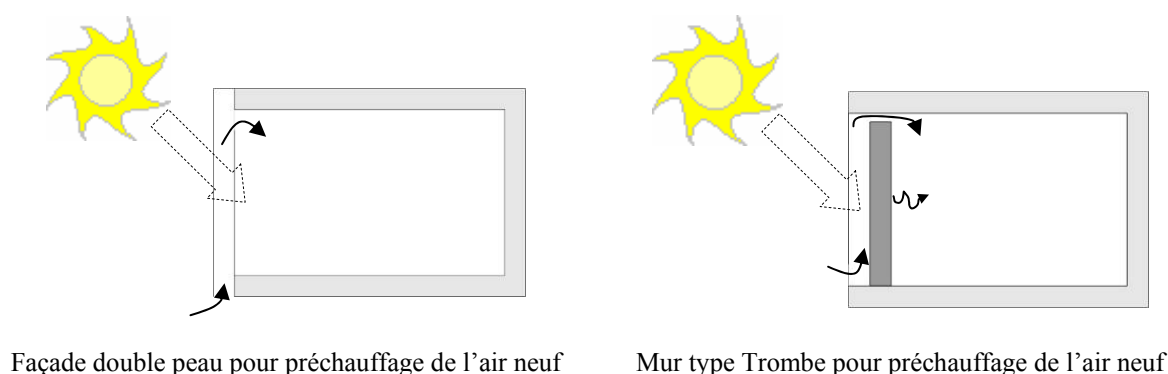
Figure 5 : Intégration de système dédiés au préchauffage de l'air neuf dans le bâtiment
