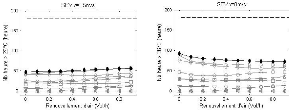
Figure 136 : Nombre d’heure de surchauffe en fonction du taux de renouvellement d’air pour les SENV et SEV sous trois régimes de convection (Grenoble, ép.: 1cm)
