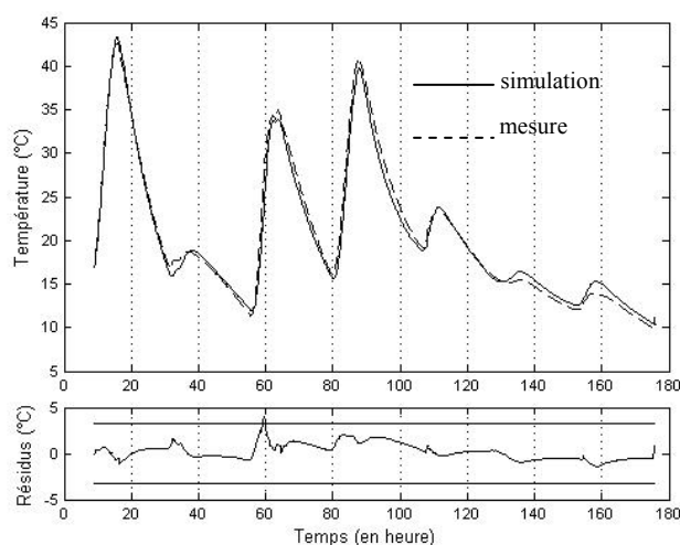
Figure 98 : Evolution des températures du volume intérieur mesurées et simulées avec les résidus correspondants en régime de convection naturelle
