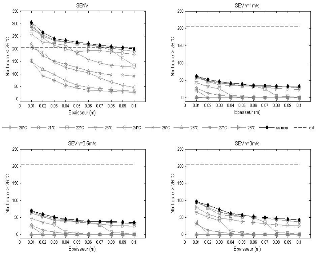
Figure 139 : Nombre d'heure de surchauffe en fonction de l'épaisseur des panneaux d'inertie pour les SENV et SEV sous trois régimes de convection (Nice, tx. d'air: 0,5 Vol/h)
