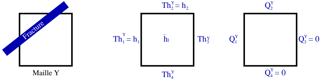
FIG. 2.5 – Maille Y et ses conditions aux limites
