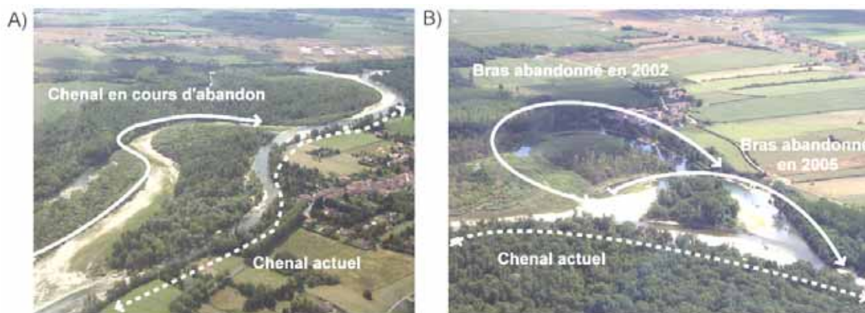
Photographie 3.1 - Recoupements naturels de méandres (A) en aval du pont de Gévrieux et (B) au droit de Martinaz
