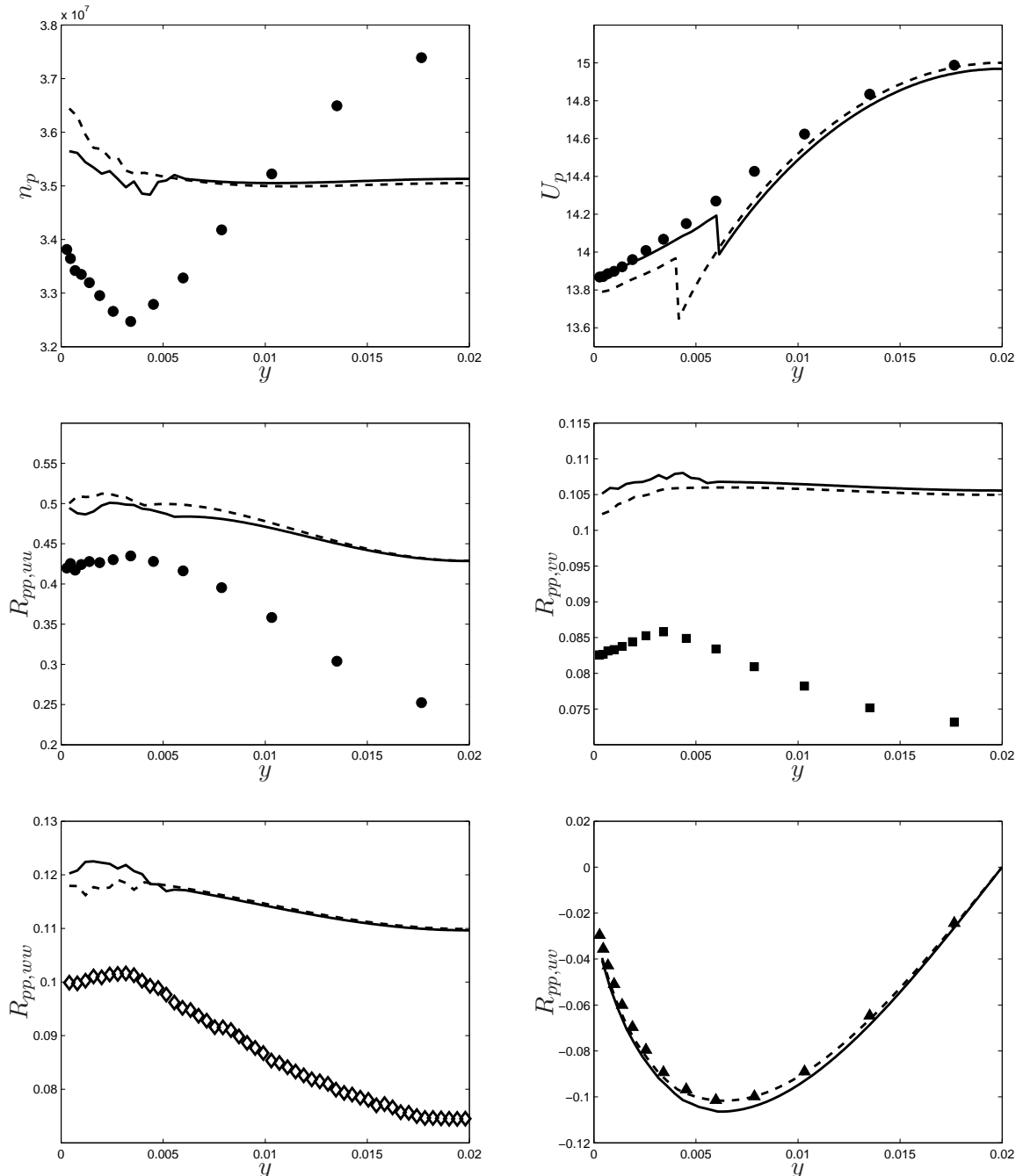
FIG. 6.19 – Influence du rapport de volume \eta dans le cas B3. \circ : lagrangien stochastique ; -\cdot-\cdot- : eulérien (6.19) ; — : HELM avec \eta = 0, 3 ; \cdots\cdots : HELM avec \eta = 0, 2 ; \bullet : DPS (Sakiz [1999]).
