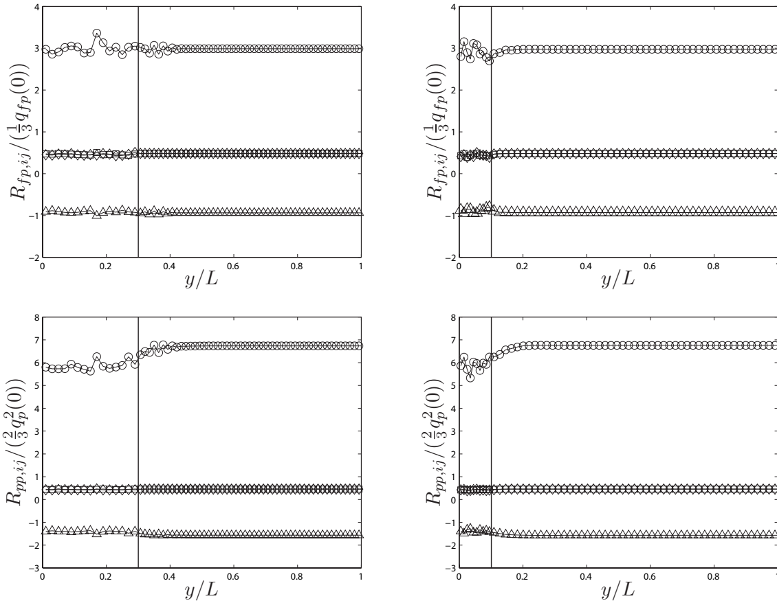
FIG. 5.33 – Profils de contraintes fluide-particules et particulières à l'instant t = 5/S_f issus de HELM avec \eta = 0,3 (gauche) et \eta = 0,1 (droite) ; \circ : R_{uu} , \square : R_{vv} , \diamond : R_{ww} , \triangle : R_{uv} .
