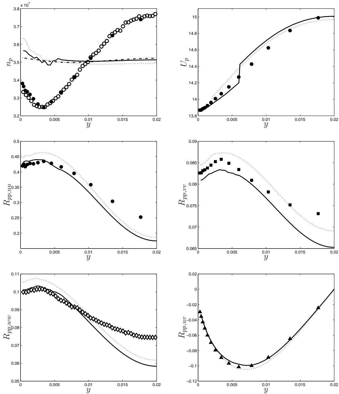
FIG. 6.18 – Influence du rapport de volume \eta dans le cas B3. \circ : lagrangien stochastique ; - \cdot - \cdot - : eulérien (6.19) avec correction par effet de Knudsen (6.18) ; — : HELM-EKC avec \eta = 0, 3 ; \cdots : HELM-EKC avec \eta = 0, 1 ; \bullet : DPS (Sakiz [1999]).
