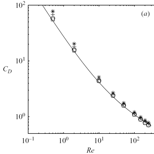
FIG. 1.10 – Influence de la distance à la paroi sur le coefficient de traînée d'une particule isolée pour différents nombre de Reynolds particulaires. \square : y = 4d_p ; \circ : y = 2d_p ; + : y = d_p ; * : y = 0.75d_p ; — : Coefficient de traînée standard (1.46). (Tirée de Arcen et al. [2005]).
