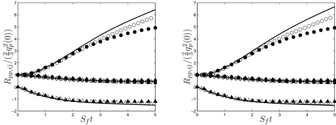
FIG. 5.31 – Développements des contraintes particulières prédits par HELM avec \eta = 0,3 (gauche) et \eta = 0,1 (droite). \circ : moyenne dans le domaine lagrangien ( \circ : R_{pp,uu}, \langle R_{pp,uu} \rangle^- , \square : R_{pp,vv}, \langle R_{pp,vv} \rangle^- , \diamond : R_{pp,ww}, \langle R_{pp,ww} \rangle^- , \triangle : R_{pp,uv}, \langle R_{pp,uv} \rangle^- ); — : moments au 5ième point du maillage pression eulérien ; \bullet : LES/DPS (Laviéville [1997]).
