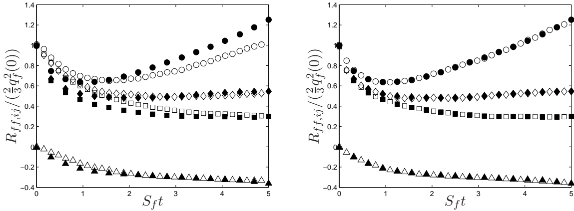
FIG. 5.5 – Développements des contraintes cinétiques du fluide vu par les particules (cas A). gauche : modèle NCLIPM avec correction (5.8), droite : modèle NCLIPM avec correction (5.9). \circ : lagrangien stochastique ( \circ : R_{ff,uu} , \square : R_{ff,vv} , \diamond : R_{ff,ww} , \triangle : R_{ff,uv} ); \bullet : LES/DPS (Laviéville [1997]).
