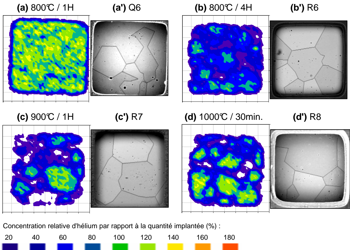
Figure IV-30 : Cartographies d'hélium normalisées d'échantillons polis O.P.U réalisées au LPS (a, b ,c et d) et images MEB (a', b', c' et d') des cases analysées, qui mesurent 63×63 µm 2 . Les joints de grain visibles ont été surlignés.
