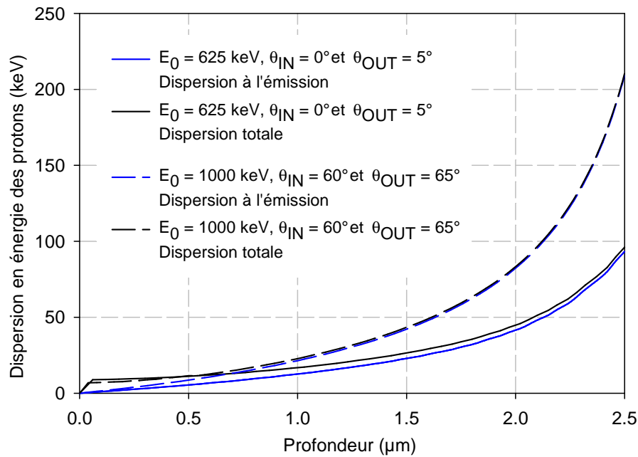
Figure II-20 : Dispersion en énergie des protons émis et totales, après leur passage à travers un filtre en Mylar de 25 \mu\text{m} d'épaisseur, dans deux configurations d'analyse favorables.
