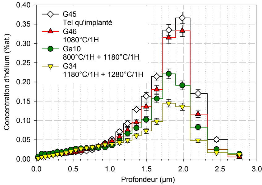
Figure IV-7 : Profils d'hélium dans des échantillons d'UO 2 du lot G implantés en 3 He + de 1 MeV à 2x10 16 3 He.cm -2 puis recuits dans le four V à haute température de 1080°C à 1280°C.
