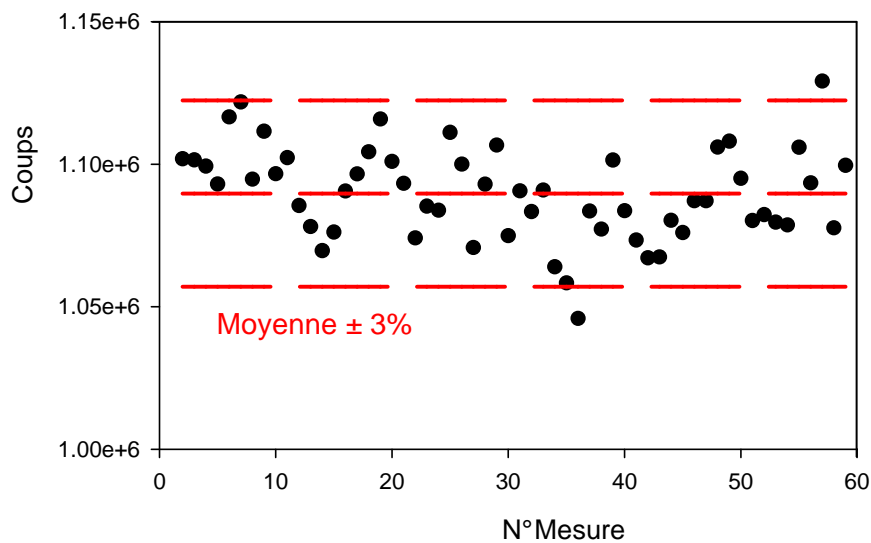
Figure II-31 : Dispersion du nombre d'ions ^4He rétrodiffusés sur les atomes d'U d'une cible d' UO_2 à charge d'analyse constante.
