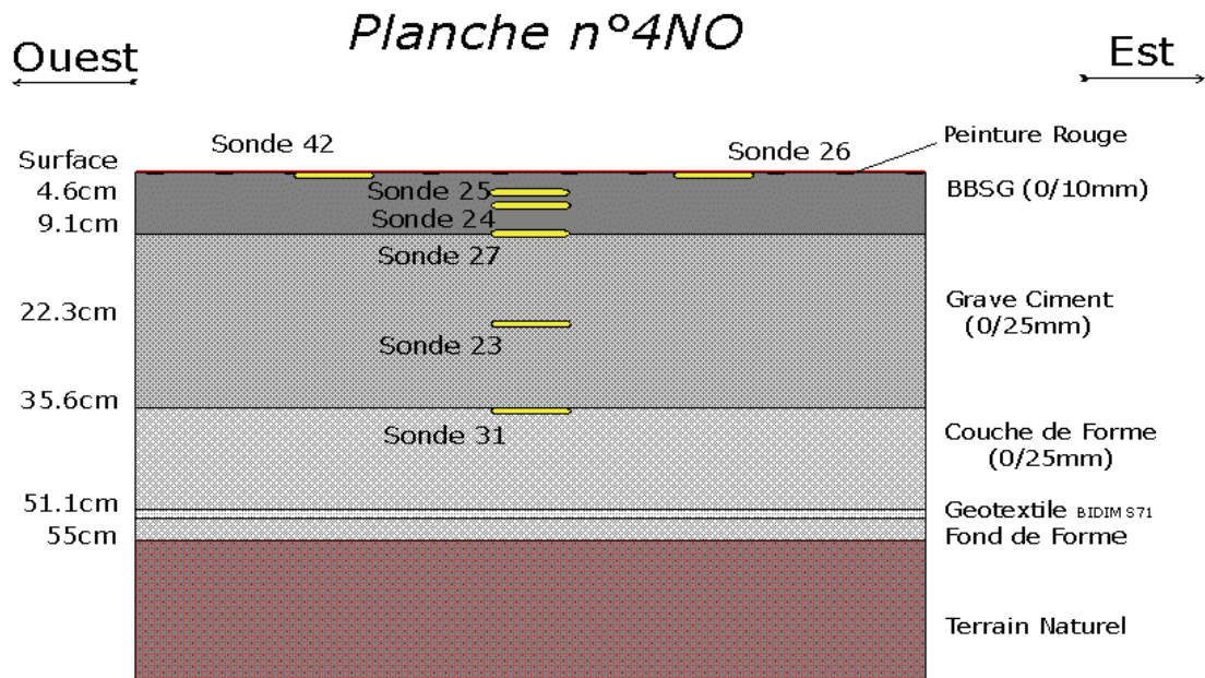
Figure A.7 : Description de la structure de la chaussée n°4NO.
