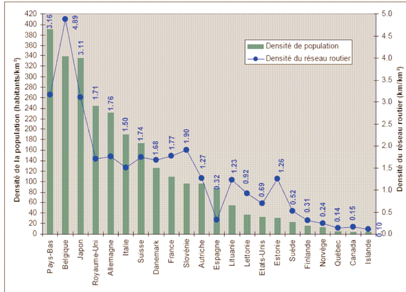
Figure 2.2 : Densités de population et du réseau routier pour des pays soumis à la viabilité hivernale, d'après Snow & Ice Databook 2006.
