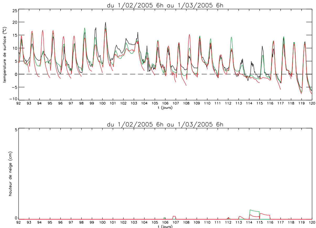
Figure 6.18 : a) Comparaison pour le mois de février 2005 de la température de surface mesurée sur l'autoroute A10 (—) avec la température de surface simulée avec le forçage analysé (—) et avec la prévision (—) ; b) Simulations des hauteurs de neige sur la chaussée avec le forçage analysé (—) et en prévision(—).
