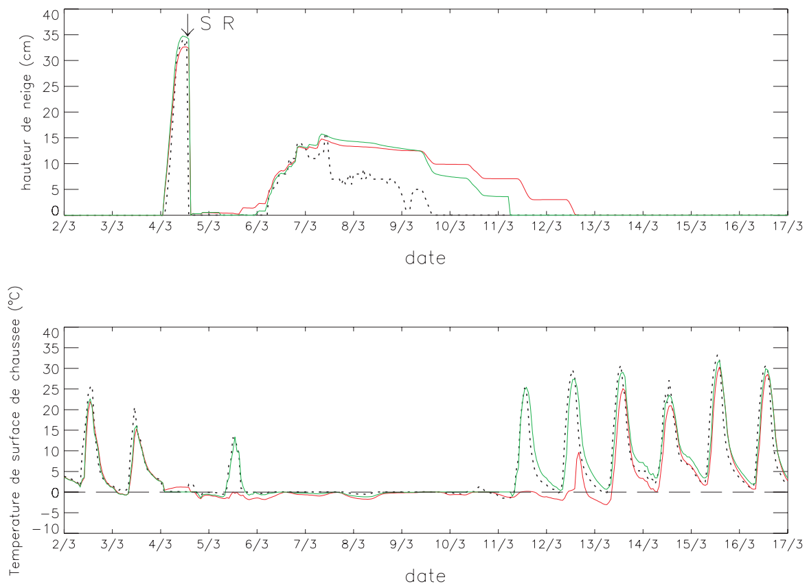
Figure 4.11 : Comparaison pour la période du 2 au 17 mars a) des hauteurs de neige mesurées (trait discontinu) et des hauteurs de neige simulées avec le modèle ISBA-Route couplé avec CROCUS (trait continu vert) et couplé avec ISBA-ES (trait continu rouge), avec présence d'un déneigement manuel (↓ SR). b) des températures de surface mesurées (trait discontinu) et simulées avec le modèle ISBA-Route couplé avec CROCUS (trait continu vert) et couplé avec ISBA-ES (trait continu rouge).
