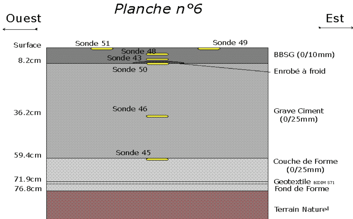
Figure A.9 : Description de la structure de la chaussée n°6.
