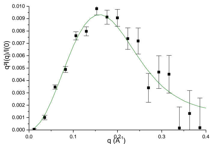
Figure III.33 : Représentation de Kratky ( q^2 I(q)/I(0)=f(q) ) pour une solution de BPTI 85 mg/ml en tampon acide acétique deutéré 50 mM en D 2 O pD 4,5 avec 100 mM (ND 4 ) 2 SO 4 à pression atmosphérique. La ligne verte représente la représentation de Kratky issue de la simulation à partir de la structure cristallographique du BPTI (6PTI.pdb).
