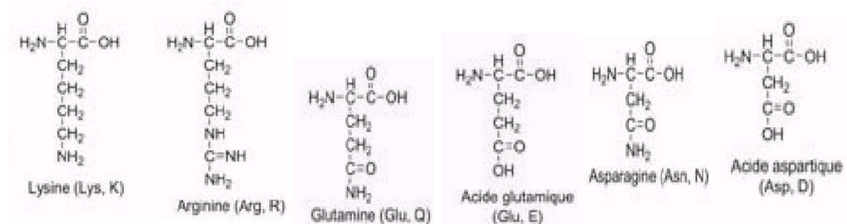
Figure IV.9 : représentation des résidus possédant une longue chaîne latérale.
