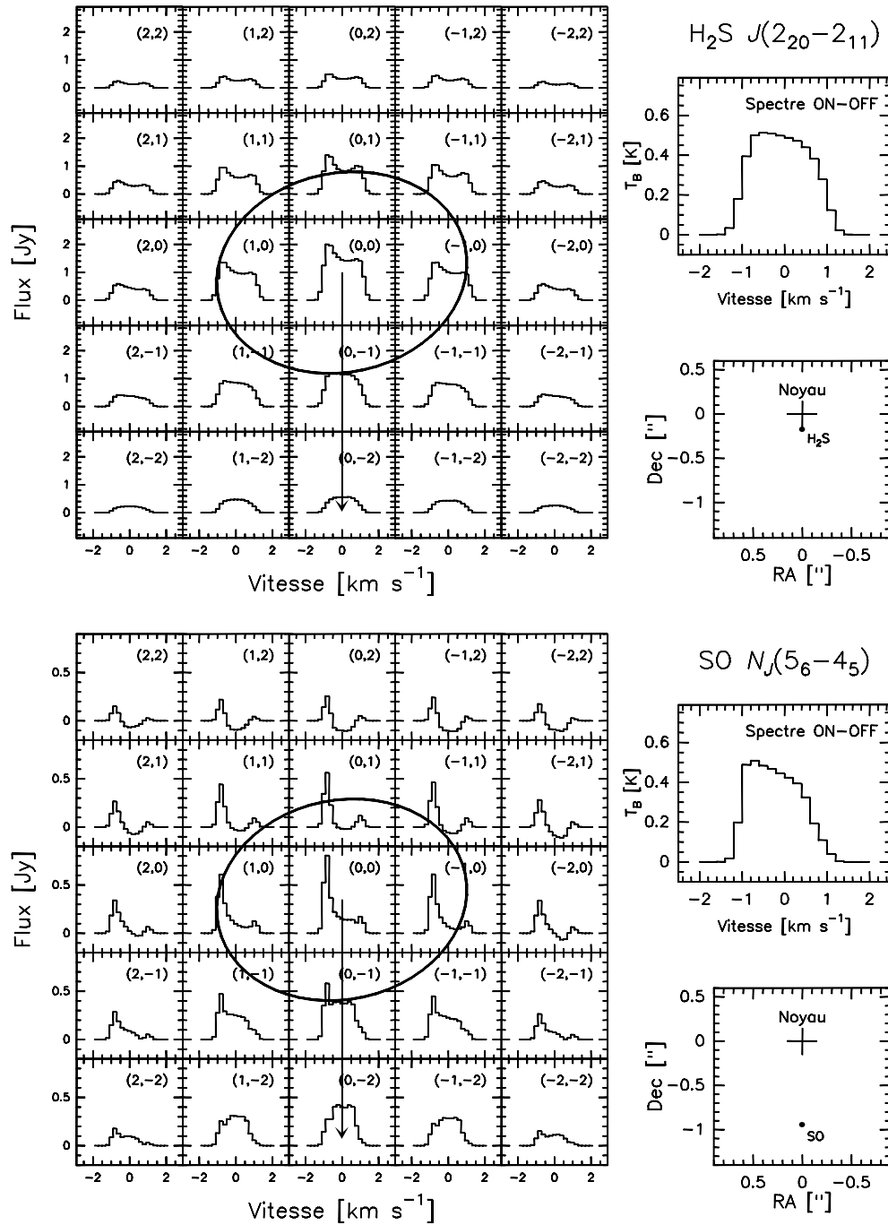
Fig. 4.22: Cartes spectrales, spectres ON-OFF et décalages (O-Nucl) simulés pour la raie (2 20 -2 11 ) de H 2 S ( en haut ) avec un modèle incluant un jet ( J = 0,2 et \psi = 40^\circ ) et une asymétrie jour/nuit ( r_{jn} = 1,5 ). Pour SO ( en bas ), on a J = 0,4 , \psi = 40^\circ et r_{jn} = 5 .
