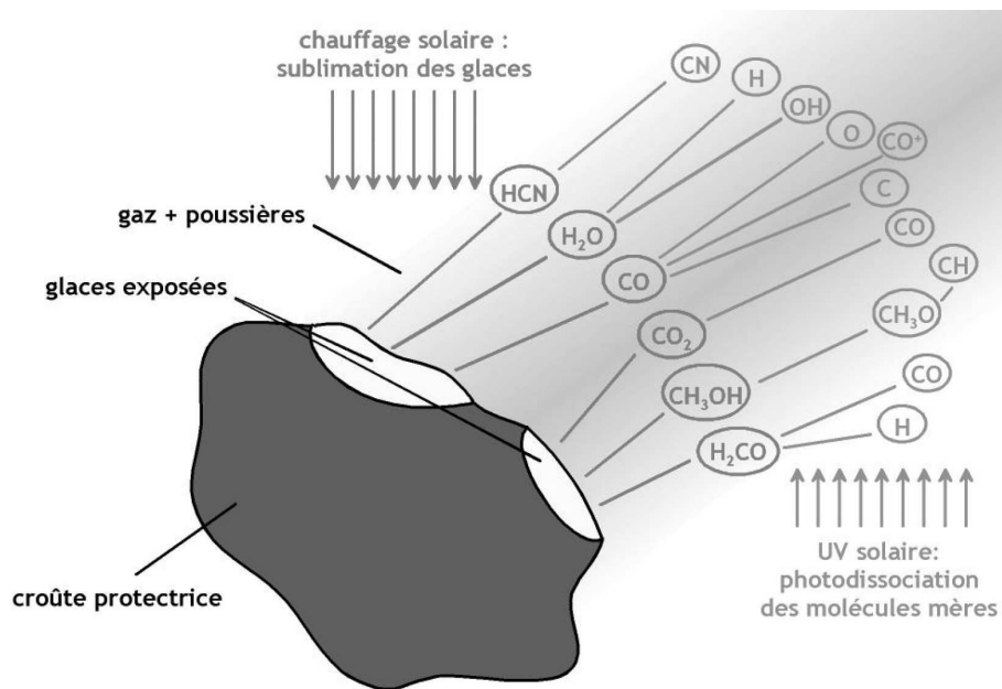
Fig. 1.3: Un noyau cométaire et sa coma. Ce schéma résume les processus actifs dans les atmosphères cométaires : sublimation des glaces, photoionisation et photodissociation des molécules mères (Figure issue de Henry, 2003).
