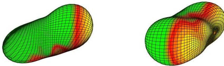
Fig. 5.11: Noyau utilisé dans le modèle de Rodionov et Crifo (2006) à deux moments distincts (séparés de 3,8 h, soit un tiers de période) au cours de la rotation dont l'axe moyen est vertical. La forme choisie est celle du noyau de la comète de Halley dont la taille a été augmentée pour être en accord avec les estimations de la taille du noyau de la comète Hale-Bopp. Les couleurs représentent l'illumination de la surface par le Soleil, situé vers la droite.
