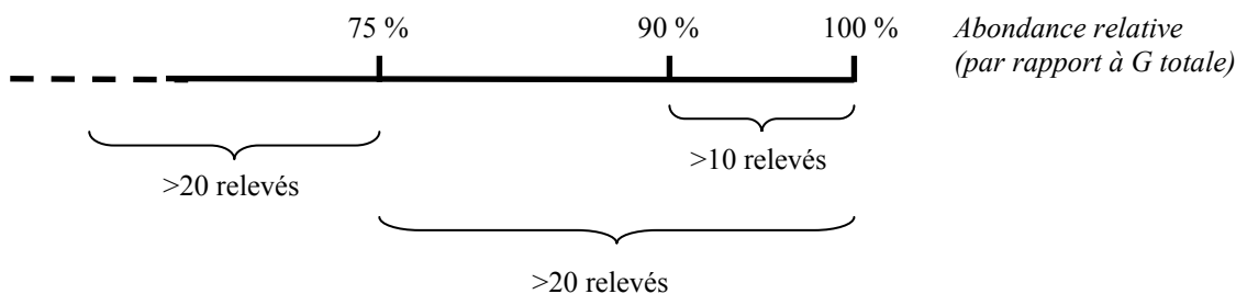
Figure 4.10 : critère de sélection des essences principales (et groupes d'essences principaux) dont la pureté est suffisamment bien distribuée pour être testée.
