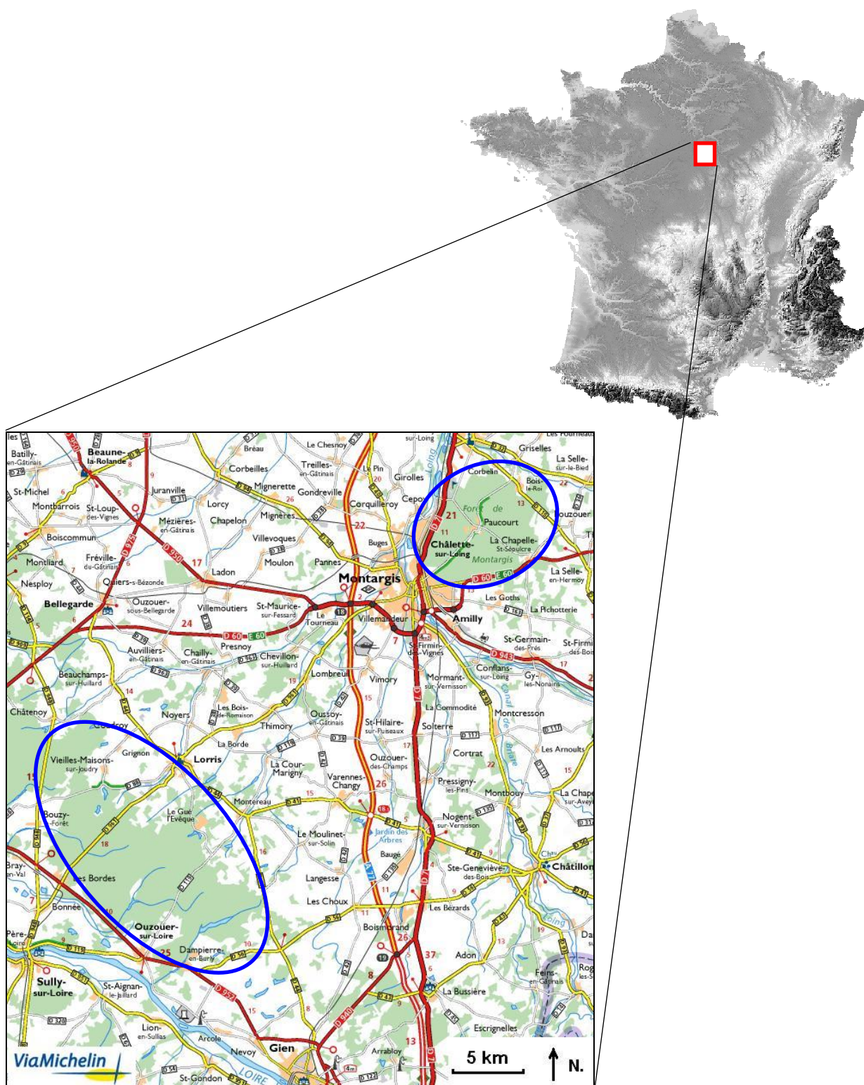
Figure 2.1 : carte des massifs forestiers étudiés : forêt de Montargis (en haut à droite) et partie sud-est du massif de Lorris de la forêt d'Orléans (en bas à gauche).
