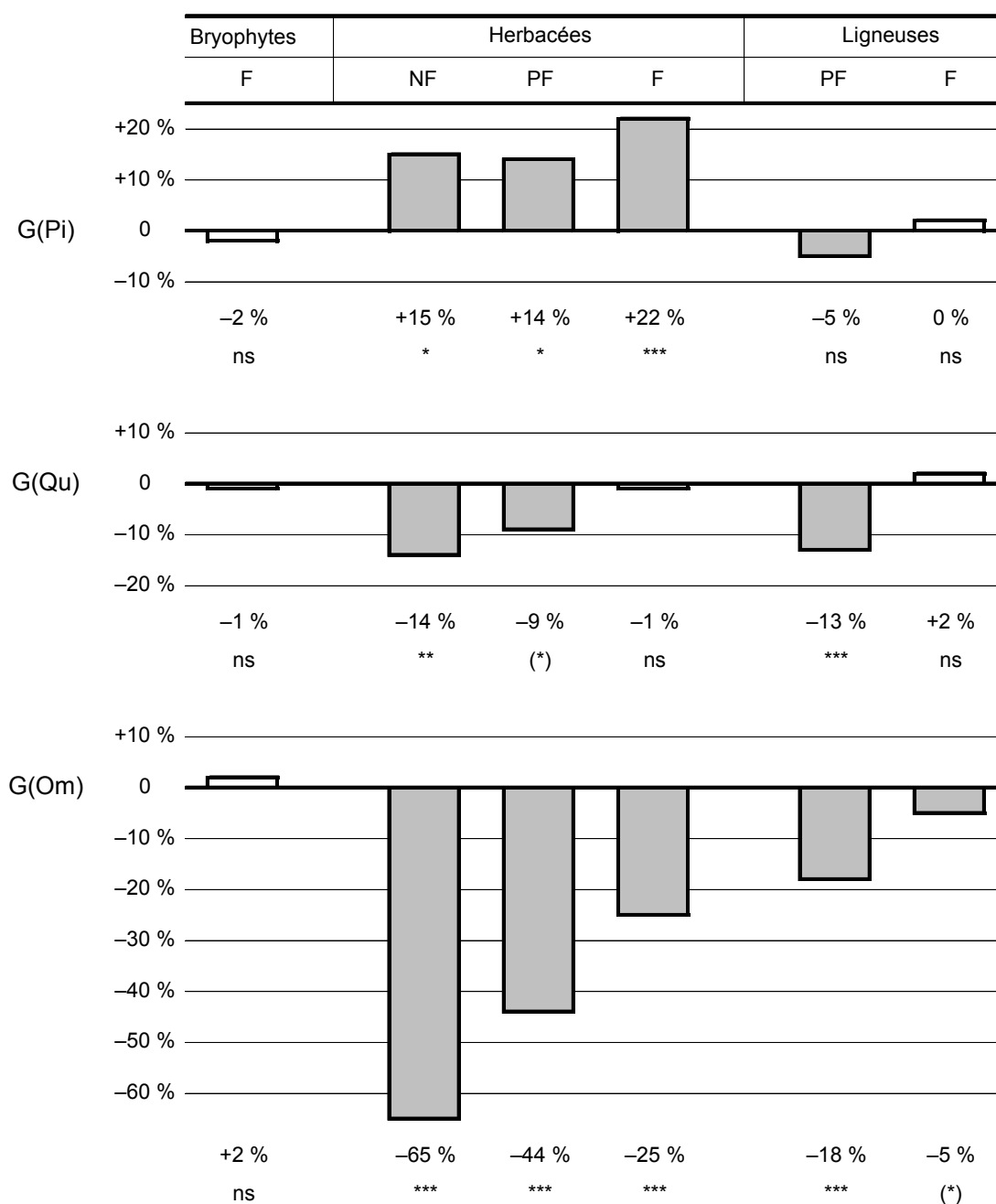
Figure 3.13 : réponse de la richesse écologique de la flore (classification "For") à une augmentation de +5 \text{ m}^2.\text{ha}^{-1} de l'un des trois groupes d'essences (modèle \Sigma G(ge) ). "NF" = non forestières ; "PF" = péri-forestières ; "F" = forestières.
