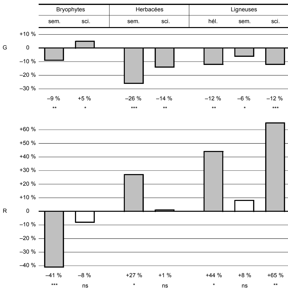
Figure 3.12 : réponse de la richesse écologique de la flore (classification "Hélio") à une augmentation de +5 \text{ m}^2.\text{ha}^{-1} de la surface terrière totale et de +2 essences (modèle G+R ). "hél." = héliophiles ; "sem." = semi-héliophiles ; "sci." = sciaphiles.
