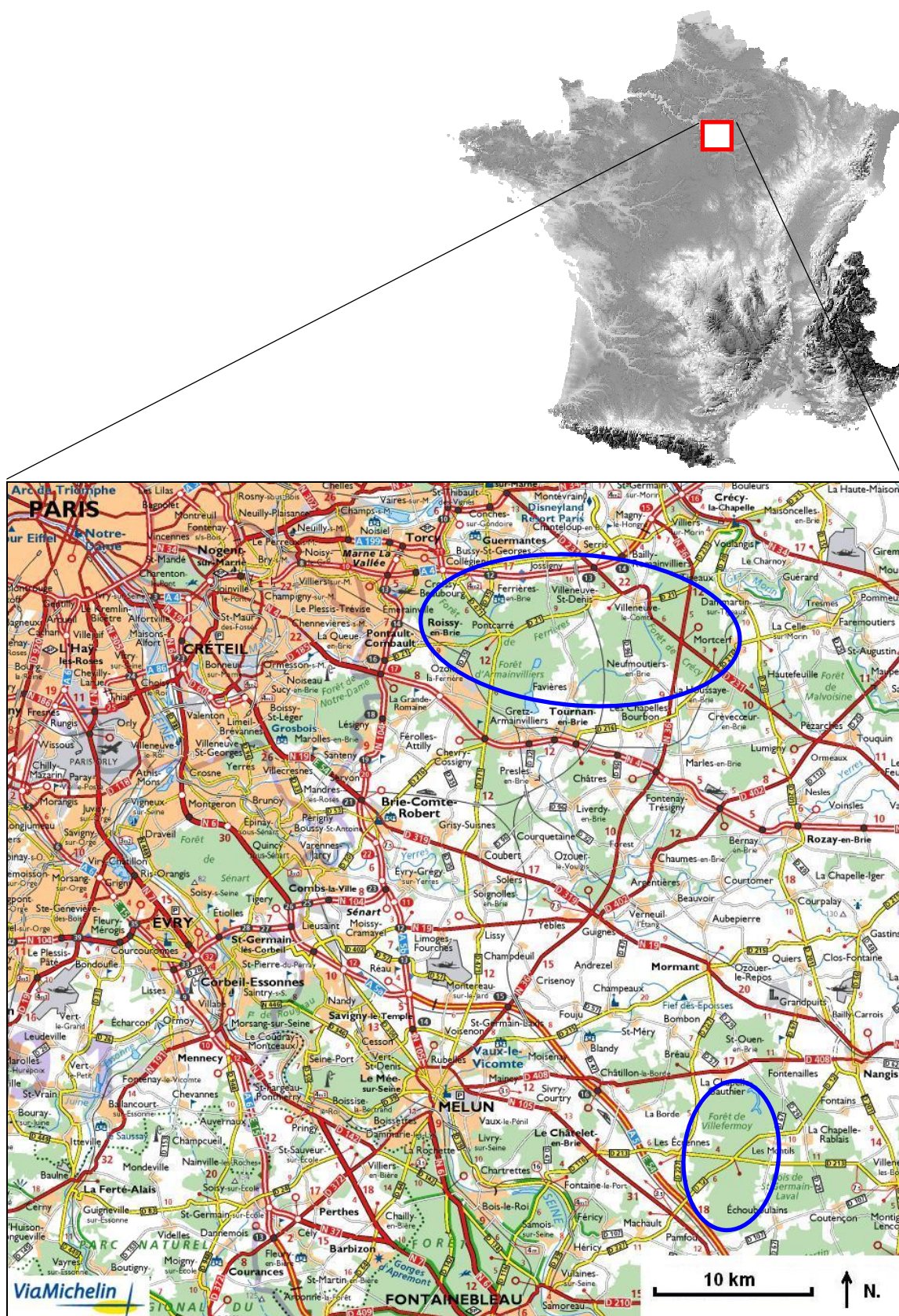
Figure 3.1 : carte des massifs forestiers étudiés : forêts de Ferrières, Armainvilliers et Crécy (en haut) et forêt de Villefermy (en bas).
