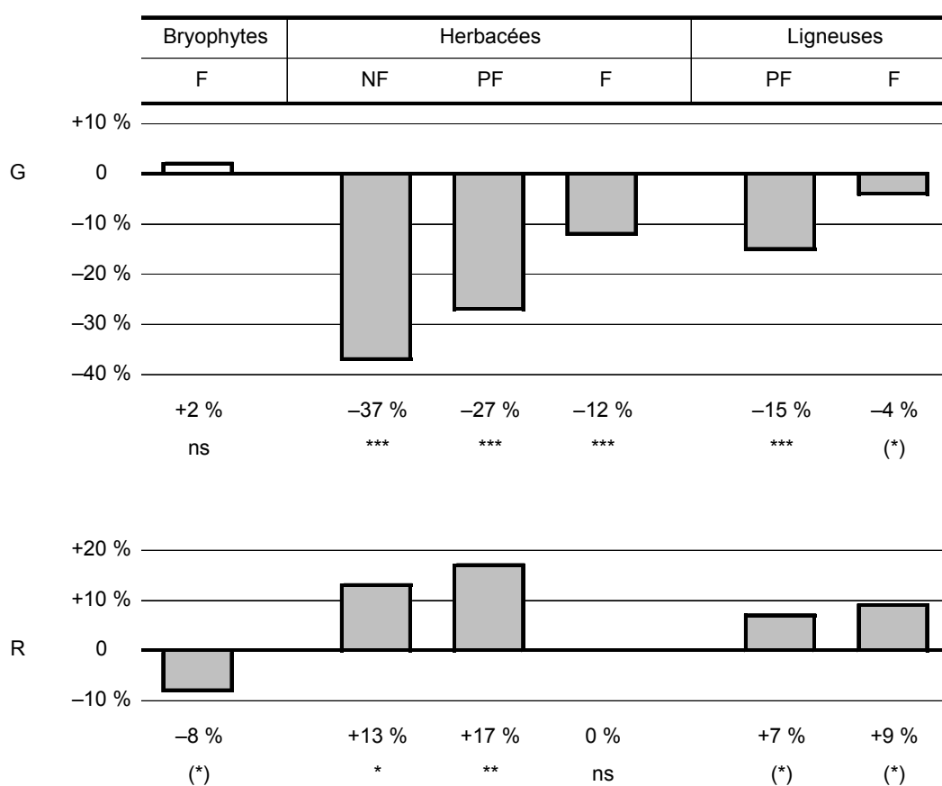
Figure 3.11 : réponse de la richesse écologique de la flore (classification "For") à une augmentation de +5 m 2 .ha -1 de la surface terrière totale et de +2 essences (modèle G+R ). "NF" = non forestières ; "PF" = péri-forestières ; "F" = forestières.
