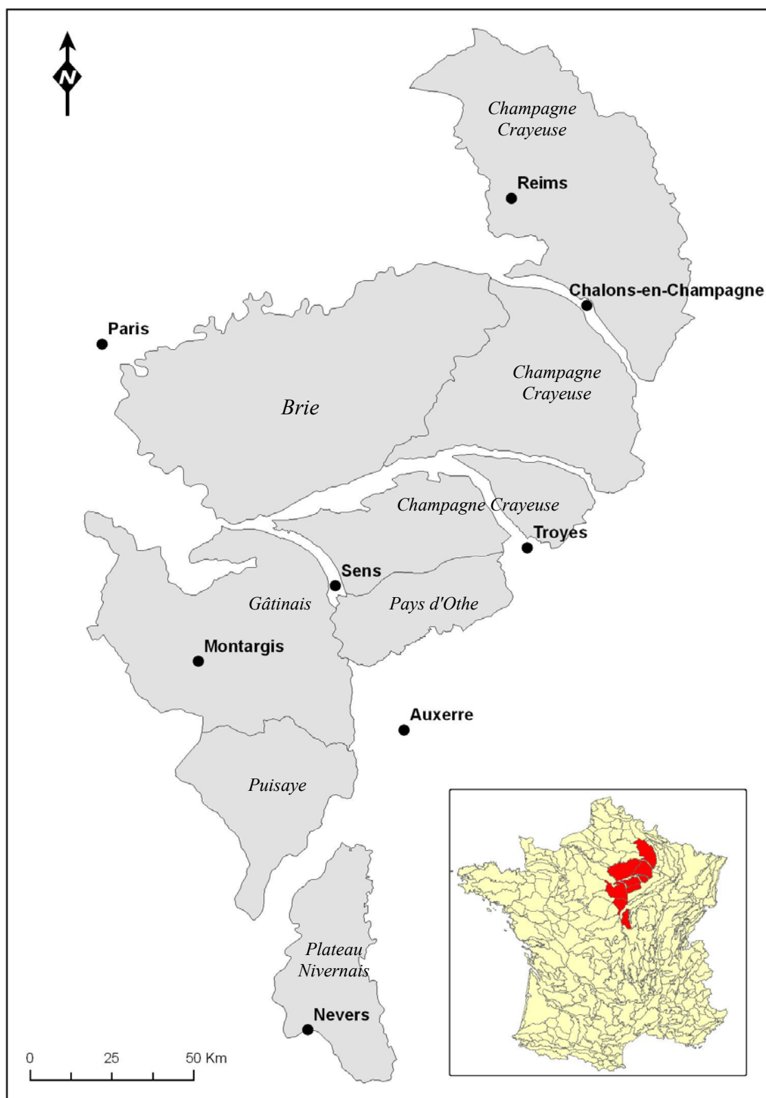
Figure 4.2 : carte des régions forestières étudiées.
