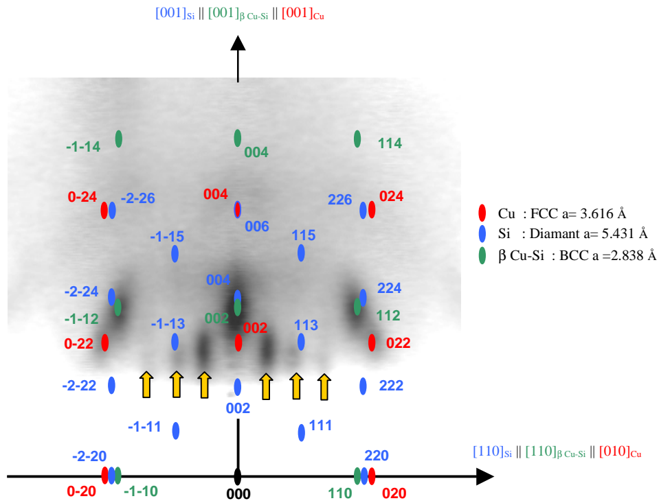
Figure II-14 : Diagramme RHEED expérimental obtenu pour une épaisseur de cuivre de 1,4 nm suivant l'azimut Si \langle 110 \rangle avec en superposition les diagrammes RHEED théoriques de Cu, Si et \beta Cu-Si. Les taches satellites repérées par des flèches correspondent à des taches de macles suivant les plans \{112\} et à des taches de diffraction multiple.
