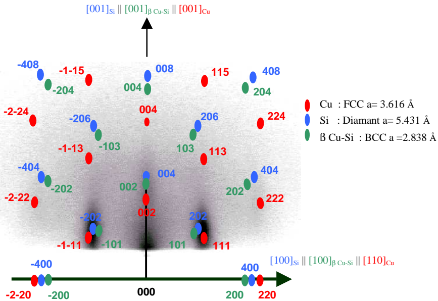
Figure II-15 : Diagramme RHEED expérimental obtenu pour une épaisseur de cuivre de 1,4 nm suivant l'azimut \langle 100 \rangle_{Si} avec en superposition les diagrammes RHEED théoriques de Cu, Si et \beta Cu-Si.
