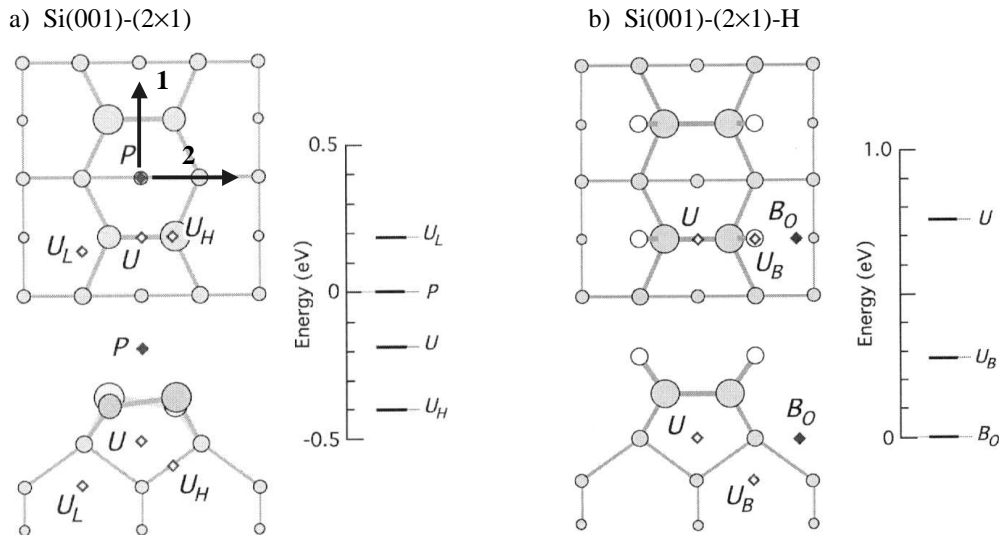
Figure II-7 : Représentation (en coupe et vue de dessus) des sites les plus énergétiquement stables pour un atome Ni près de la surface : Sites U, U L , U H , dans le silicium et P sur la surface pour Si(001)-(2x1) (a) et sites U, U B , dans le silicium et B 0 sur la surface pour Si(001)-(2x1)-H (b). Les énergies du système en fonction de la position de l'atome Ni sont également représentées (le niveau d'énergie nulle correspond à la position de l'atome de nickel sur le site en surface P ou B 0 ). Les flèches indexées 1 et 2 représentent les directions de diffusion de l'atome Ni parallèlement et perpendiculairement respectivement aux lignes de dimères Si. D'après S. Higai et T. Ohmo [40].
