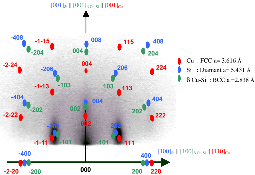
Figure II-15 : Diagramme RHEED expérimental obtenu pour une épaisseur de cuivre de 1,4 nm suivant l'azimut \langle 100 \rangle_{Si} avec en superposition les diagrammes RHEED théoriques de Cu, Si et \beta Cu-Si.
