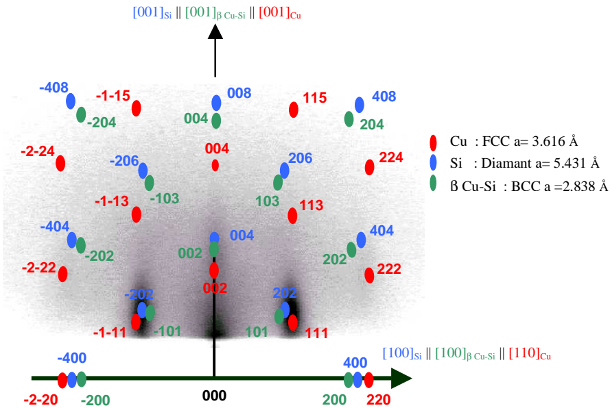
Figure II-15 : Diagramme RHEED expérimental obtenu pour une épaisseur de cuivre de 1,4 nm suivant l'azimut <100> Si avec en superposition les diagrammes RHEED théoriques de Cu, Si et β Cu-Si.
