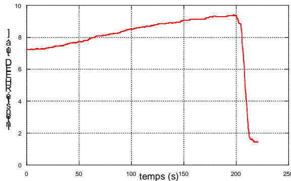
Figure III-7 : Evolution de l'intensité du signal RHEED sur une couche mince de Cu(001) épitaxiée sur Si(001). La chute de l'intensité après 200 secondes traduit un changement rapide (en quelques secondes) de la structure de la surface du Cu dû à la formation du siliciure
