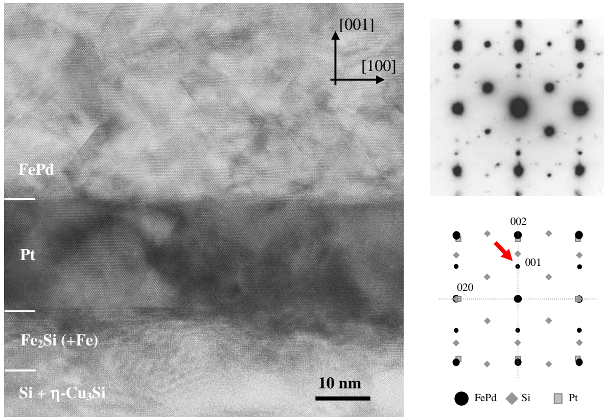
Figure III-34 : Image de haute résolution d'une section de l'échantillon Si(001)/Cu-Si/Fe/Pt/FePd (35nm)/Pd suivant l'axe de zone [1-10]_{Si} et cliché de diffraction correspondant. Les taches de surstructure de la phase L1_0 sont indiquées par une flèche.
