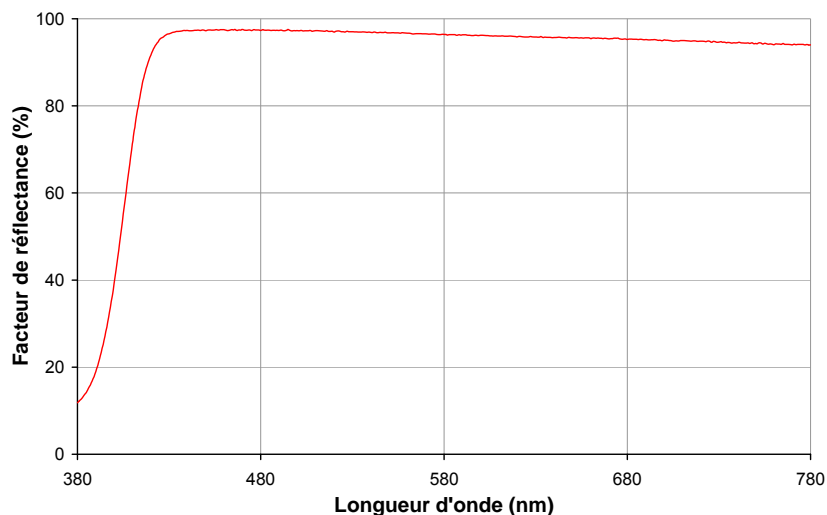
Fig. III-18 : Spectre de réflexion diffuse du blanc de titane mesurée avec le Cary et sa sphère d'intégration
