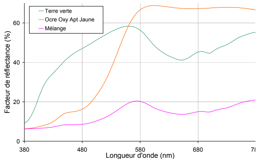
Fig. III-26 : Spectres de réflexion diffuse de couches picturales mesurés en configuration 0^\circ /diffus pour un mélange de terre verte et d'un ocre jaune, ainsi que pour les constituants mesurés séparément
