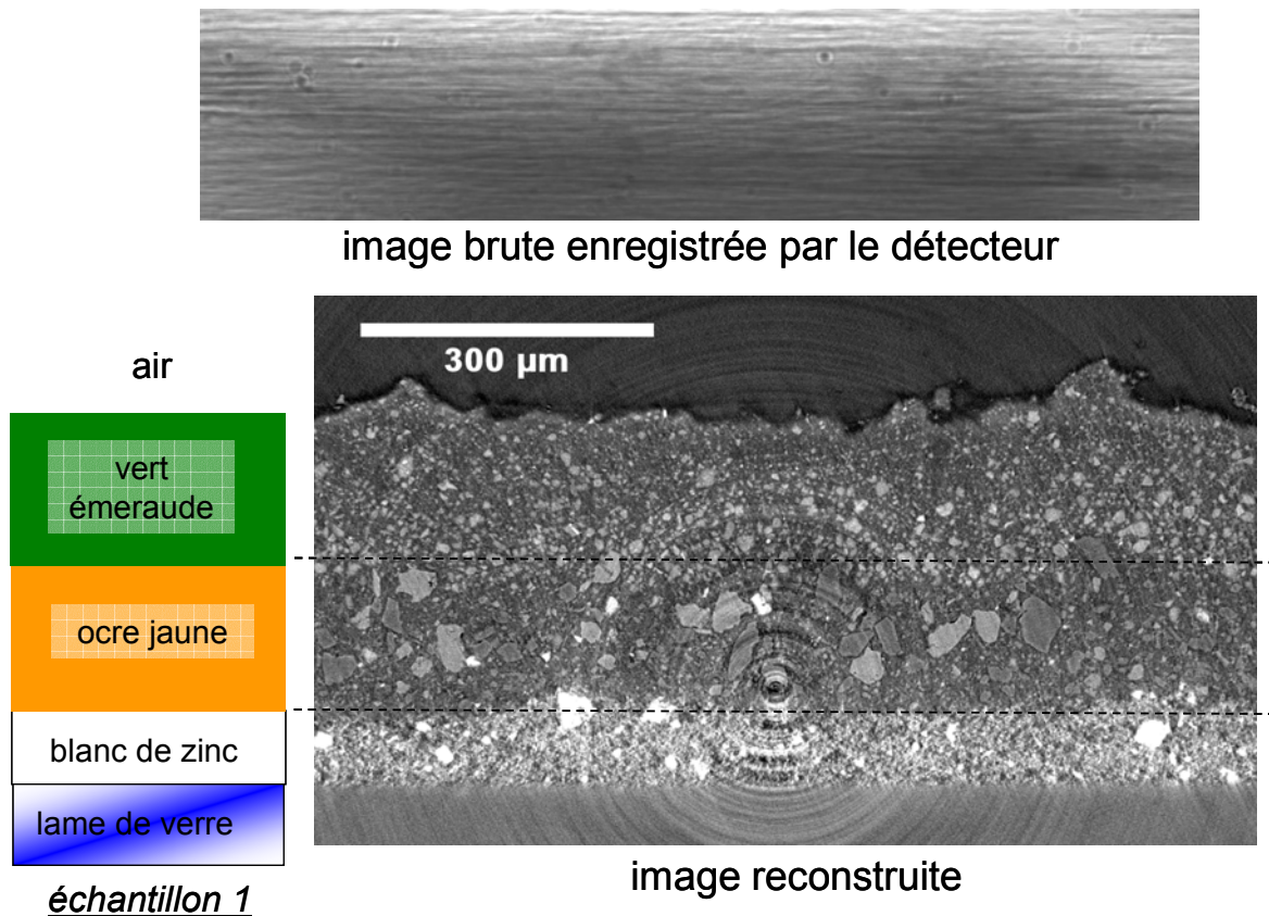
Fig. V-3 : Image de l'intensité transmise par l'échantillon 1 (en haut) et image d'absorption X reconstruite, équivalente à une coupe verticale (en bas)
