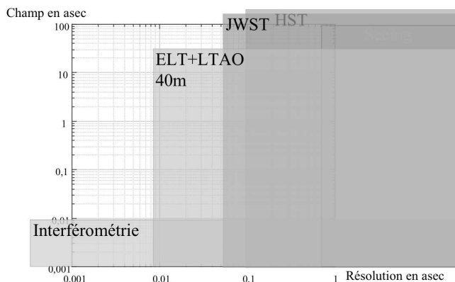
FIG. 8.10 – Les principaux instruments futurs sont représentés sur ce diagramme dimension de champ vs résolution maximale atteignable. Si les caractéristiques du JWST sont fixées, celles du (des) ELT ne le sont pas encore, notamment au niveau du type d'optique adaptative qui sera utilisée, et en conséquence quel sera le compromis entre l'étendue de champ et la résolution qui sera obtenu. Les performances de l'ELT représentées ici sont pour le cas de l'utilisation d'une optique adaptative dite "Laser Tomography AO", mais peuvent "glisser" jusqu'à être proches de celles du JWST, ou en eXtremeAO avoir une résolution meilleure mais un champ de l'ordre de la seconde d'arc. Les interféromètres longue base sont limités en champ à cause de leur nombre d'ouvertures.
