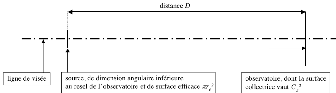
FIG. 8.1 – Etendue de faisceau S\Omega d'une source dont l'extension angulaire sur le ciel est inférieure au resel de l'observatoire. On a alors S = \pi r_e^2 et \Omega = 4\pi \frac{C_g^2}{4\pi D^2} . L'étendue de faisceau S\Omega vaut S\Omega = \pi r_e^2 \frac{C_g^2}{D^2} . Elle est dépendante de C_g , de D et de r_E .
