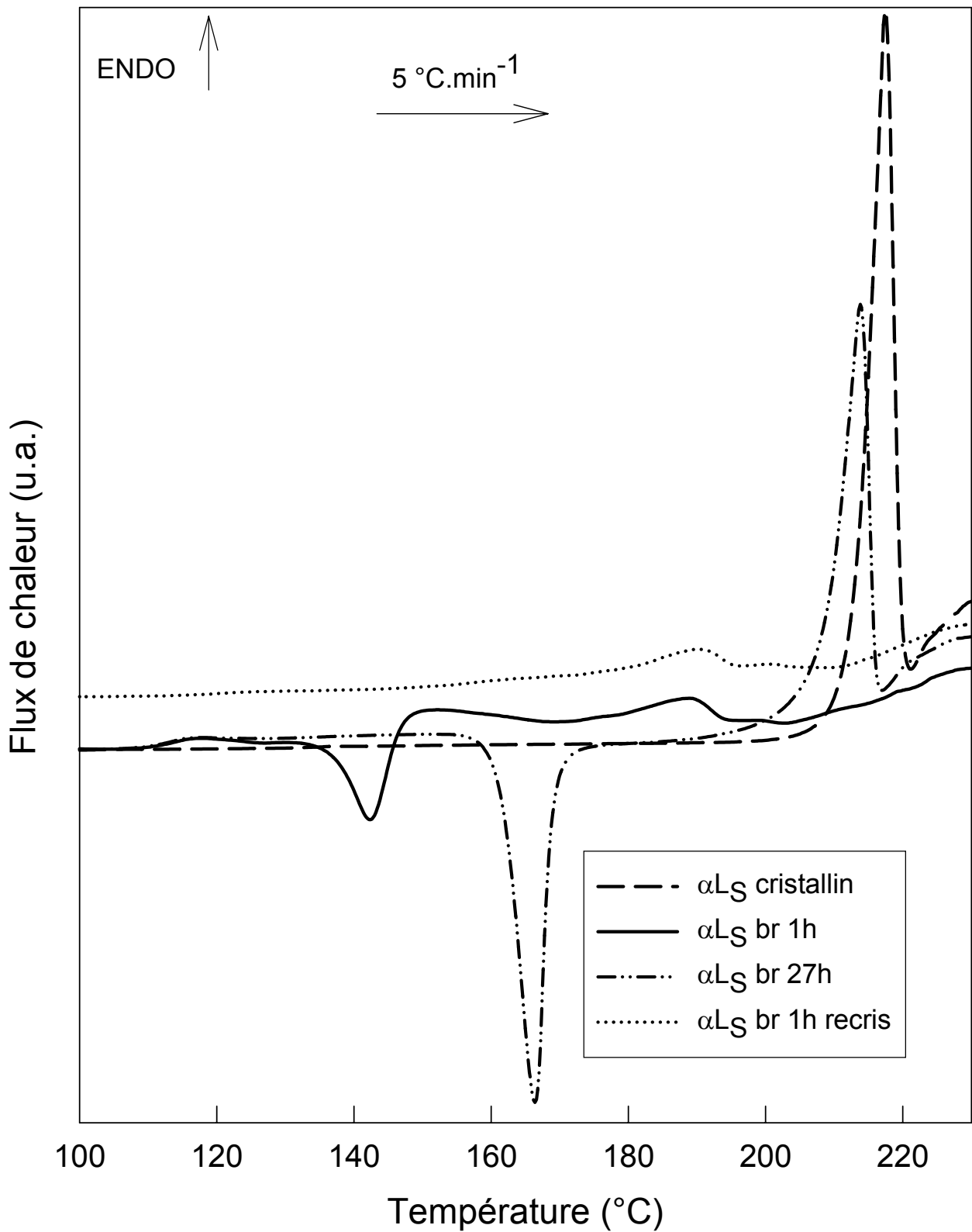
Fig. VII.1 : Thermogrammes enregistrés au chauffage ( 5\text{ °C}\cdot\text{min}^{-1} ) d'échantillons de \alpha\text{L}_S cristallin, broyé 1h, broyé 27h, et broyé 1h puis recristallisé dans la zone de températures de cristallisation rapide. La position en flux de chaleur du thermogramme du \alpha\text{L}_S broyé 1h puis recristallisé a été décalée vers le haut afin de permettre une meilleure visibilité
