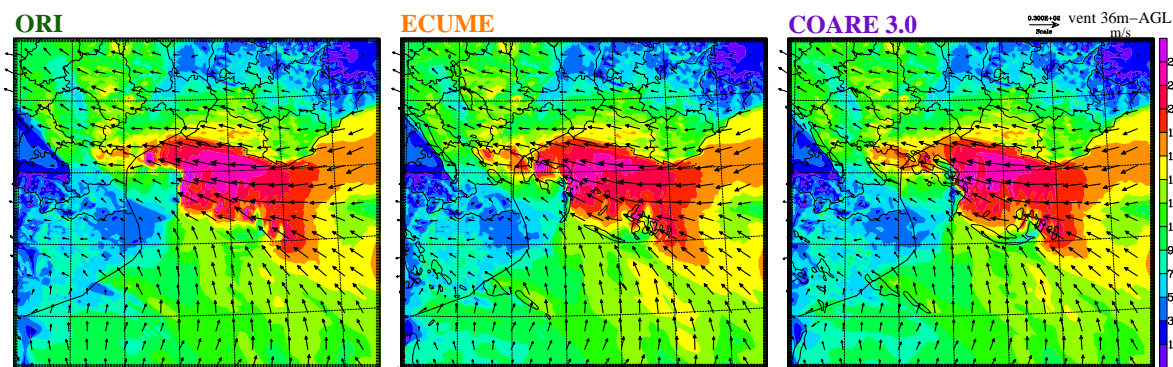
FIG. 7.8 : Vent au premier niveau du modèle ( m s^{-1} ) pour les simulations sur le cas de l'Aude le 13 novembre 1999 à 06UTC. En isolignes, les zones où les différences de vent au premier niveau pour ECUME et COARE 3.0 par rapport à la simulation de référence sont supérieures à 5 m s^{-1} en valeur absolue.
