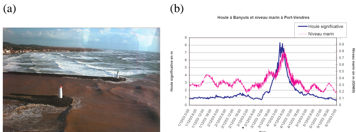
FIG. 3.14 : (a) Photographie du ressaut hydraulique à l'entrée de l'Hérault le 4 décembre 2003 à 12h d'après Hontarrède et al. (2004). (b) Évolution entre le 1 er et le 6 décembre 2003 de la houle à Banyuls et du niveau marin à Port-Vendres dans le département des Pyrénées-Orientales (Source : Météo-France).
