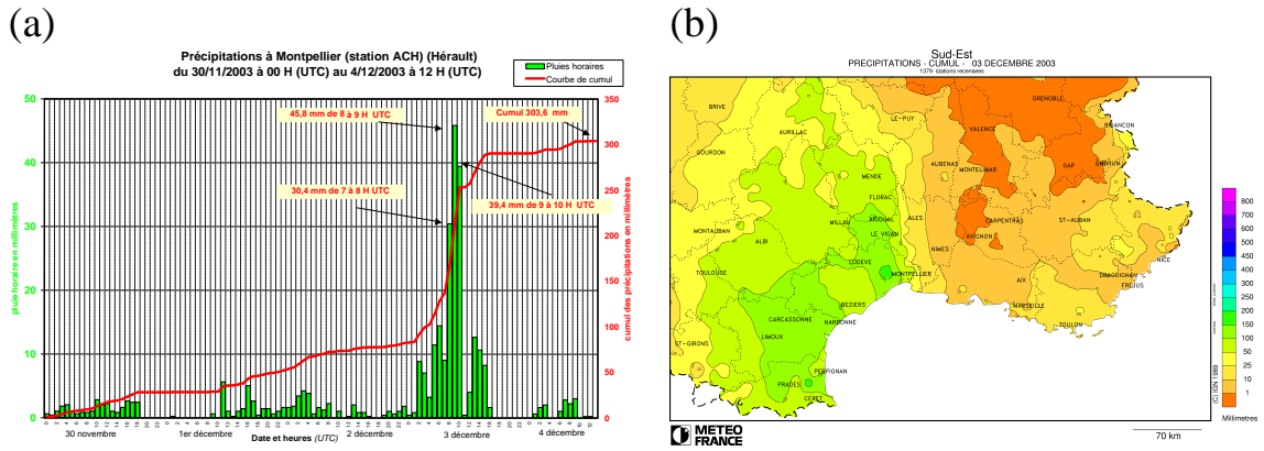
FIG. 3.15 : Précipitations observées : (a) précipitations horaires à Montpellier dans l'Hérault relevées entre le 30 novembre et le 4 décembre 2003 et (b) cumuls de précipitations sur 24h entre le 3 décembre 2003 00UTC et le 4 décembre 2003 à 00UTC. Source : Météo-France
