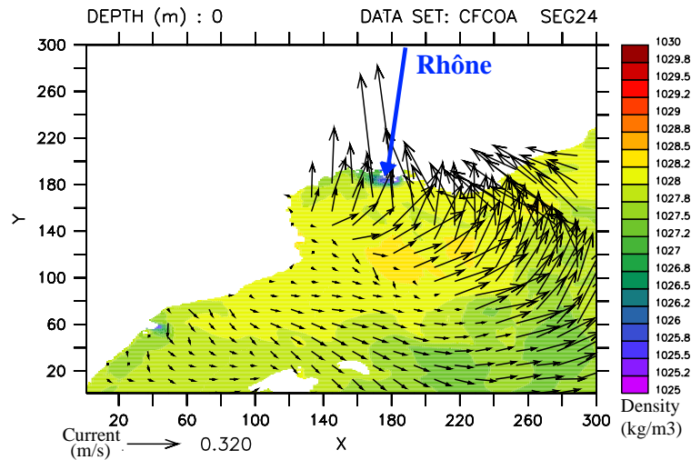
FIG. 9.29 : Densité de l'eau de mer en surface et courant océanique induit dans le golfe du Lion pour la simulation de référence CFCOA, le 4 déc. 2003, 00UTC.
