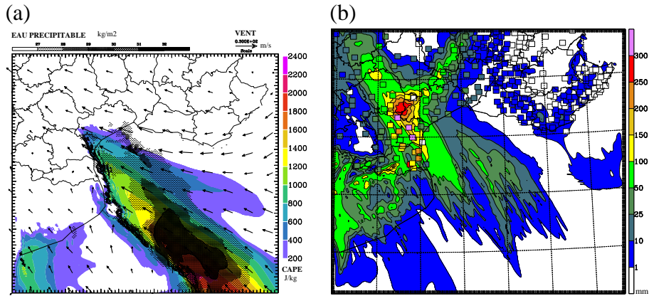
FIG. 5.5 : Simulation de référence (arp12) pour le cas de l'Aude : (a) Environnement à méso-échelle simulé le 13 novembre 1999 à 00UTC : CAPE ( J\text{ kg}^{-1} , en couleurs), vent à environ 36 m au dessus du sol ( \text{m s}^{-1} , flèches) et eau précipitable ( \text{kg m}^{-2} , en grisés ; les isolignes délimitent les zones où l'eau précipitable est supérieure à 29\text{ kg m}^{-2} ). (b) Cumuls de précipitation simulés sur 18h (mm, plages de couleurs) comparés aux cumuls pluviométriques observés sur la même période (carrés de couleur).
