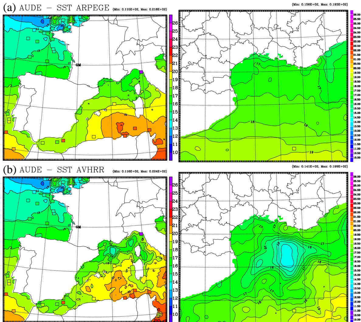
FIG. 5.1 : Cas de l'Aude, 12-13 novembre 1999 : champs de SST (°C) sur les domaines à 9.5 et 2.4 km (a) SST ARPEGE et (b) SST à haute résolution. Les observations de SST enregistrées par les bouées et bateaux le 12 novembre 1999 à 12UTC sont pointées sous forme de carrés de couleur.
