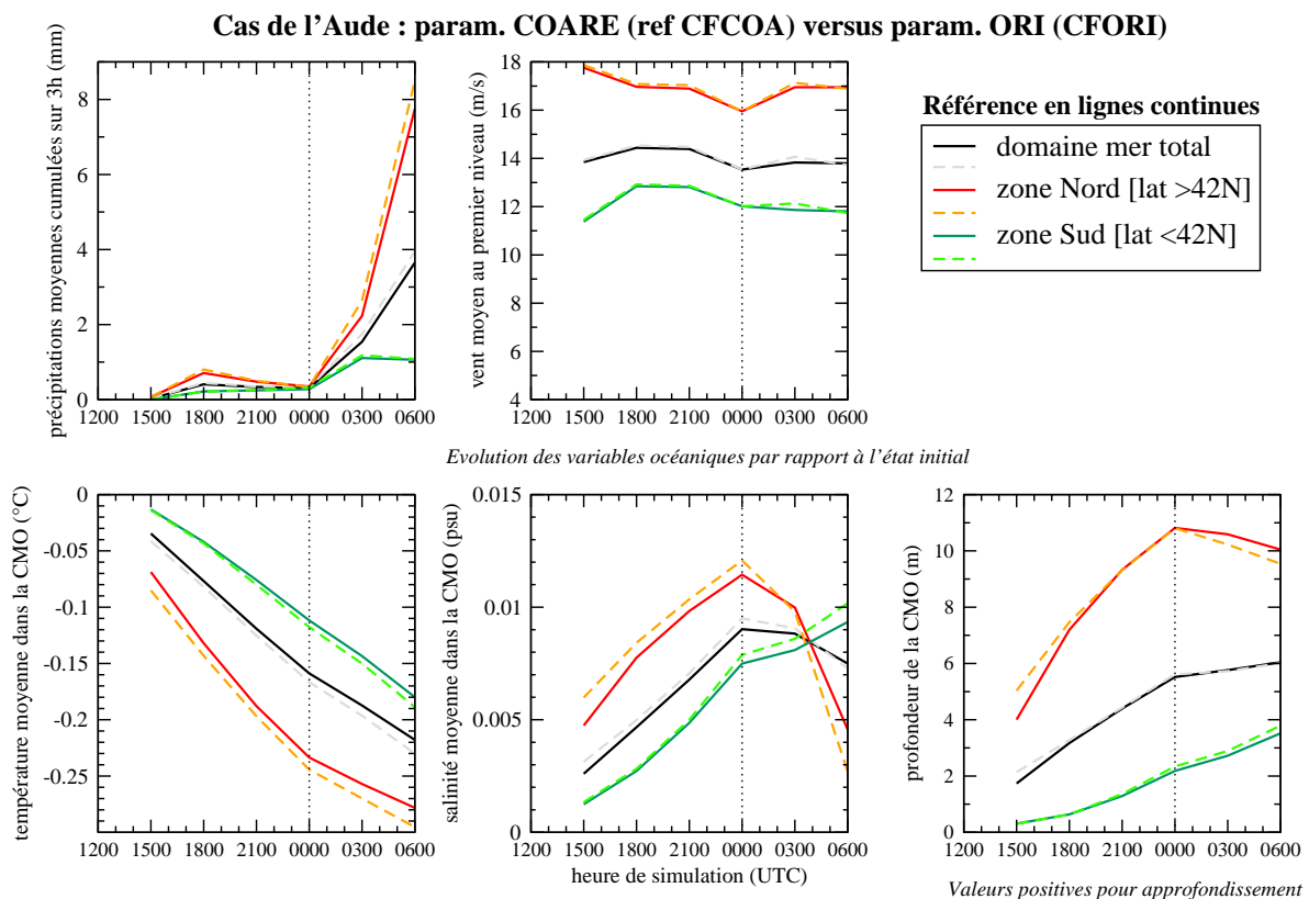
FIG. 9.5 : Cas de l'Aude : Évolution temporelle des paramètres moyens océaniques et du forçage atmosphérique pour différentes zones pour les simulations CFCOA (trait plein) et CFORI (pointillé) : Différence par rapport à l'état initial pour la température moyenne dans la CMO, la salinité moyenne dans la CMO et la profondeur de la CMO (graphes du bas) et cumuls tri-horaires de précipitations et vent à 36 mètres au dessus de la mer (en haut).
