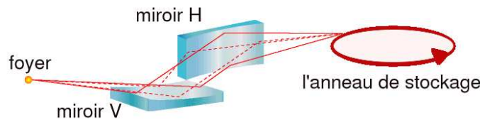
FIGURE 24. Le principe d'une optique Kirkpatrick-Baez.
