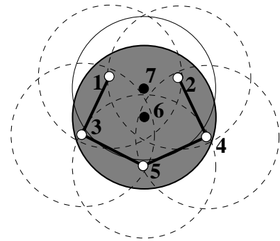
(b) Les cinq premiers nœuds ont déjà décidé. 6 est donc totalement couvert par un ensemble connecté.
