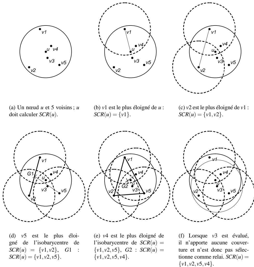
FIG. 3.2 – Exemple de calcul local d'un ensemble SCR avec l'heuristique des isobarycentres.
