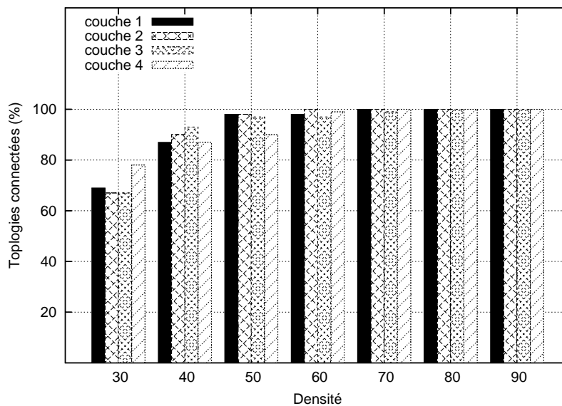
FIG. 4.10 – Connexité de chaque couche (%) avec le protocole SCR-CADS adapté.
