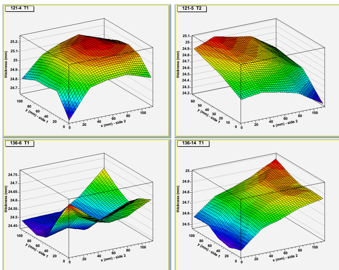
FIG. 2.33 – Profils géométriques typiques des tuiles du RICH d'AMS.
