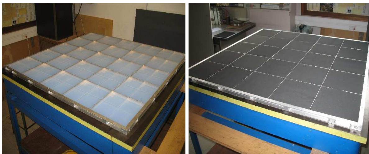
FIG. 3.8 – Plan d'aérogel complet du détecteur CHERCAM, constitué de 200 tuiles de 10 \times 10 \times 105 mm superposées deux à deux. On distingue les tuiles d'aérogel assemblées dans le cadre en aluminium sur la figure de gauche. Sur la figure de droite, les tuiles sont recouvertes de mousse permettant d'absorber les photons provenant du dessus du plan d'aérogel.
