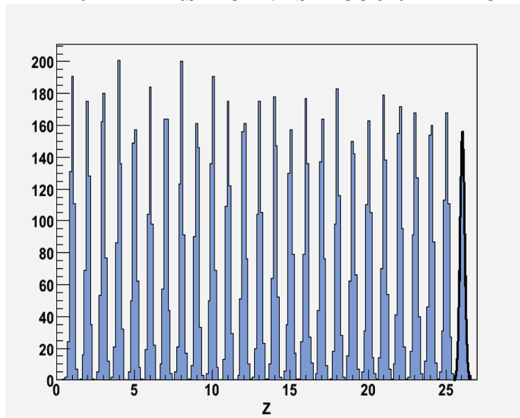
FIG. 4.7 – Reconstruction de la charge pour 11000 événements simulés, uniformément distribués en charge [26].
