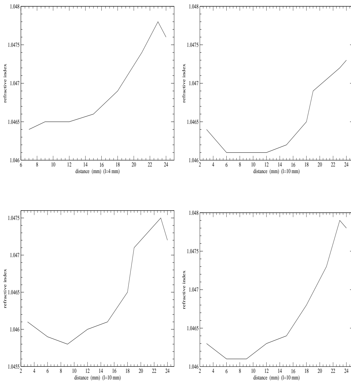
FIG. 2.17 – Variation de l'indice avec la hauteur h du spot d'entrée sur la face latérale de la tuile. (tuile positionnée horizontalement - voir figure 2.19) pour chacun des quatre coins. La distance l est constante pour chacune de ces mesures, et indiquée entre parenthèses.
