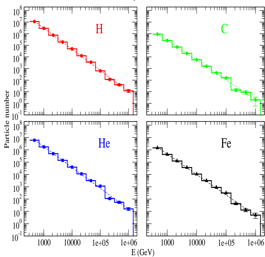
FIG. 1.4 – Spectres en énergie simulés pour les éléments H, He, C et Fe, pour 300 jours de comptage effectif (avec 3 bins par décade en énergie pour une résolution de 50%). Les valeurs de l'indice spectral utilisées sont celles de la référence [7]. Voir texte.
