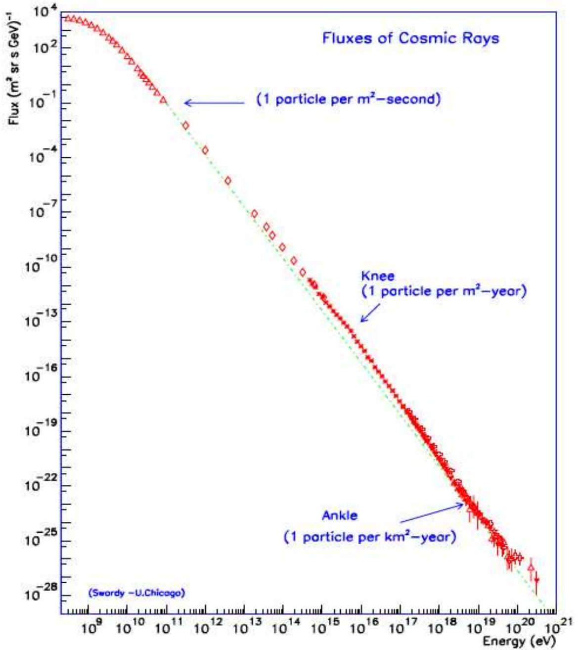
FIG. 1.1 – Spectre d'énergie du rayonnement cosmique (flux différentiel en fonction de l'énergie).
