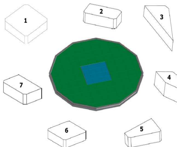
FIG. 2.5 – Le schéma du plan d'aérogel du RICH d'AMS avec les 7 géométries de tuiles qui l'équipent. La partie bleue au centre du plan est constituée de NaF.
