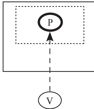
Figure 3.9: La situation visuelle canonique d'après Langacker [2002, p. 16].
