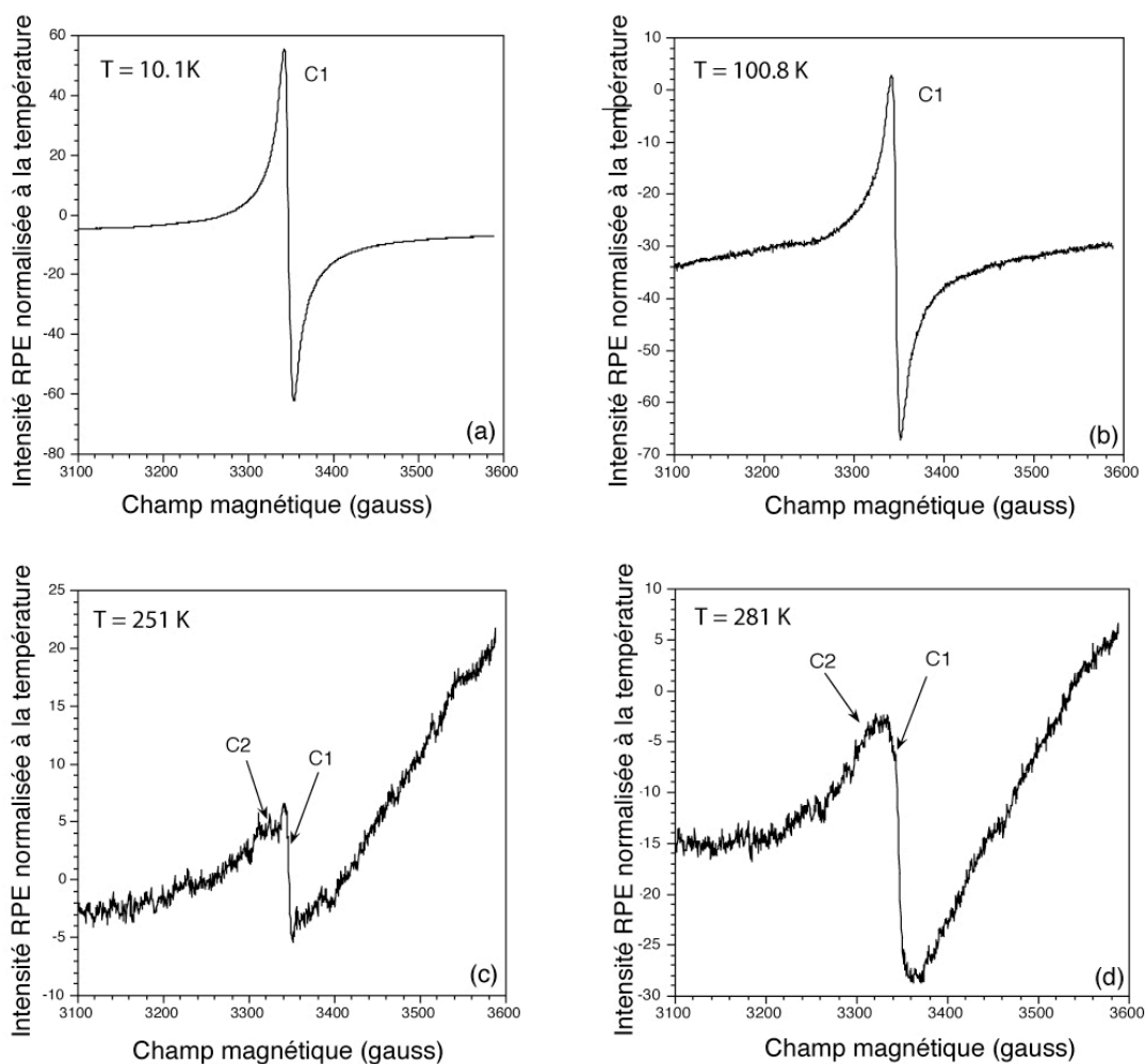
Fig; V-7 : Variation de l'intensité du signal RPE en fonction du champ magnétique appliqué et de la température de l'échantillon NT.
