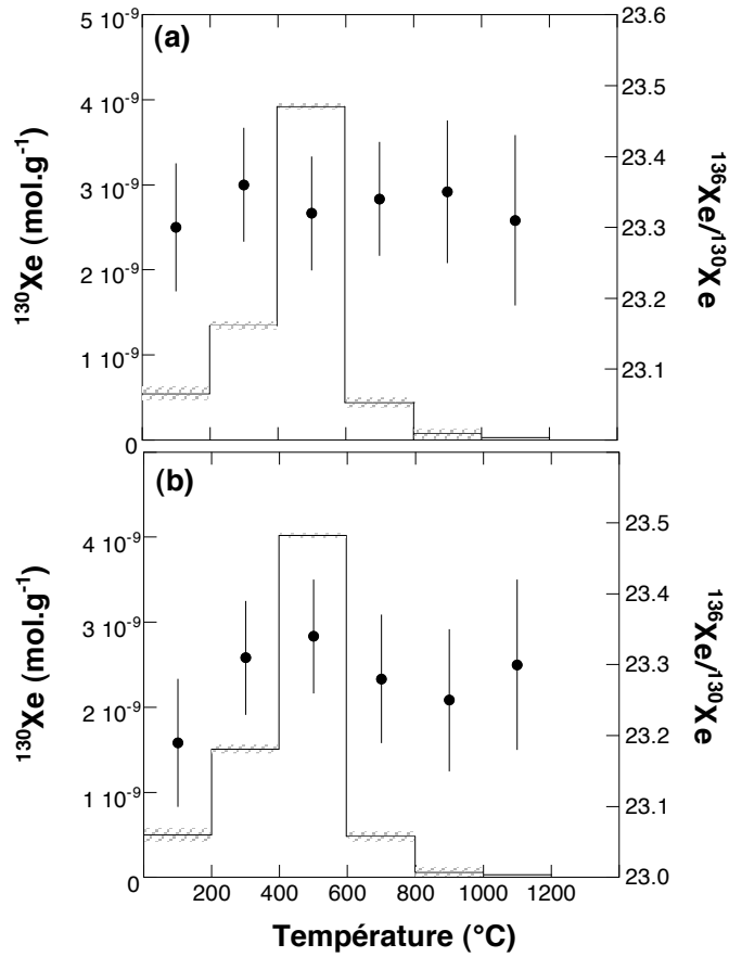
Fig. V-5 : Abondance en ^{130}\text{Xe} et rapport isotopique ^{136}\text{Xe}/^{130}\text{Xe} du xénon piégé dans les échantillons NT obtenus par condensation (rapports isotopiques \times 100 ).
