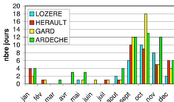
FIGURE 2.6 – Distribution mensuelle du nombre de jours de précipitation > 200 mm de 1958 à 2000 pour les départements de la Lozère, l’Hérault, le Gard et l’Ardèche. Source : Météo-France (2001), extrait du CD-Rom Pluies extrêmes sur le Sud de la France.
