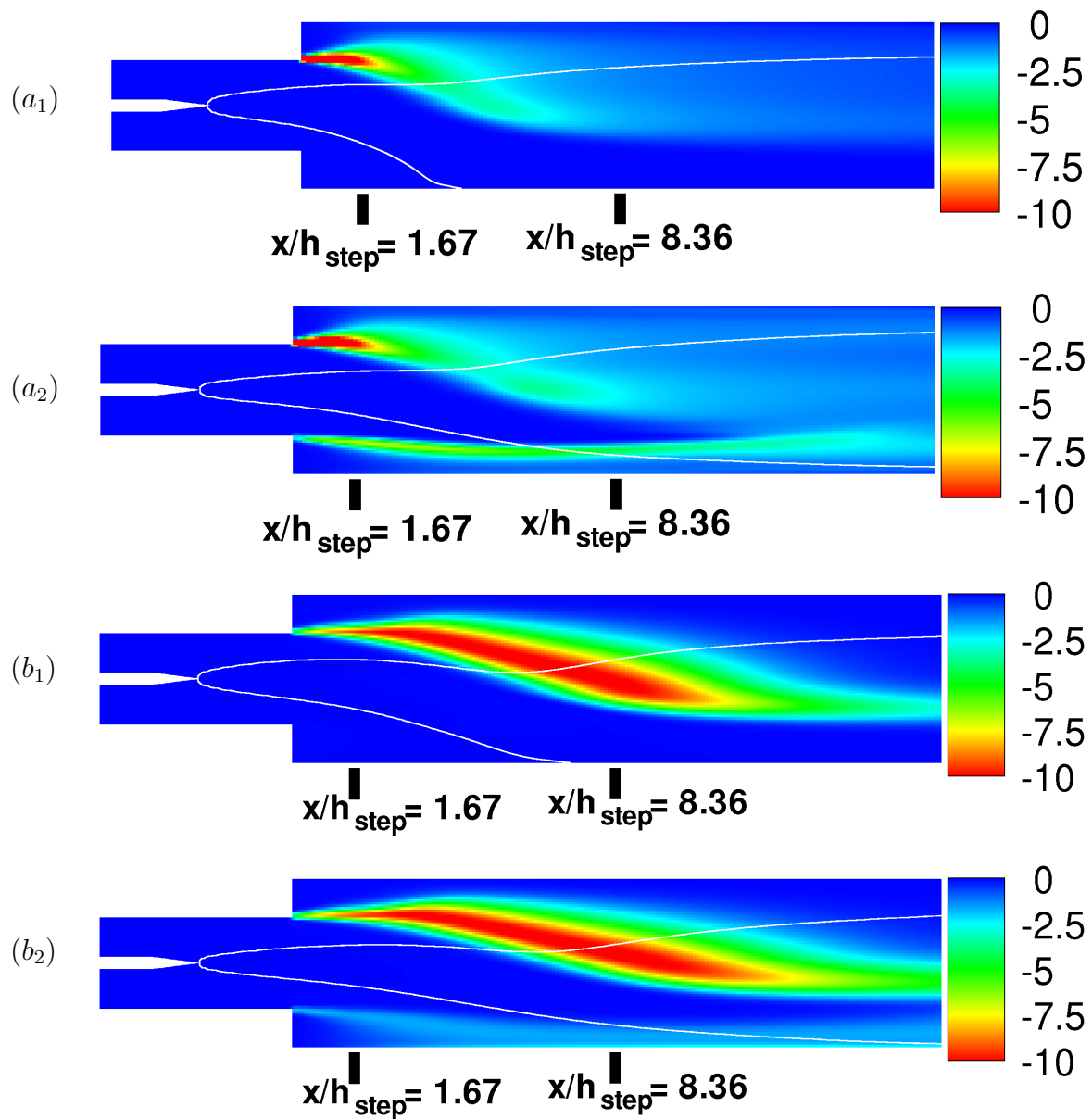
FIG. 8.15 – Taux de réaction moyen ( s^{-1} ). Iso-ligne \widetilde{\xi'^2}=1.10^{-8} (ligne blanche). a_1 : \Phi(1)=0,3 , \Phi(2)=0,9 et relaxations linéaires, a_2 : \Phi(1)=0,7 , \Phi(2)=0,9 et relaxations linéaires, b_1 : \Phi(1)=0,3 , \Phi(2)=0,9 et fermetures généralisées, b_2 : \Phi(1)=0,7 , \Phi(2)=0,9 et fermetures généralisées.
