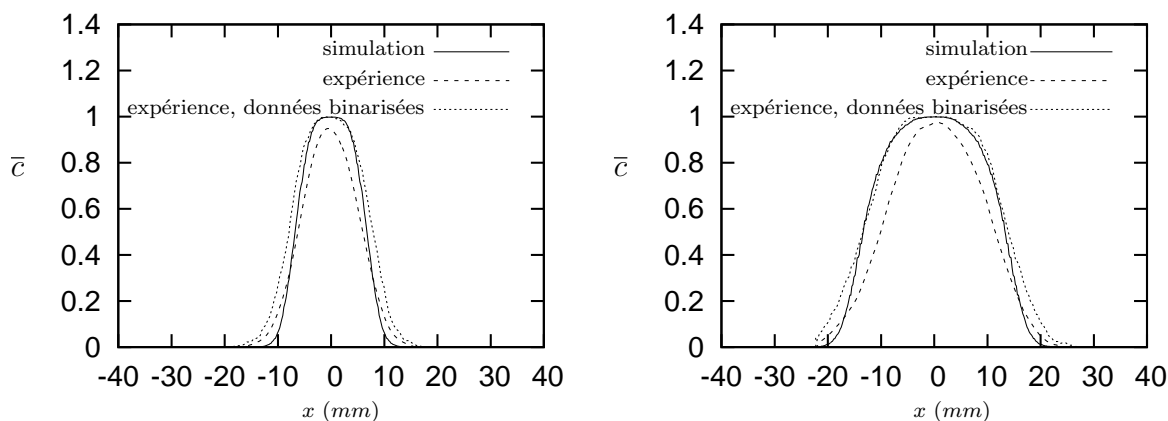
FIG. 9.13 – Variable d'avancement moyenne à z=42.5 mm (gauche) et 70 mm (droite) pour des conditions d'un mélange homogène, cas HE06.
