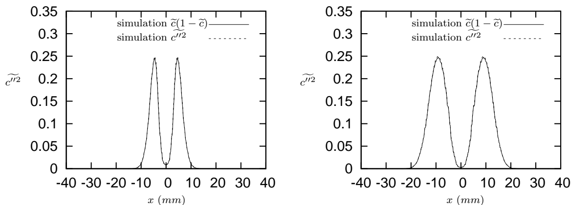
FIG. 9.12 – Variance de la variable d'avancement à z=42.5 mm (gauche) et 70 mm (droite) pour des conditions d'un mélange homogène, cas HE06.
