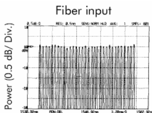
Figure 26. Signal à l'entrée de la fibre (d'après [10])
