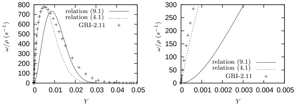
FIG. 9.10 – \omega / \rho = f(Y) pour \Phi=1 dans le cas d'une réaction globale en utilisant l'expression (4.1), dans le cas d'une réaction globale en utilisant l'expression (9.1) et dans le cas du schéma cinétique détaillé GRI-2.11, la figure de droite est un agrandissement de la figure de gauche pour de faibles valeurs de Y .
