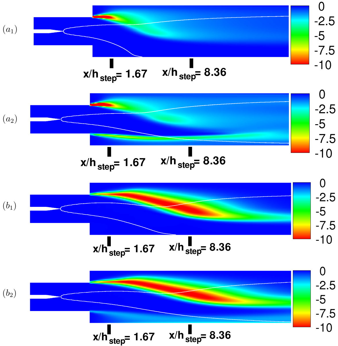
FIG. 8.15 – Taux de réaction moyen ( s^{-1} ). Iso-ligne \widetilde{\xi''^2} = 1.10^{-8} (ligne blanche). a_1 : \Phi(1)=0, 3 , \Phi(2)=0, 9 et relaxations linéaires, a_2 : \Phi(1)=0, 7 , \Phi(2)=0, 9 et relaxations linéaires, b_1 : \Phi(1)=0, 3 , \Phi(2)=0, 9 et fermetures généralisées, b_2 : \Phi(1)=0, 7 , \Phi(2)=0, 9 et fermetures généralisées.
