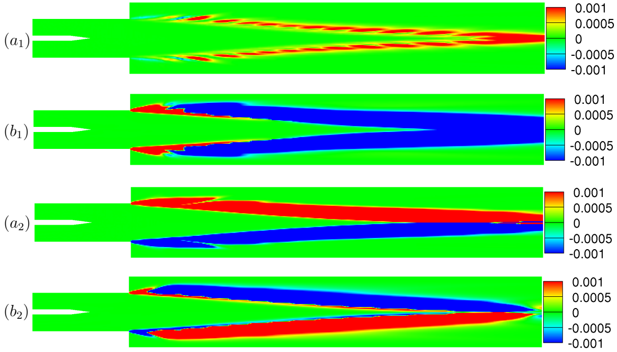
FIG. 10.5 – Composante longitudinale des flux turbulents \widetilde{u''Y''} (2 figures du haut) et composante transversale des flux turbulents \widetilde{v''Y''} (2 figures du bas), en m.s^{-1} obtenues pour \Phi(1)=\Phi(2)=0,8 en utilisant le modèle LW-P du second ordre complet, (a_1) : D_T \partial \widetilde{Y} / \partial x , (b_1) : \widetilde{u''Y''} , (a_2) : D_T \partial \widetilde{Y} / \partial y , (b_2) : \widetilde{v''Y''}
