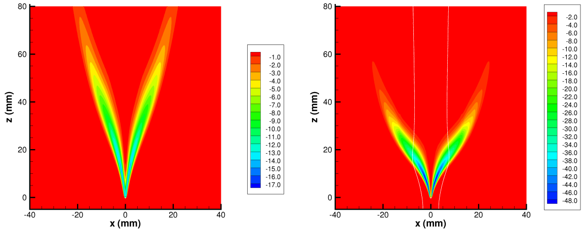
FIG. 9.22 – Taux de réaction chimique moyen \bar{\omega} / \bar{\rho} \text{ (s}^{-1}\text{)} pour des conditions d'un mélange stratifiés SB08-0 et SB12-0. La ligne stœchiométrique \tilde{\xi} = \xi_{st} est visualisée.
