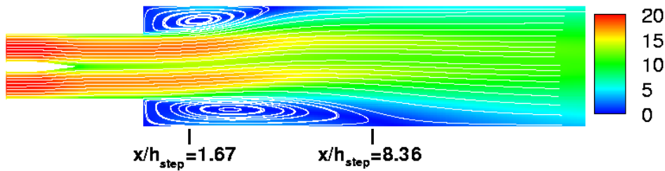
FIG. 8.8 – Écoulement non-réactif : champ de vitesse moyenne ( m/s ) et ligne de courant
