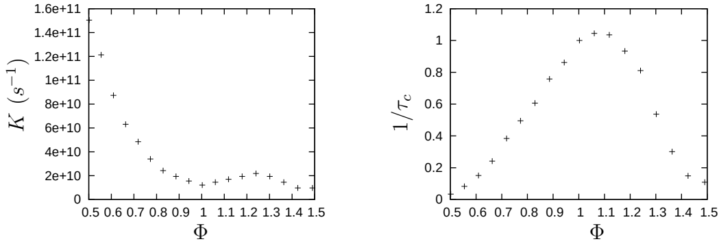
FIG. 9.8 – Coefficient pré-exponentiel K (gauche) et l'inverse du temps chimique ( 1/\tau_c = K \exp(T_a/T_{ad}) ) du mélange méthane-air adimensionné par la valeur à la stœchiométrie (droite) en fonction de la richesse
