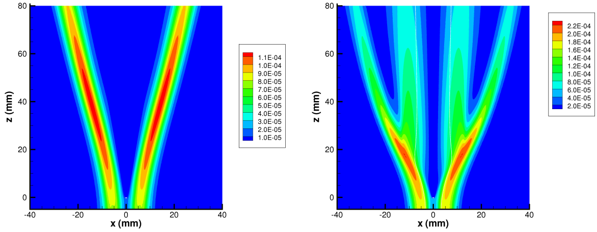
FIG. 9.23 – Champ de covariance \widetilde{\xi''Y''} pour des conditions d'un mélange stratifié SB08-0 et SB12-0. La ligne stœchiométrique \tilde{\xi} = \xi_{st} est visualisée.
