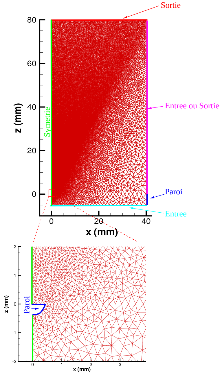
FIG. 9.4 – Maillage non structuré utilisé pour les simulations numériques
