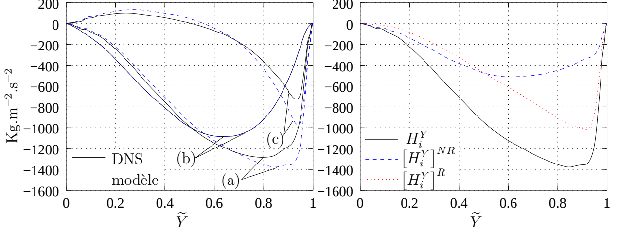
FIG. 7.2 – Validation du modèle pour le terme de corrélation scalaire-pression par comparaison avec la base de données DNS : (a) -\overline{Y''\partial p/\partial x} = H_i^Y , (b) -\overline{Y''\partial \bar{p}/\partial x} , (c) -\overline{Y''\partial p'/\partial x}
