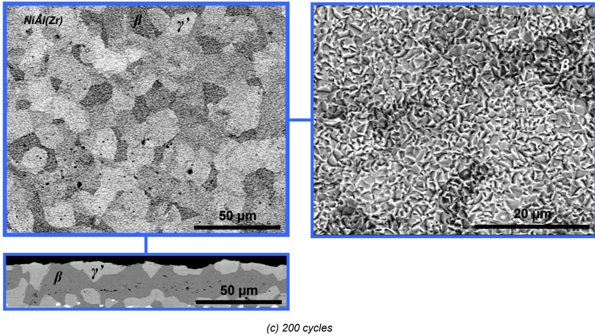
Figure 3.9 - Faciès de rupture (côté métal) des éprouvettes représentatives du système AM1/NiAl(Zr)/YPSZ après oxydation cyclique à 1100°C et coupe de la couche de liaison associée (a) 50 cycles (b) 100 cycles (c) 200 cycles (+ détail du faciès de rupture)
