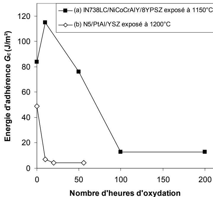
Figure 3.1 - Evolution de l'énergie d'adhérence de deux systèmes barrière thermique en oxydation isotherme pour \Psi^* = 90^\circ
