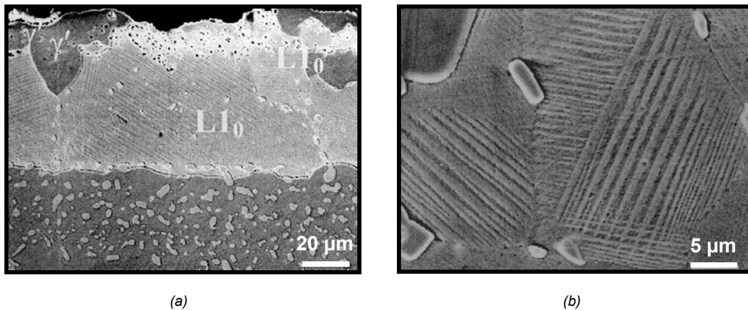
Figure 1.14 - Phase martensitique lamellaire (structure cristallographique L1_0 ) au sein d'une couche de liaison (Ni,Pt)Al en surface du superalliage CMSX-4 après 1500 h à 1100°C [96] (a) Vue d'ensemble (b) Vue rapprochée
