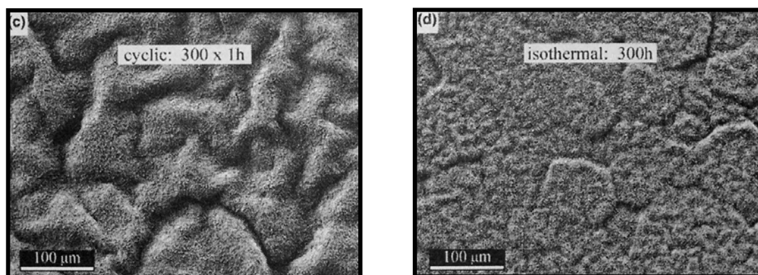
Figure 1.15 - Couche d'alumine formée en surface du système superalliage/(Ni,Pt)Al [99]
