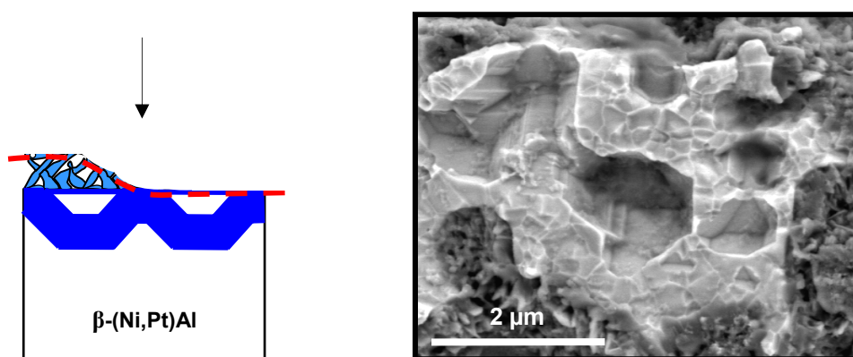
Figure X – Détail du faciès de rupture du système AM1/(Ni,Pt)Al/YPSZ brut d'élaboration dont la couche de liaison n'a pas été sablée - Empreintes d'alumine \alpha en surface de la couche de liaison et cavités
