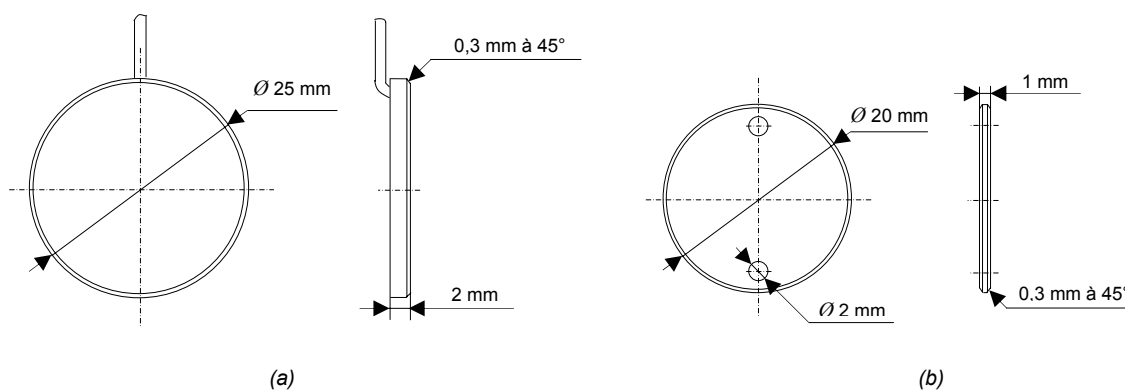
Figure 1.22 - Géométrie des échantillons dédiés aux essais d'oxydation cyclique
