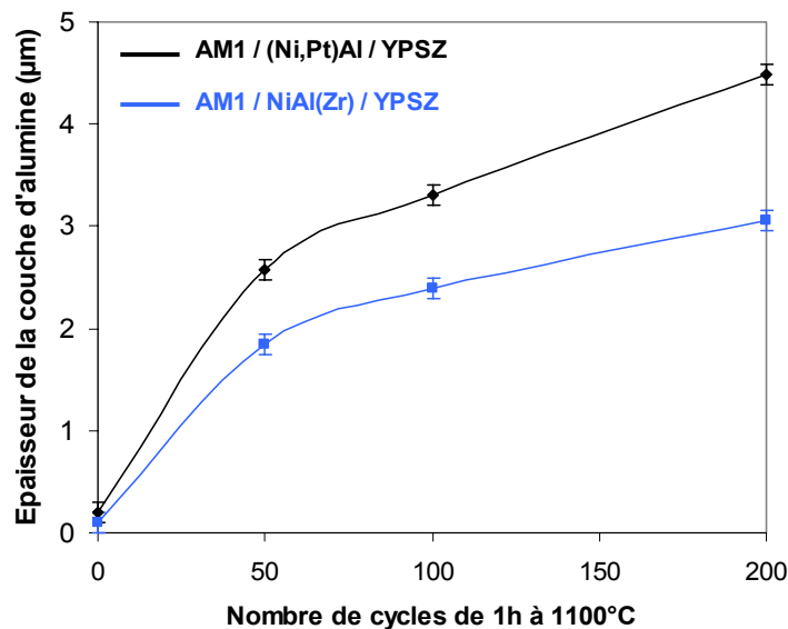
Figure 1.58 - Evolution de l'épaisseur moyenne de la couche d'alumine des systèmes AM1/(Ni,Pt)Al/YPSZ et AM1/NiAl(Zr)/YPSZ en oxydation cyclique à 1100°C
