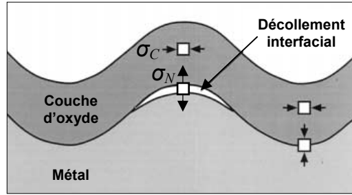
Figure 1.16 - Endommagement consécutif à l'augmentation progressive de la rugosité de l'interface métal/oxyde en oxydation cyclique [61]
