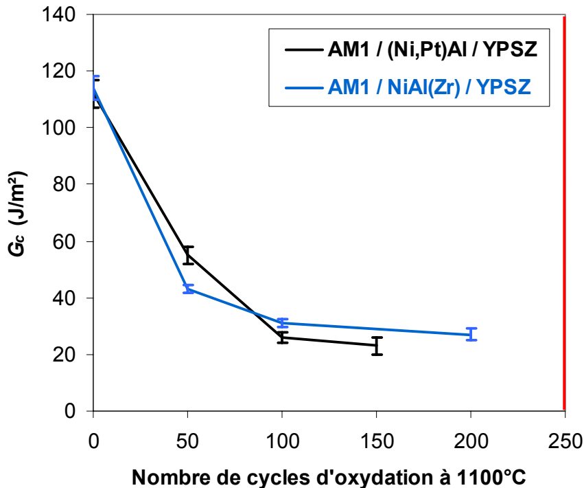
Figure 3.2 - Evolution de l'adhérence des deux systèmes barrière thermique G_c ( \Psi^* = 40^\circ ) en oxydation cyclique à 1100°C
