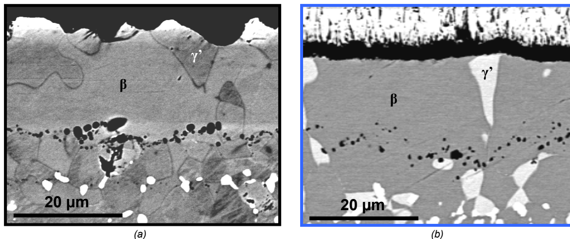
Figure 1.50 - Couche de liaison biphasée après 50 cycles d'oxydation de 1 h à 1100°C (a) AM1/(Ni,Pt)Al/YPSZ (b) AM1/NiAl(Zr)/YPSZ
