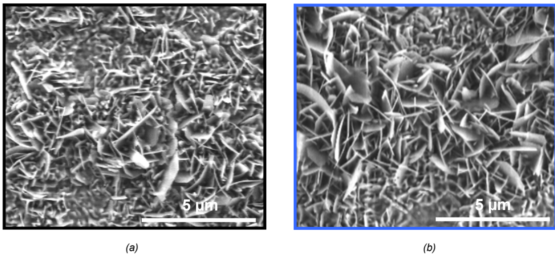
Figure 1.36 - Alumine \theta formée en surface des aluminures de nickel après 5 cycles de 1 h à 1100°C (a) AM1/(Ni,Pt)Al (b) AM1/NiAl(Zr)
