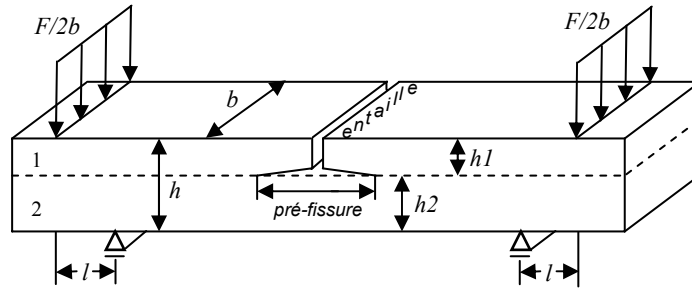
Figure 2.4 - Essai d'adhérence
