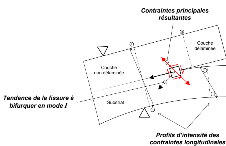
Figure 2.5 - Analyse qualitative de l'état de contraintes en pointe de fissure montrant la tendance de la fissure à bifurquer lors de l'essai de flexion 4 points
