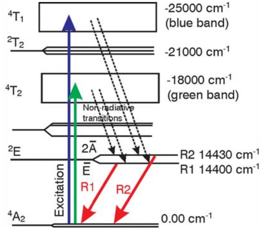
Figure 1.32 - Niveau d'énergie dans le domaine visible du chrome dans l'alumine [161]
