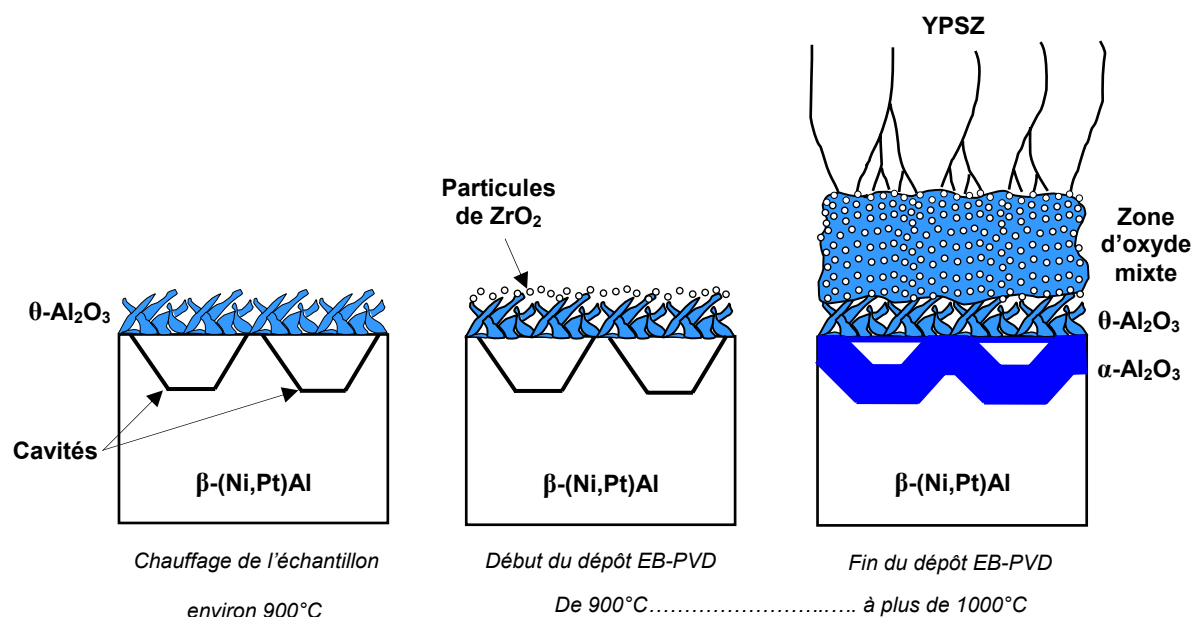
Figure VI – Oxydation des échantillons non sablés au cours de l'élaboration du dépôt EB-PVD de zircone (en bleu clair : \theta\text{-Al}_2\text{O}_3 ; en bleu foncé \alpha\text{-Al}_2\text{O}_3 )
