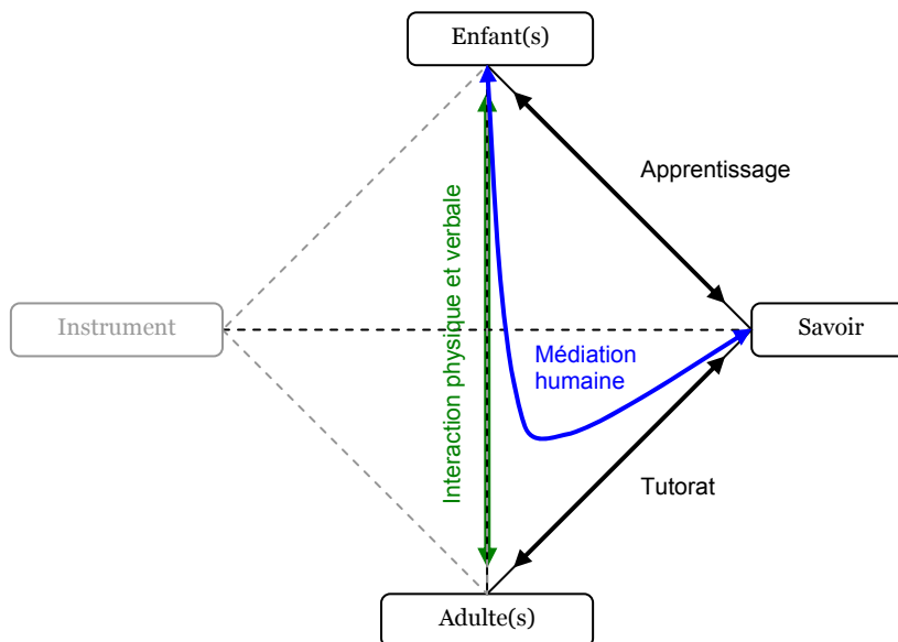
Figure 3-8. Carré médiateur tronqué (exemple 3)
