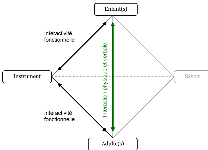
Figure 3-7. Carré médiateur tronqué (exemple 2)
