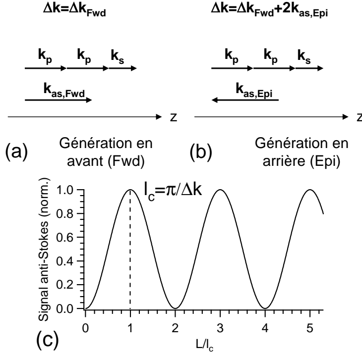
FIG. 2.6 – Désaccord de phase lors de la génération du signal anti-Stokes en configuration Fwd-CARS (a) et Epi-CARS (b). (c) Influence de la longueur L du milieu sur la génération du signal anti-Stokes et définition de la longueur de cohérence l_c .
