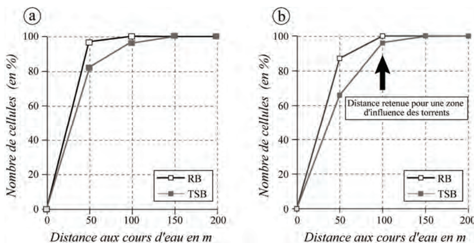
a. Fréquences cumulées avec VM2. b. Fréquences cumulées avec VM3. TSB = Mouvement translationnel superficiel de berge ; RB = Mouvement rotationnel de berge.
