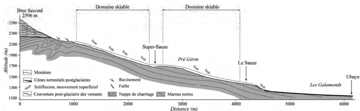
Fig. 3.16. Coupe géologique simplifiée du secteur d'Enchastrayes.
