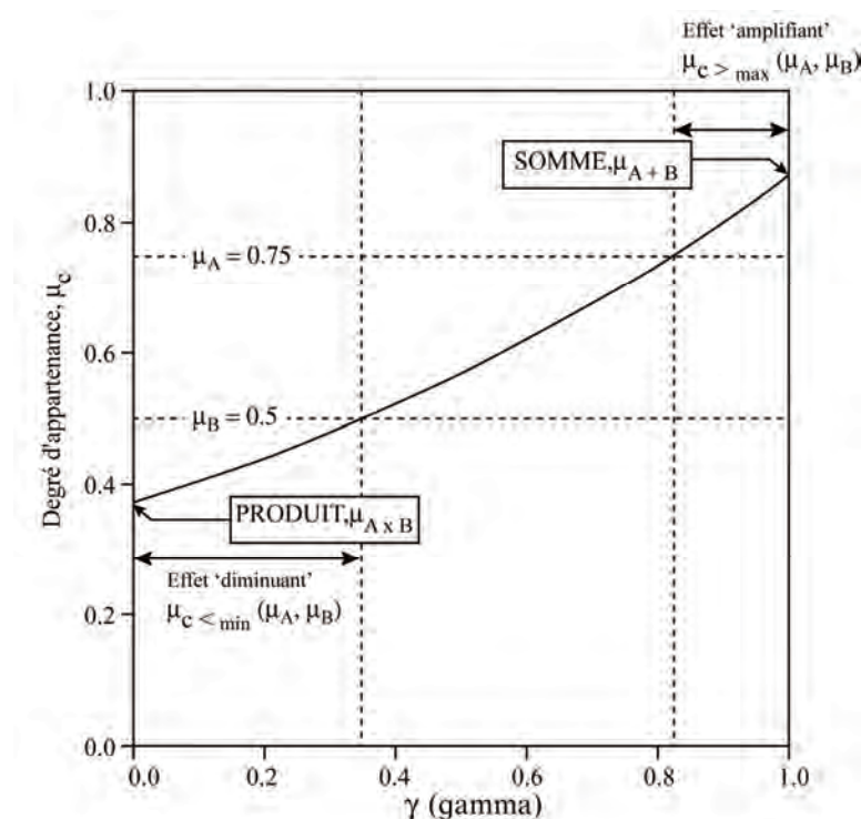
Fig. A6.2. Graphique représentant l'influence du coefficient \gamma pour l'opérateur GAMMA (d'après Bonham-Carter, 1994).
