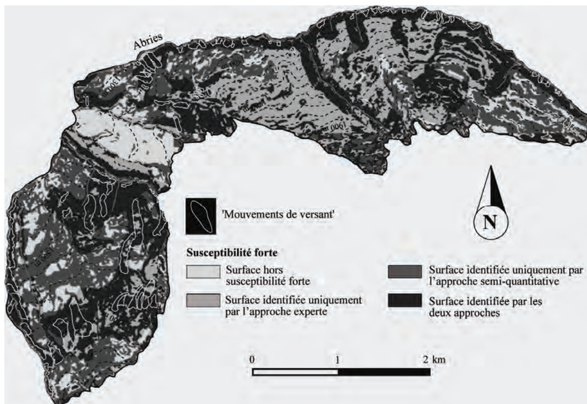
Fig. 6.12. Carte des différences entre les surfaces reconnues en susceptibilité forte pour la carte 'expert' et la carte semi-quantitative unifiée.
