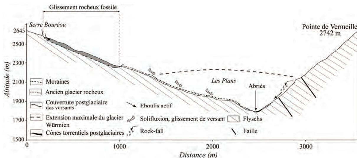
Fig. 3.5. Coupe géologique simplifiée de la vallée de l'Abriès (localisation de la coupe sur la Fig. 3.6).
