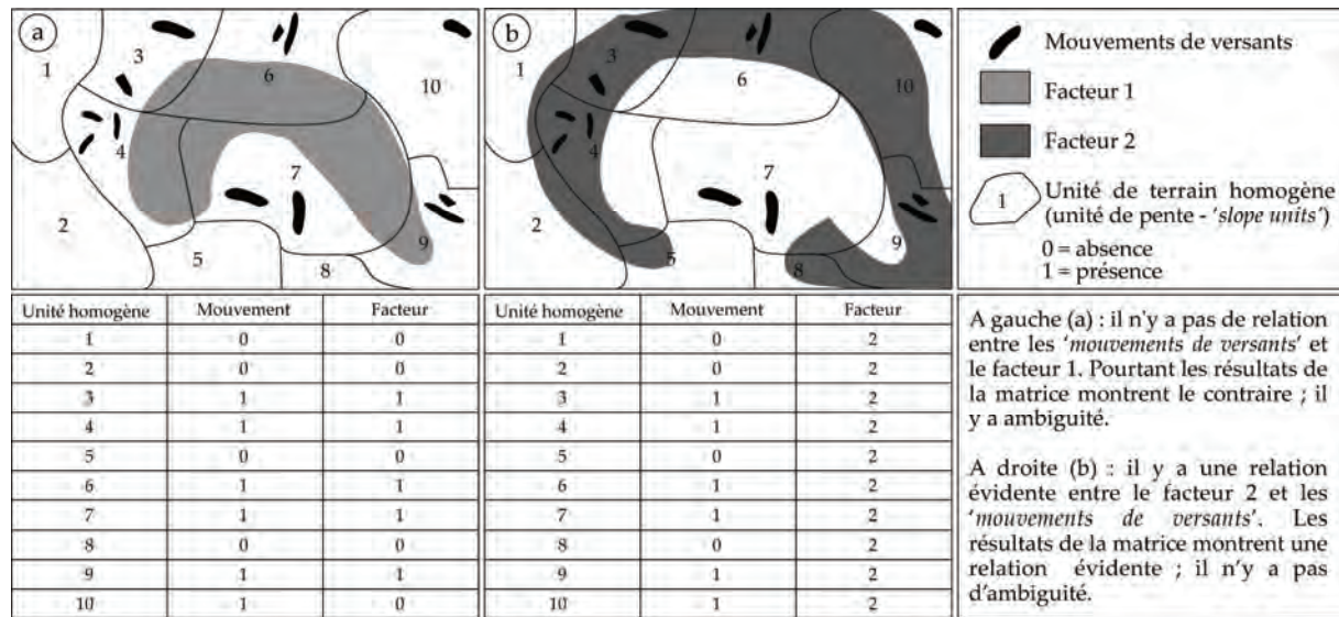
Fig. 1.7. Problèmes relatifs à l'échantillonnage des facteurs avec des unités homogènes par polygones pour une analyse statistique (adapté de van Westen, 1993).
